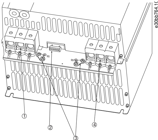
Рисунок 7: Размер корпуса Н8, IP20, 380–480 В, 90 кВт (125 л. с.), IP20, 200–240 В, 37–45 кВт (50–60 л. с.), IP20, 525–600 В, 75–90 кВт (100–125 л. с.)
