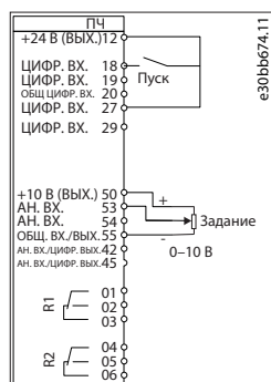
Рисунок 27: Проводка преобразователя частоты
