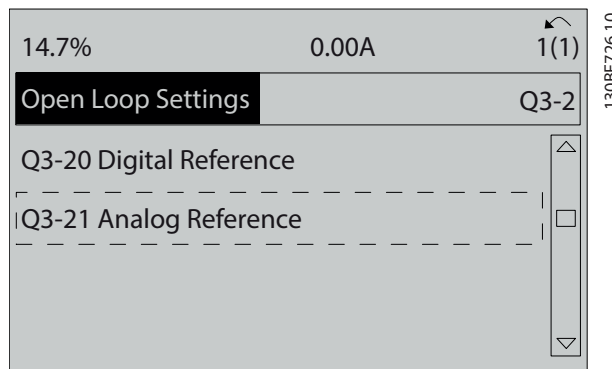
圖 6.5 Q3-21 類比設定值
