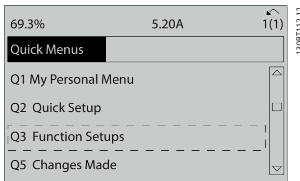
圖 6.3 Q3 功能設定表單 (Function Setups)
