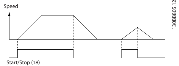
圖 7.2 啟動/停機指令 (含安全轉矩關閉功能)
