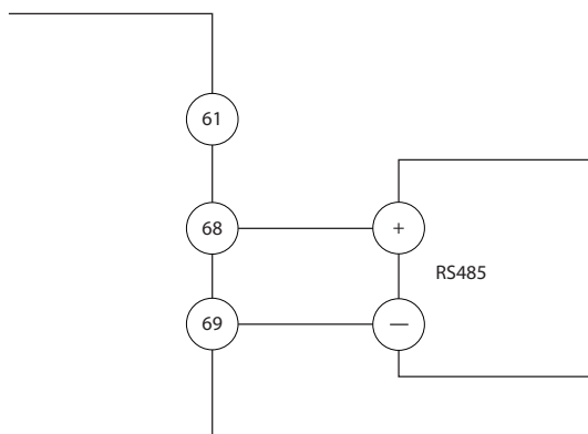
圖 5.22 串列通訊配線圖
