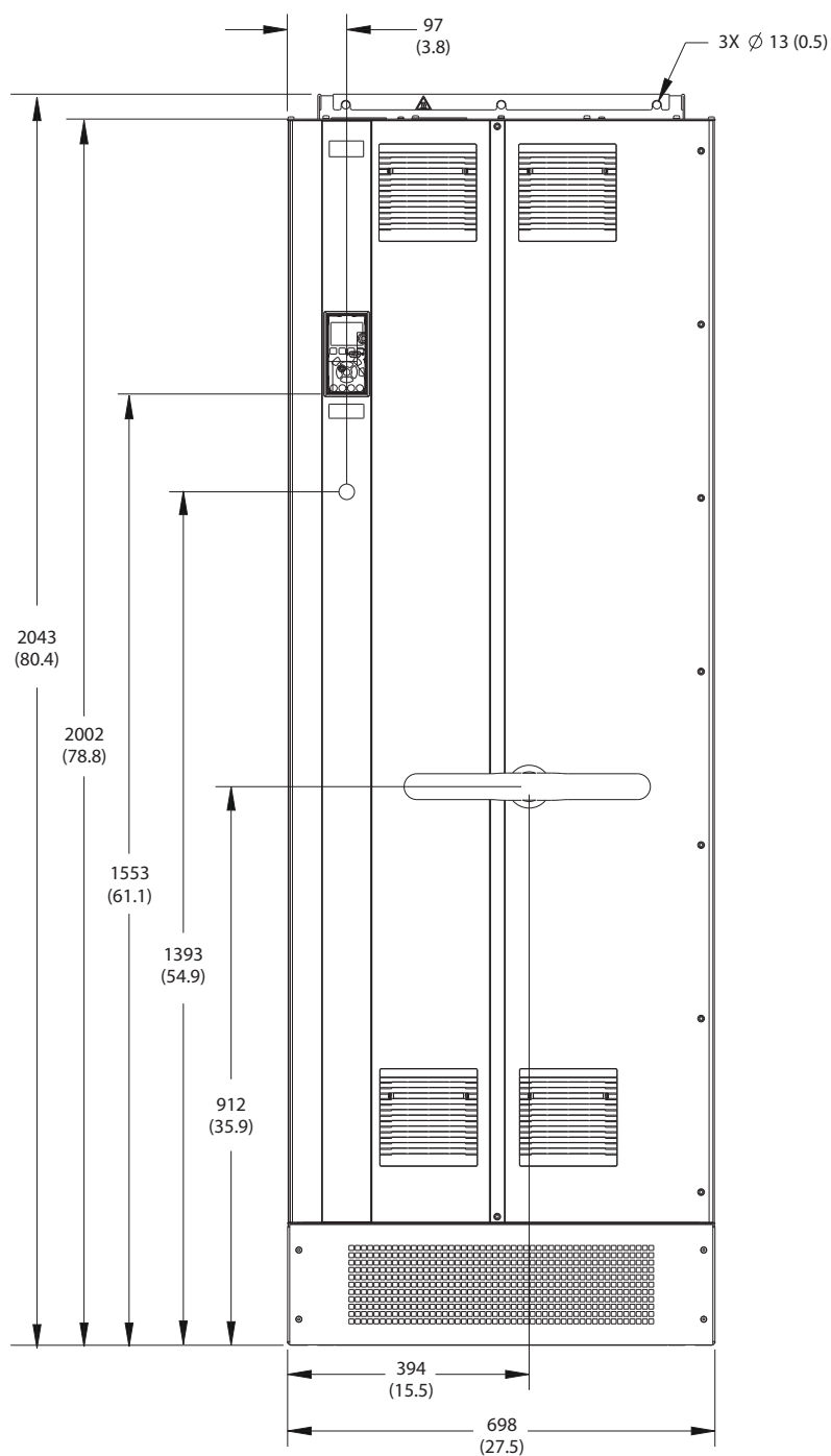
圖 9.6 E2h 的正面圖
