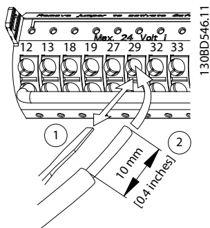
圖 5.21 連接軟型控制電線
