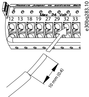
圖 5.20 連接實心的控制電線
