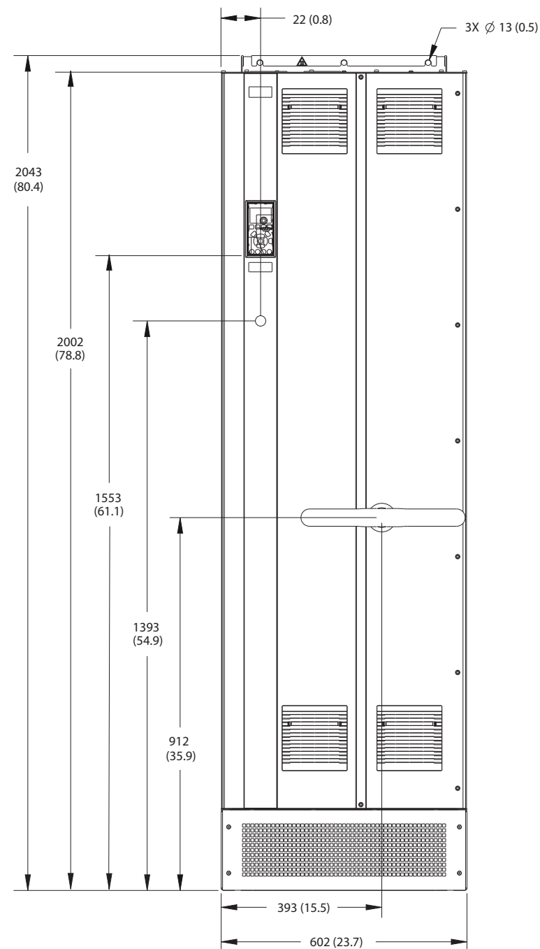
圖 9.2 E1h 的正面圖
