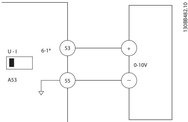
圖 6.12 提供 0-10 V 控制信號之外部裝置的線路範例
