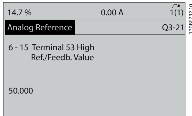
圖 6.11 參數 6-15 端子 53 最高設定值/回授值
