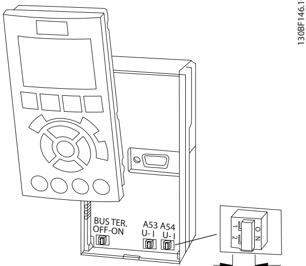
圖 5.23 端子 53 和 54 開關的位置
