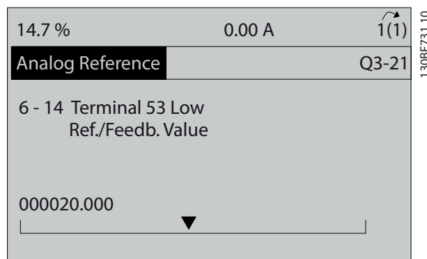
圖 6.10 參數 6-14 端子 53 最低設定值/回授值
