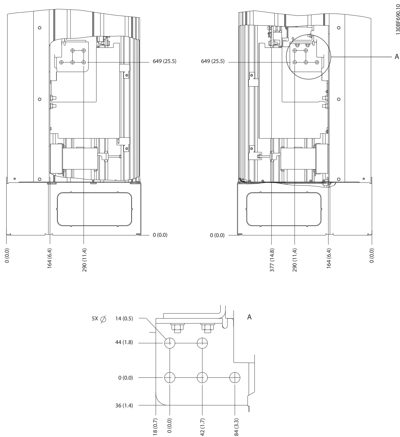
圖 5.9 E2h 端子尺寸 (側面視圖)
