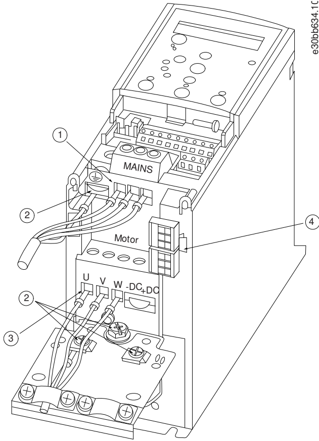
Çizim 4: Muhafaza Boyutları H1–H5, IP20, 200–240 V, 0,25–11 kW (0,33–15 hp), IP20, 380–480 V, 0,37–22 kW (0,5–30 hp)
