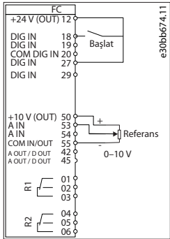
Çizim 27: Sürücü Kablo Tesisatı
