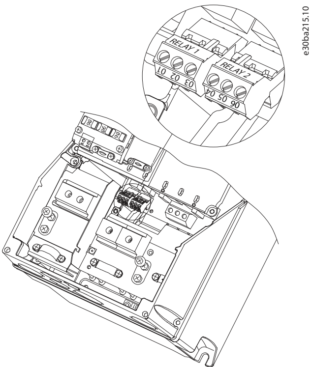
圖解 20: 外殼規格為 I6, IP54, 380–480 V, 22–37 kW (30–50 hp) 的繼電器
