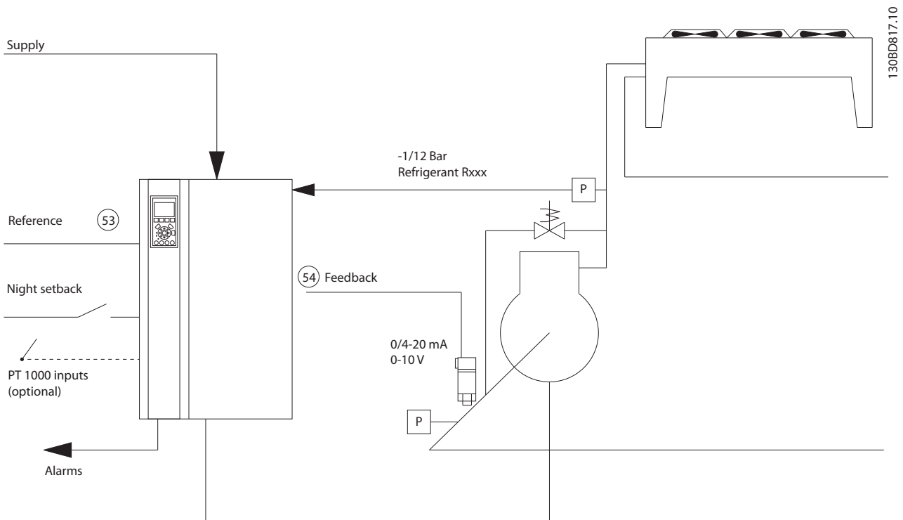
그림 6.1 "내부 제어부가 있는 압축기"의 기본 도면
