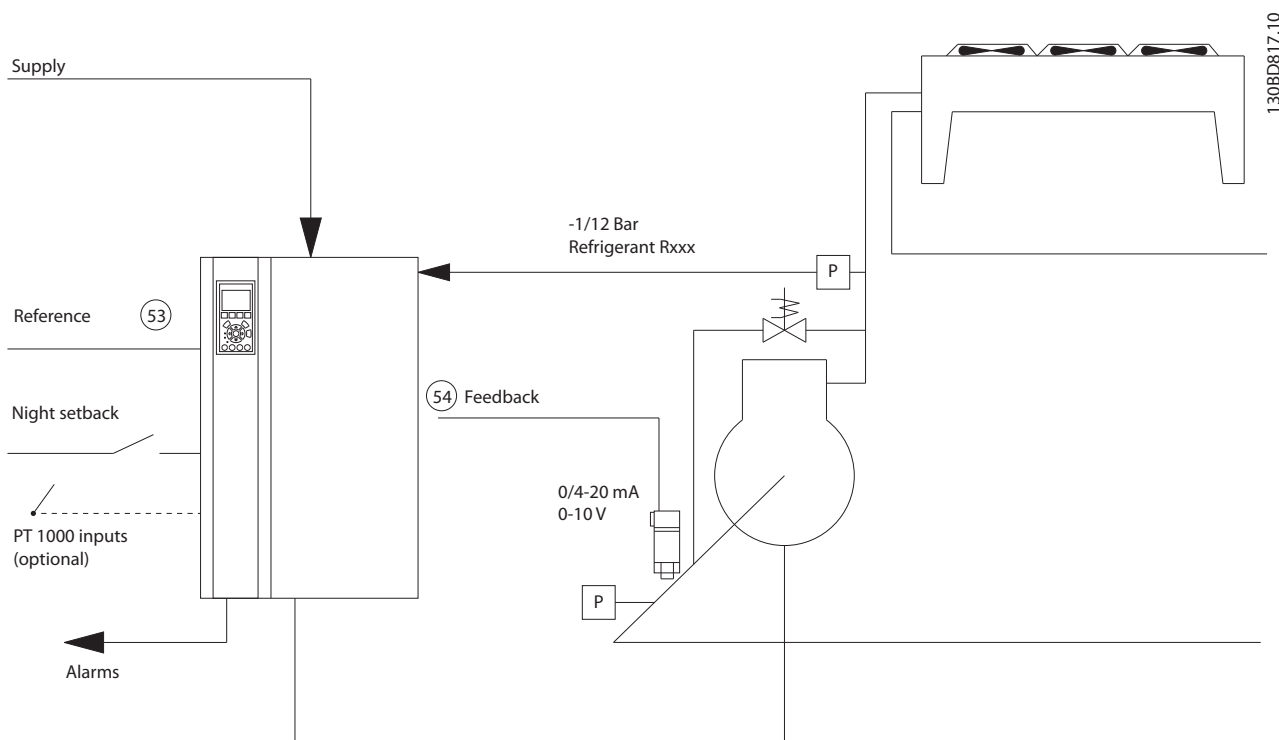
Afbeelding 6.1 Standaardtekening van 'compressor met interne regeling'
