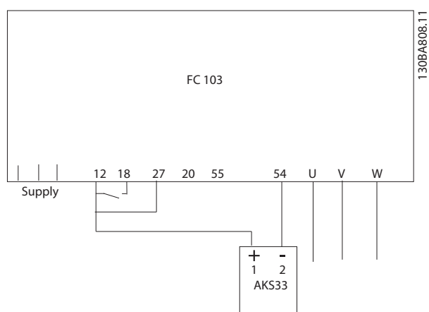
Afbeelding 6.5 De FC 103 en AKS 33 aansluiten voor een toepassing met terugkoppeling
