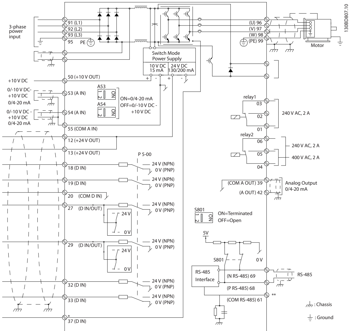
Afbeelding 4.1 Eenvoudig bedradingsschema
