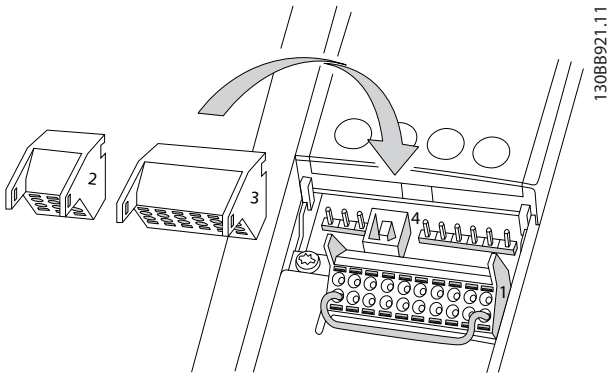
Afbeelding 4.7 Stuurklemposities
