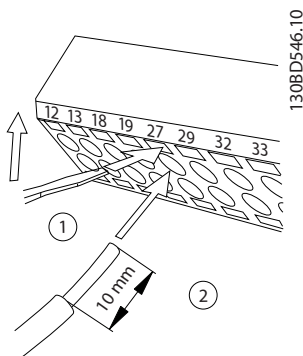
Ilustracija 4.9 Povezava krmilnih žic
