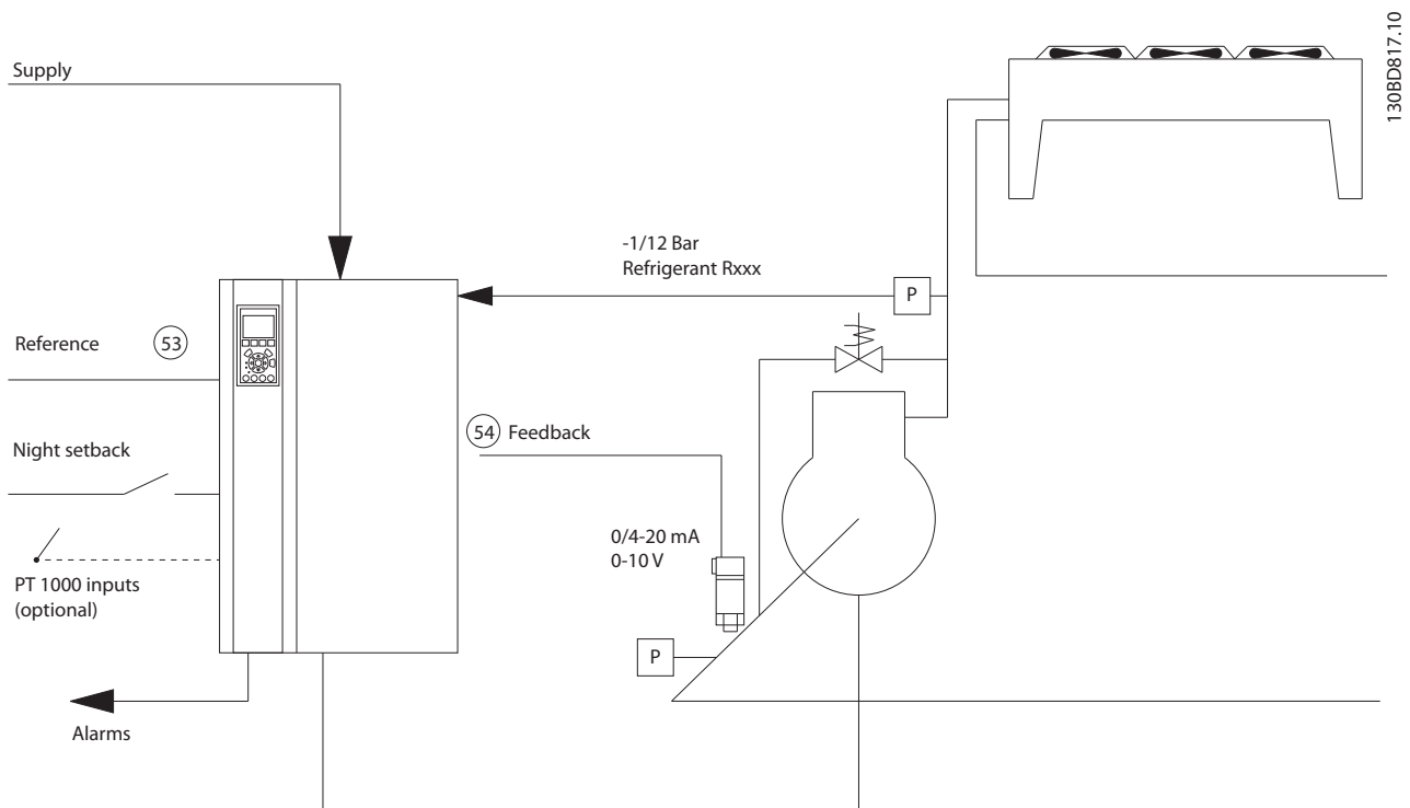
Slika 6.1 Standardni crtež „Kompresor sa internom kontrolom“
