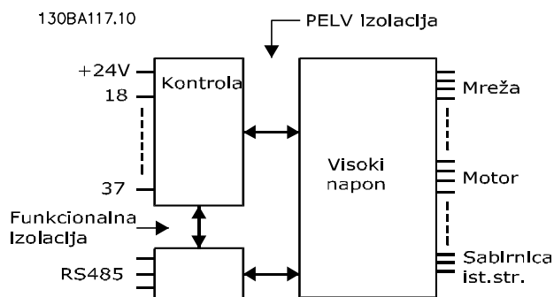
Slika 8.1 PELV izolacija analognih ulaza
