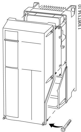
Slika 4.4 Pristup ožičenju za kućišta IP55 i IP66
