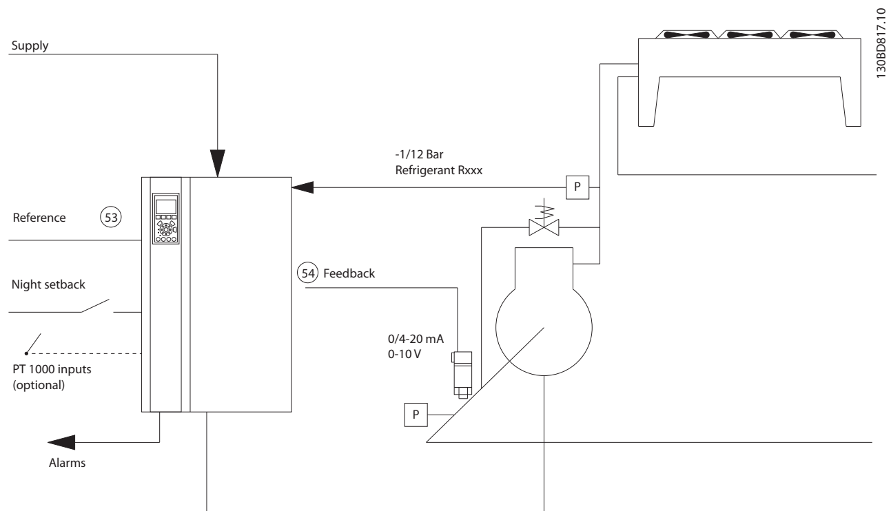
圖 6.1 「具內部控制的壓縮機」標準圖
