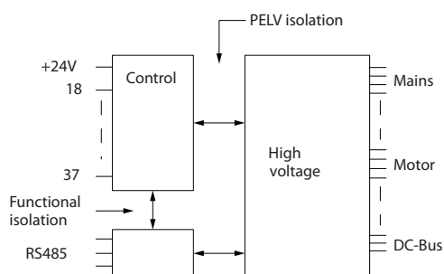
圖 8.1 類比輸入的 PELV 絕緣
