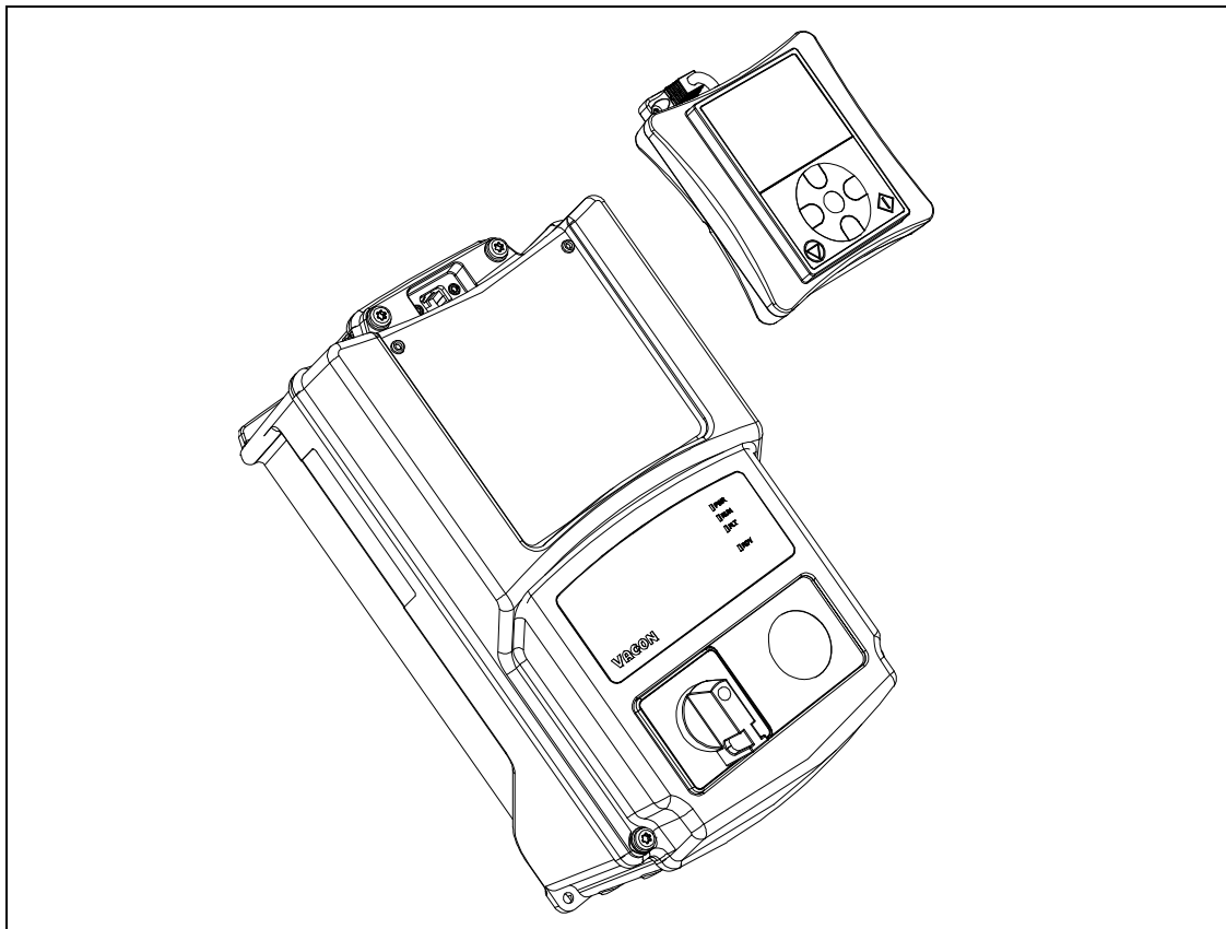
Figura 48. Montaje del panel.
