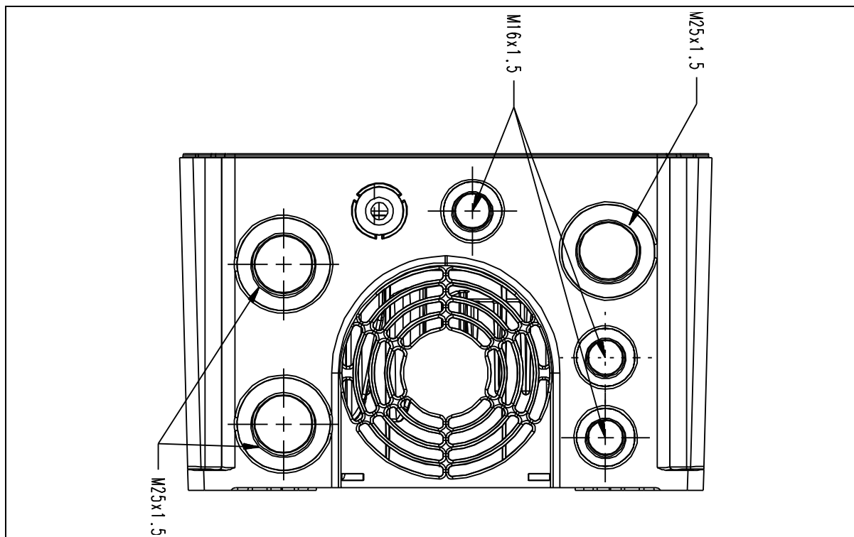
Figura 22. Entradas de cable, MU3.
