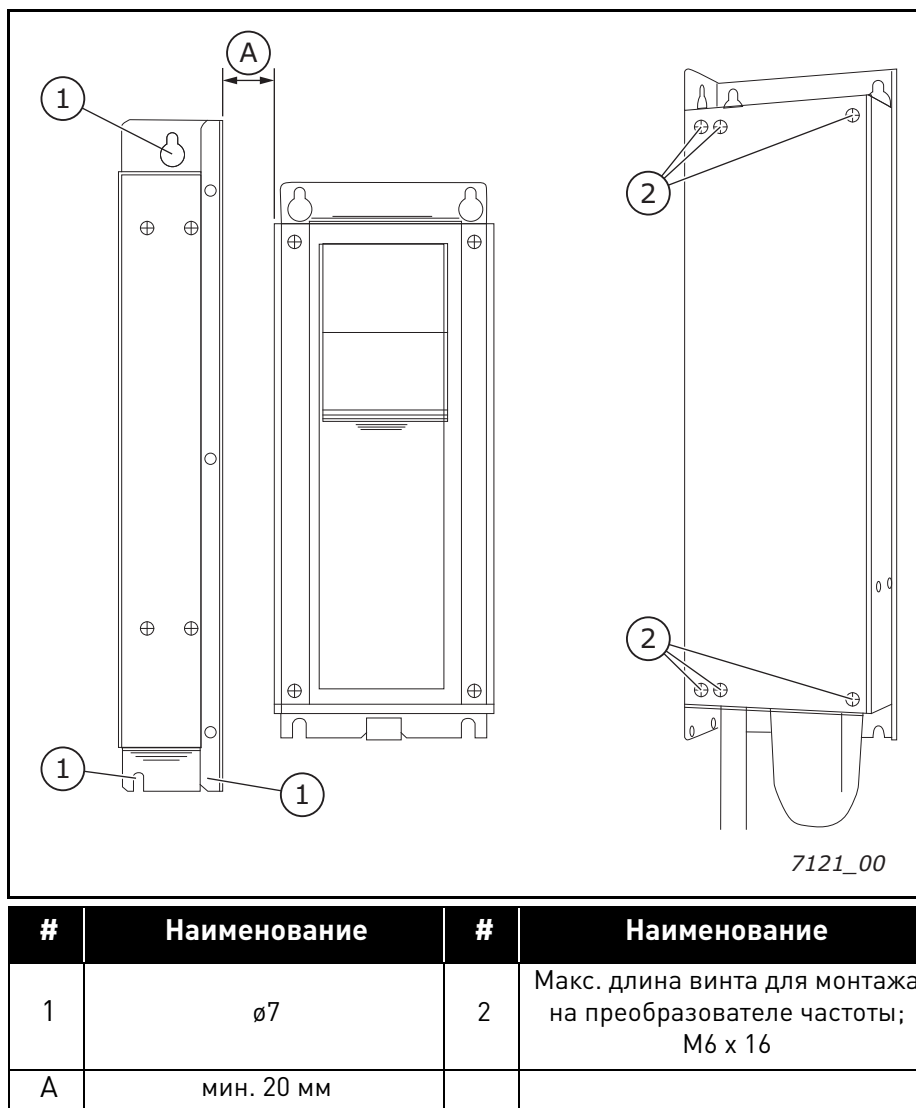
Рис. 4. Монтаж фильтра ВЧ-помех сбоку
