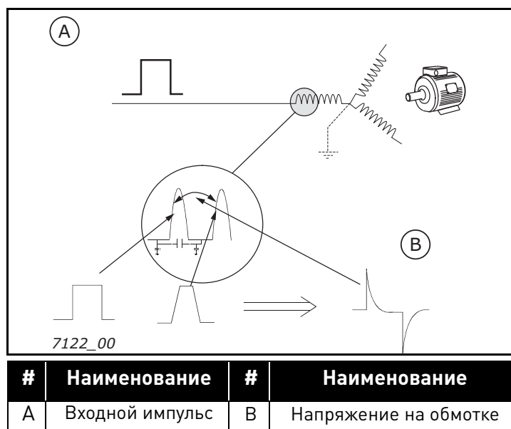
Рис. 5. Изменение формы импульса напряжения в обмотке
