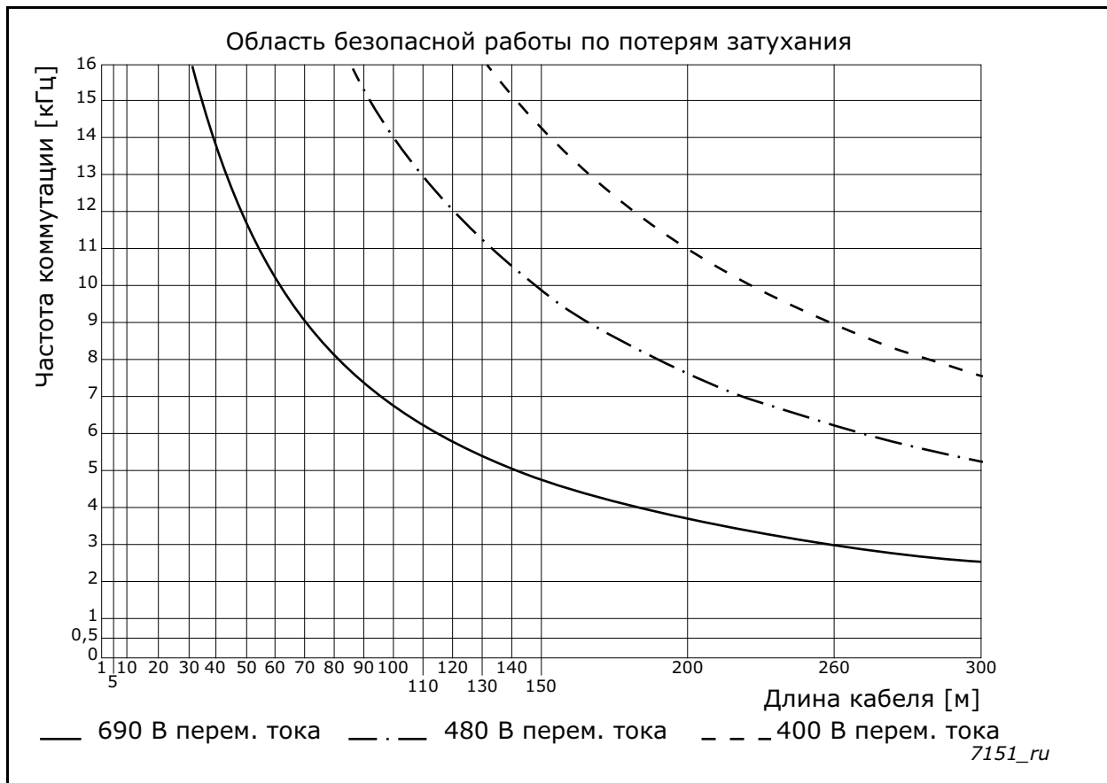
Рис. 38. Область безопасной работы для DUT 0590 6 0 S
