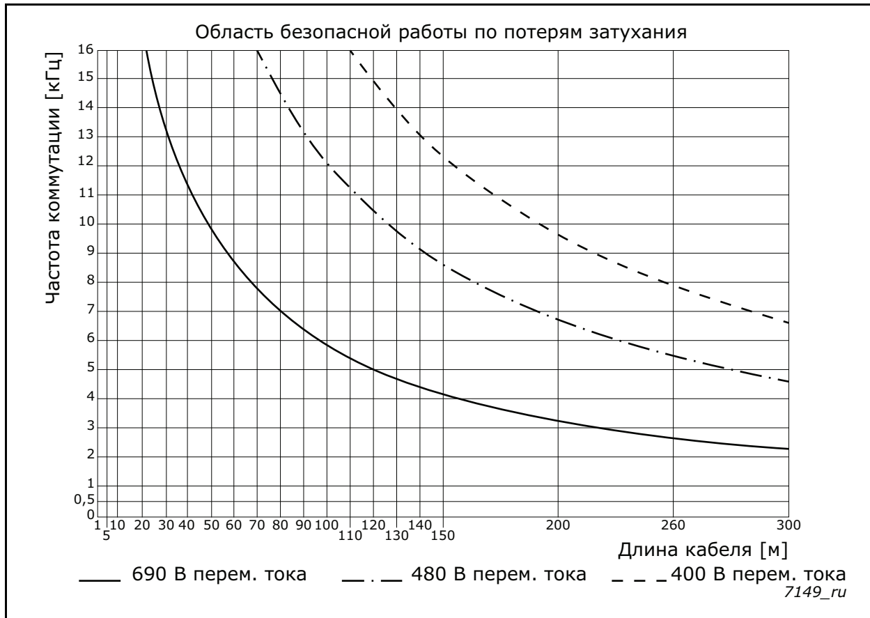
Рис. 36. Область безопасной работы для DUT 0280 6 0 S
