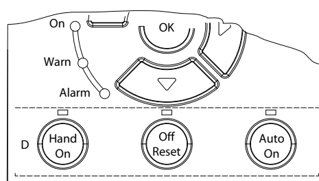
图 5.1 Hand On (手动启动)、Off/Reset (停止/复位) 和 Auto On (自动启动) 键在 NLCP 上的位置
