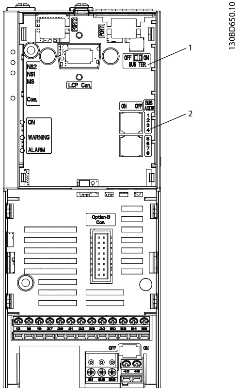
图 5.12 展示了带有 PROFIBUS 的控制盒的前面板。
