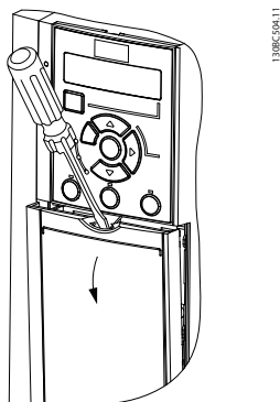
图 4.6 J1-J7 机箱规格的控制线路檢視
