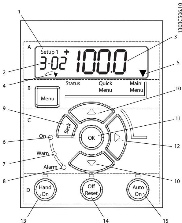
图 5.2 LCP 21 视图
