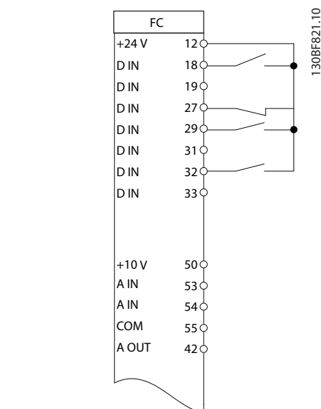
图 1.8 加速/减速
