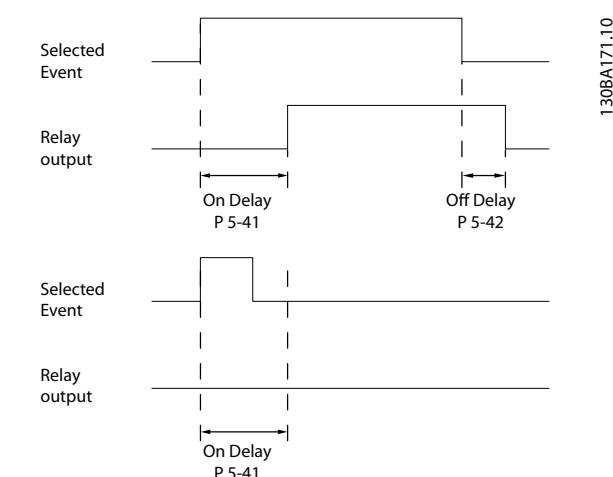
图 4.15 继电器打开延时
