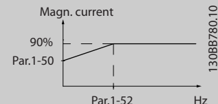
图 4.2 电机磁化
