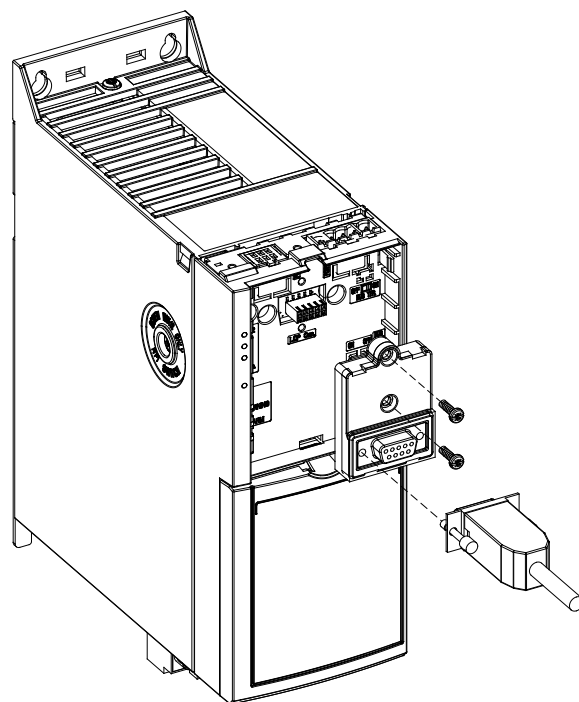
图 3.10 GLCP 适配器和连接电缆
