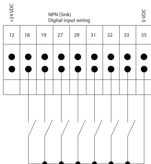
图 1.4 NPN（漏型）
