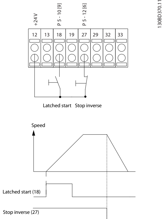
图 1.7 自锁启动/停止反逻辑
