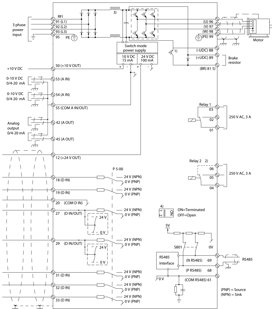
图 1.2 基本接线示意图
