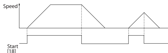
图 1.6 启动/停止
