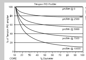
图 4.32 张力 PID 模式
