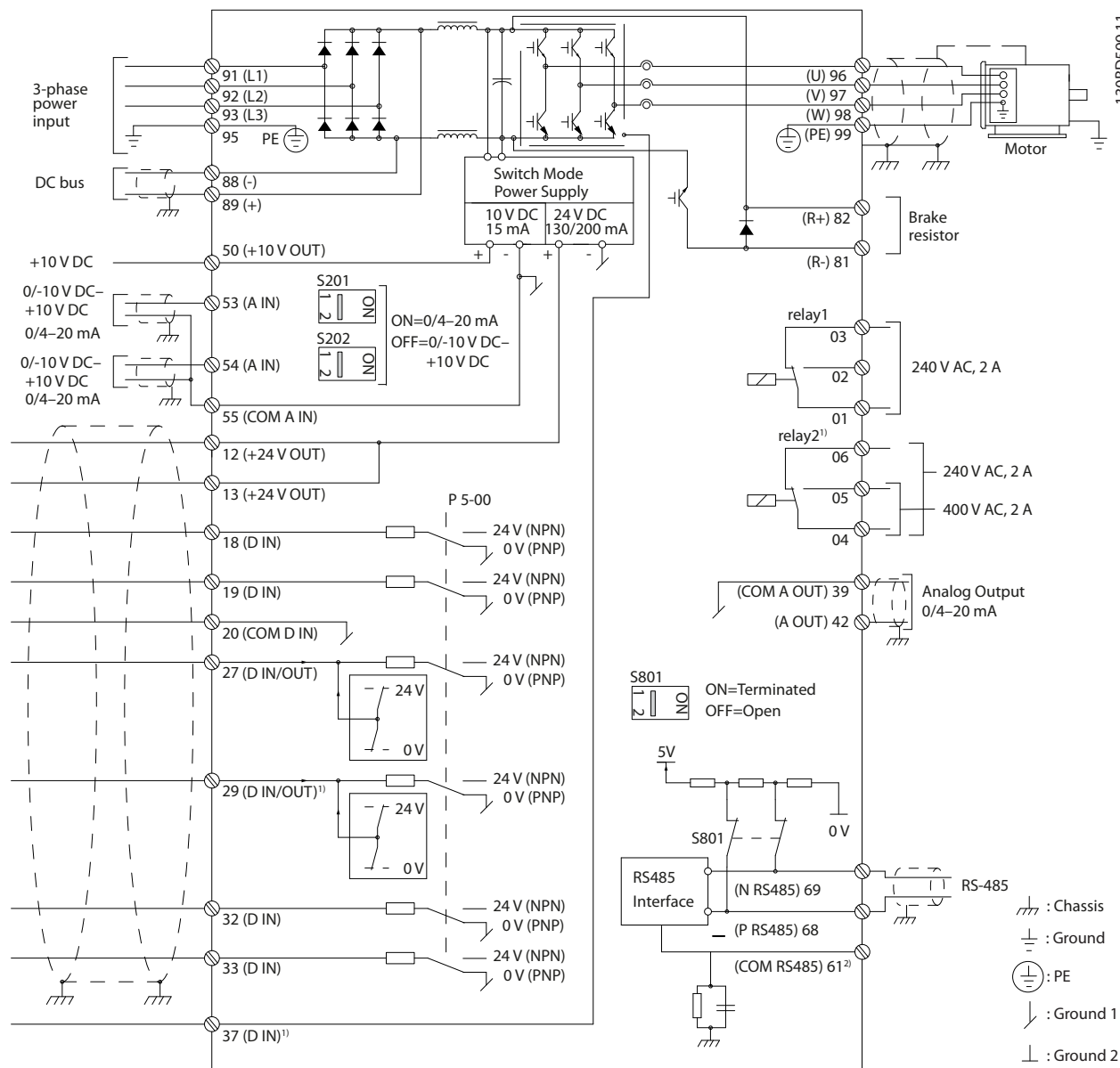
Bild 4.2 Grundläggande kopplingsschema
