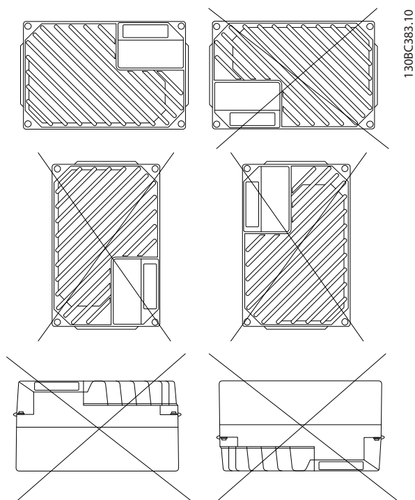
图 3.5 允许的安裝位置 - 卫生型应用
