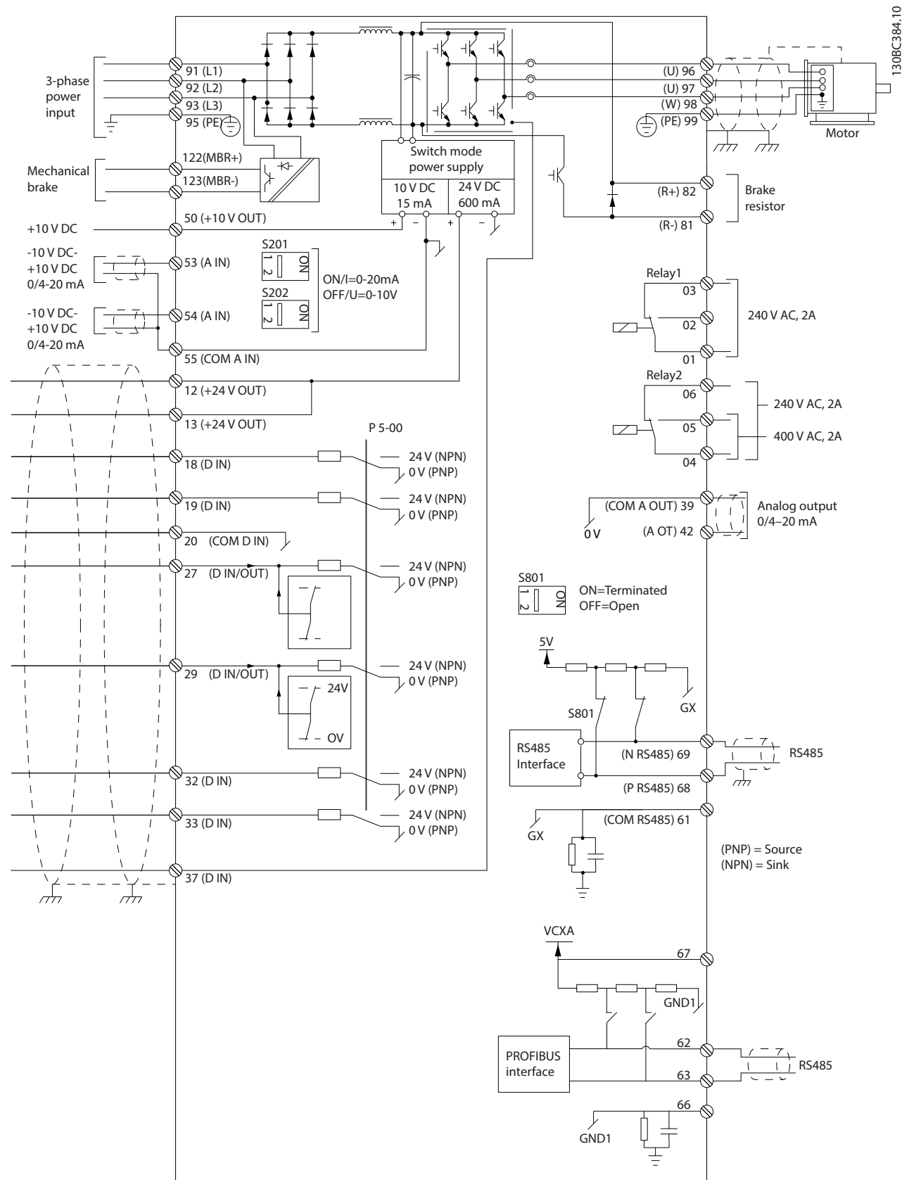
图 4.4 基本接线示意图
