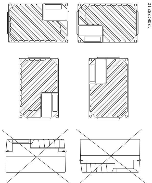
图 3.4 允许的安裝位置 - 标准应用
