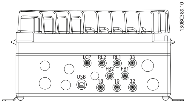
图 4.12 M12 套筒上的传感器/执行机构连接
