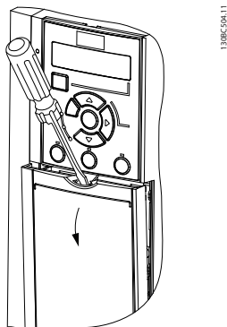
Illustration 4.4 Adgang til styreledninger
