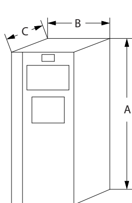
Illustration 9.4 Standard med IP21/UL/Type 1-sæt
