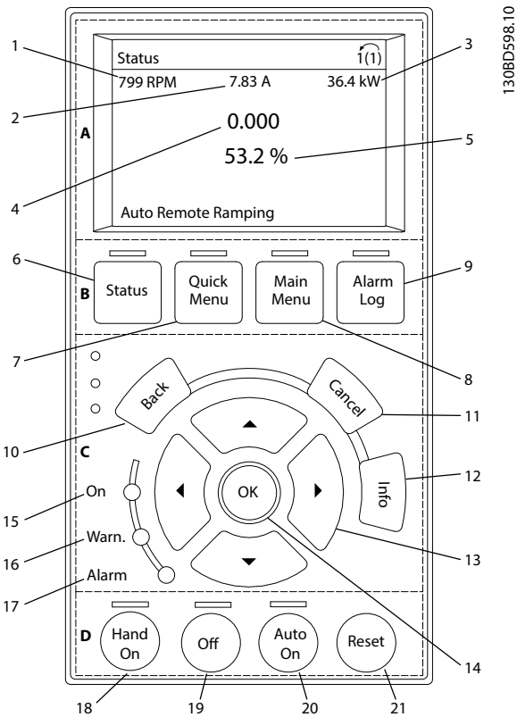
Abbildung 5.8 Grafisches LCP-Bedienteil (GLCP)
