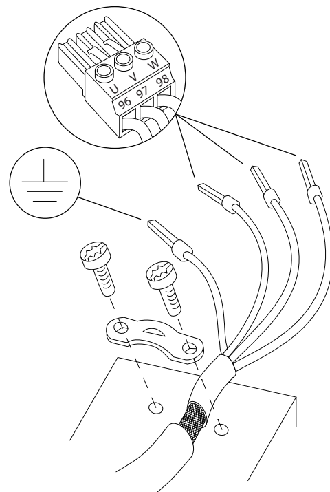
Εικόνα 4.5 Σύνδεση κινητήρα
