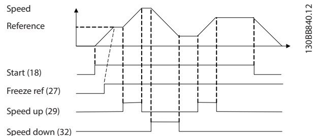
Εικόνα 7.1 Επιτάχυνση/επιβράδυνση
