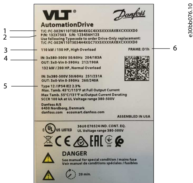
Abbildung 1: Beispiel für den Typencode auf dem Typenschild
