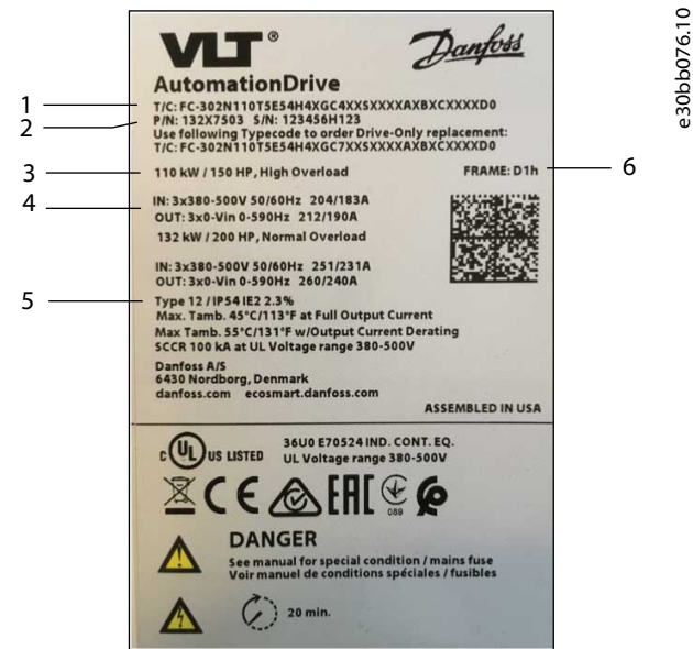
Ilustración 1: Ejemplo del código descriptivo de la placa de características
