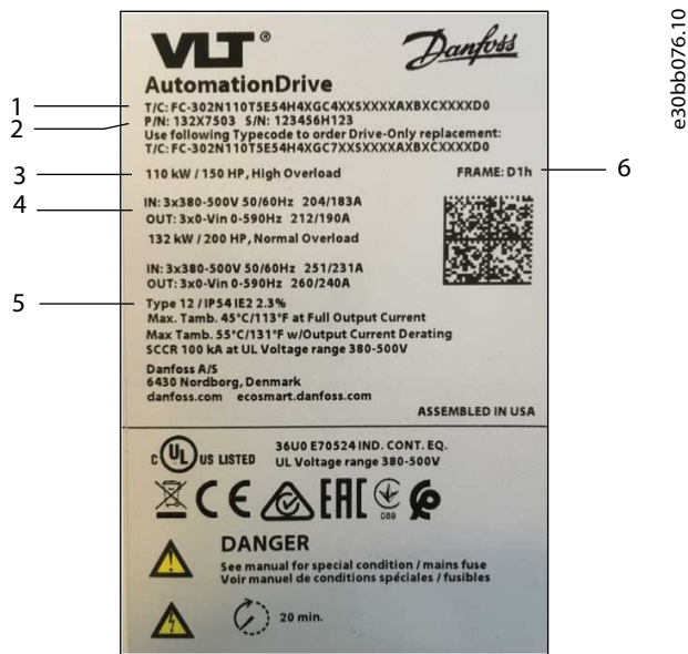
Ілюстрація 1: Приклад типового коду на паспортній таблиці
