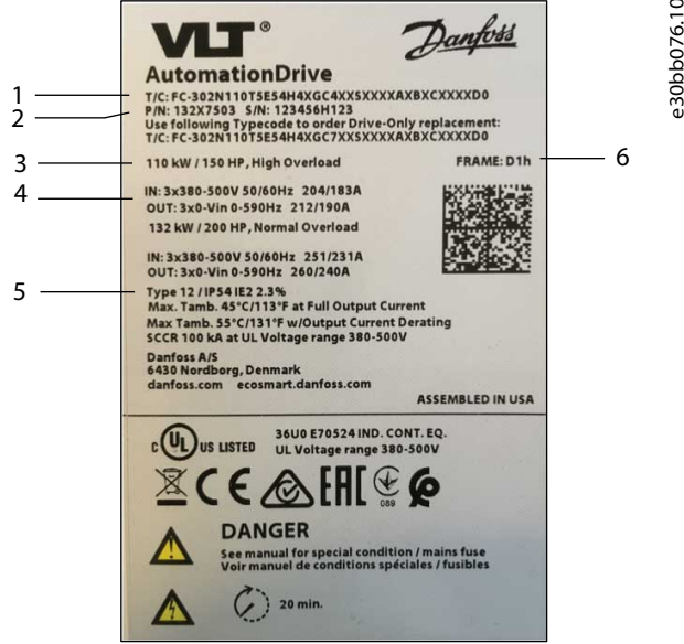
Çizim 1: İsim Plakasındaki Tür Kodu Örneği
