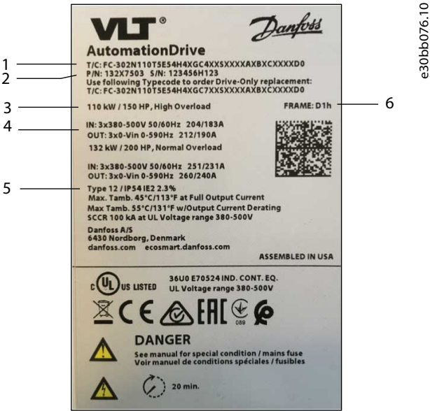
Illustrazione 1: Esempio di codice tipo riportato sulla targa
