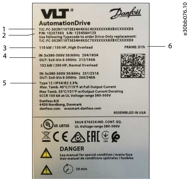
图解 1: 铭牌上的型号代码示例
