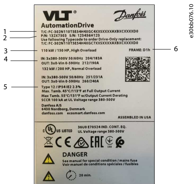
Рисунок 1: Пример кода типа на паспортной табличке
