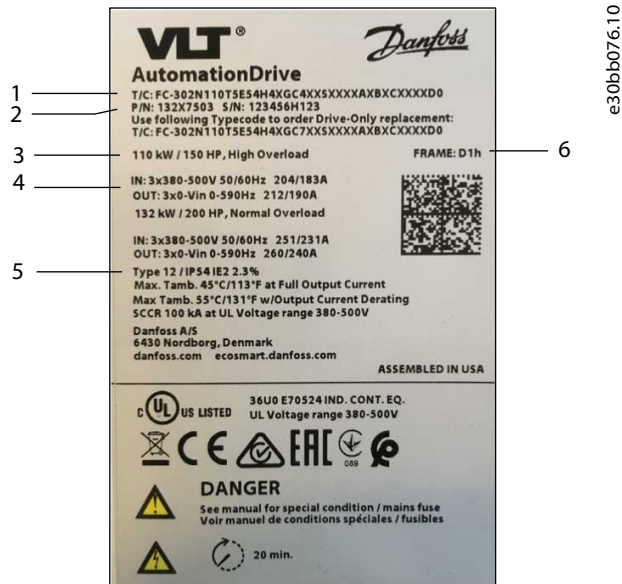
그림 1: 명판의 유형 코드 예시
