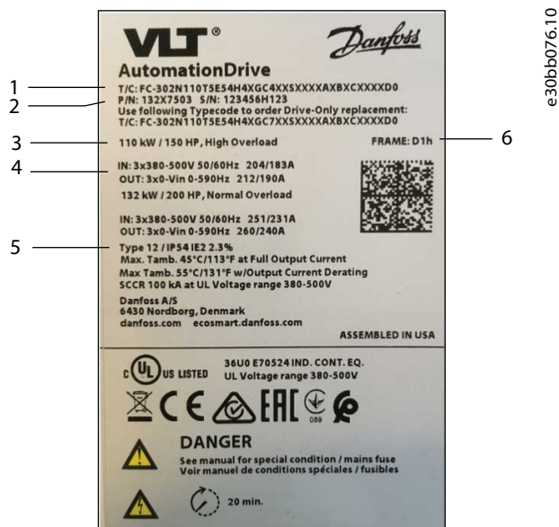
Ilustração 1: Exemplo de código do tipo na plaqueta de identificação
