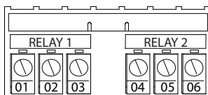
Afbeelding 5.19 Klemmen relais 1 en relais 2
