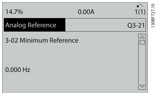
Afbeelding 6.6 Parameter 3-02 Minimumreferentie
