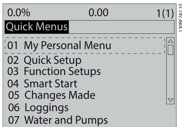
Afbeelding 6.1 Overzicht Snelmenu
