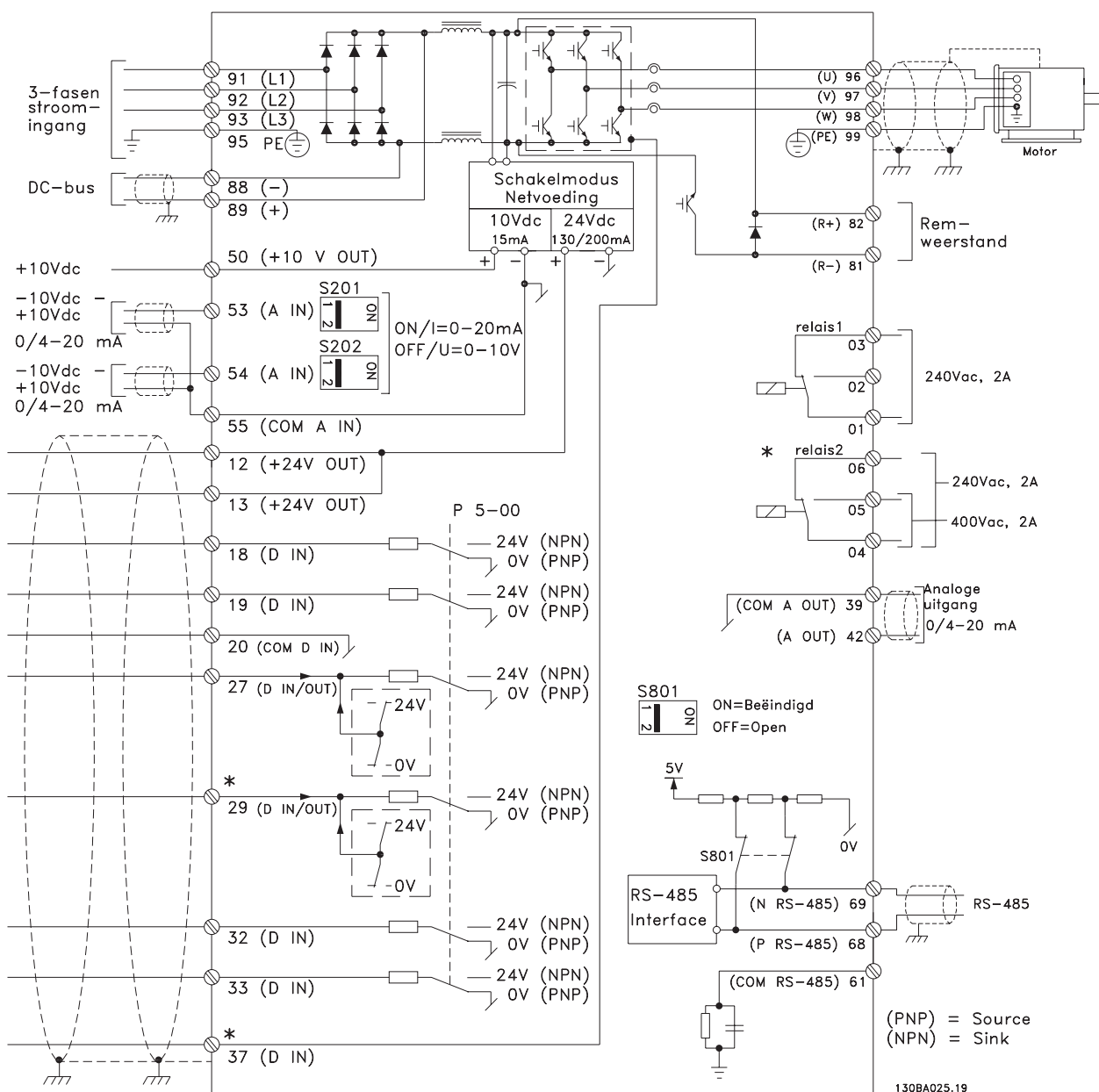
Afbeelding 5.2 Eenvoudig bedradingsschema
