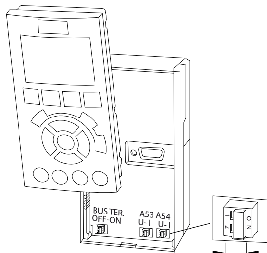
Afbeelding 5.23 Positie van de schakelaars voor klem 53 en 54
