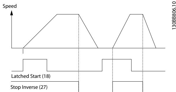
Afbeelding 7.3 Pulsstart/Stop geïnverteerd
