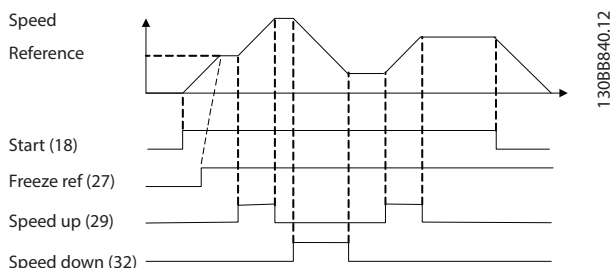
Afbeelding 7.1 Snelheid omhoog/omlaag
