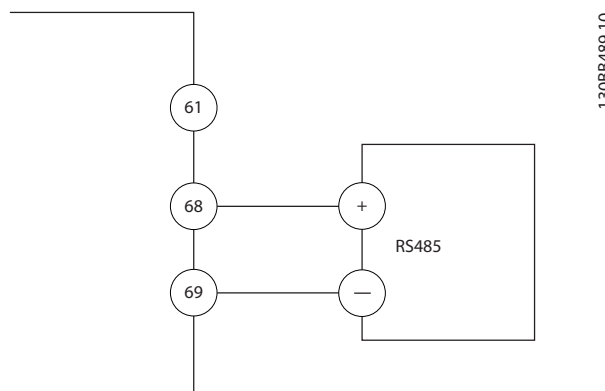
Afbeelding 5.22 Bedradingsschema voor seriële communicatie
