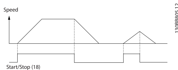
Afbeelding 7.2 Start-/stopcommando met STO-functie
