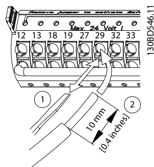
Afbeelding 5.21 Buigzame stuurdraden aansluiten
