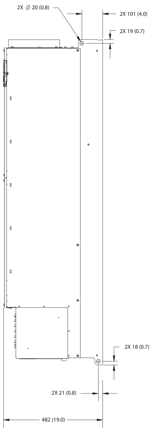
Afbeelding 9.15 Zijaanzicht E4h
