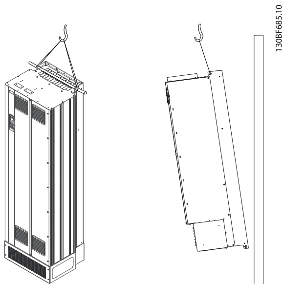
Afbeelding 4.2 Aanbevolen hijsmethode
