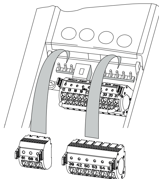
Afbeelding 5.17 Stuurklemposities
