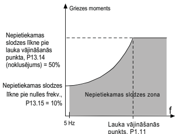
9.17. att. Aizsardzība nepietiekamas slodzes gadījumā
