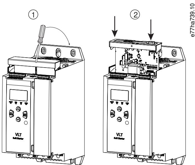
Abbildung 1: Installation der Erweiterungskarten
