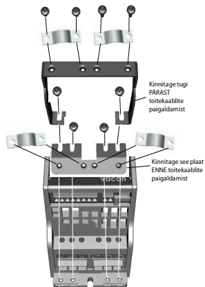
Joonis 5: PE-plaadi ja API kaablite kinnitamine, MI1 kuni MI3
