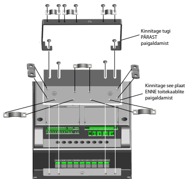
Joonis 6: PE-plaadi ja API kaablite kinnitamine, MI4 ja MI5
