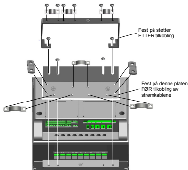
Figur 9: PE-platen og API-kabelholderen festes på, MI4–MI5
