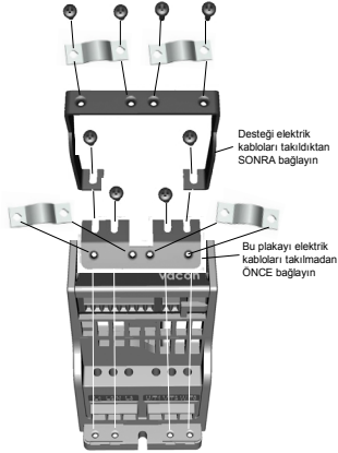
Şekil 5: PE'nin (plaka ve API kablo desteđi) bađlanması, MI1 - MI3
