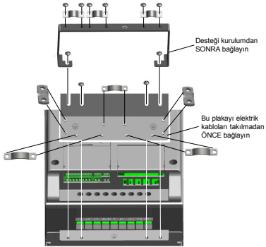
Şekil 6: PE'nin (plaka ve API kablo desteđi) bađlanması, MI4 - MI5
