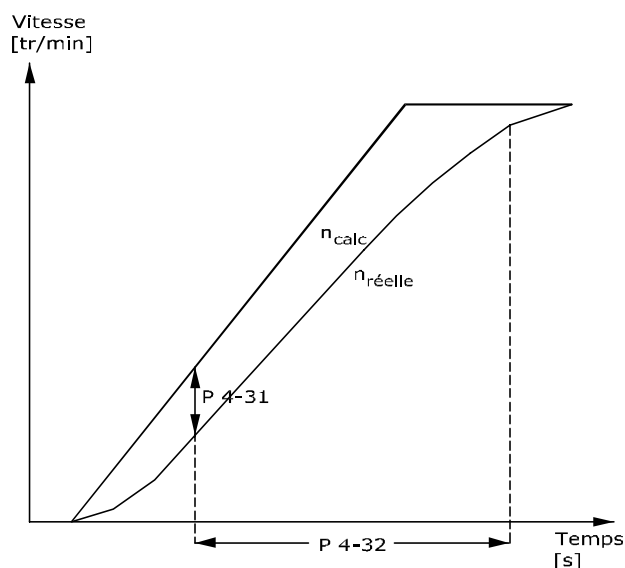
Illustration 4.8 Erreur vitesse signal de retour moteur
