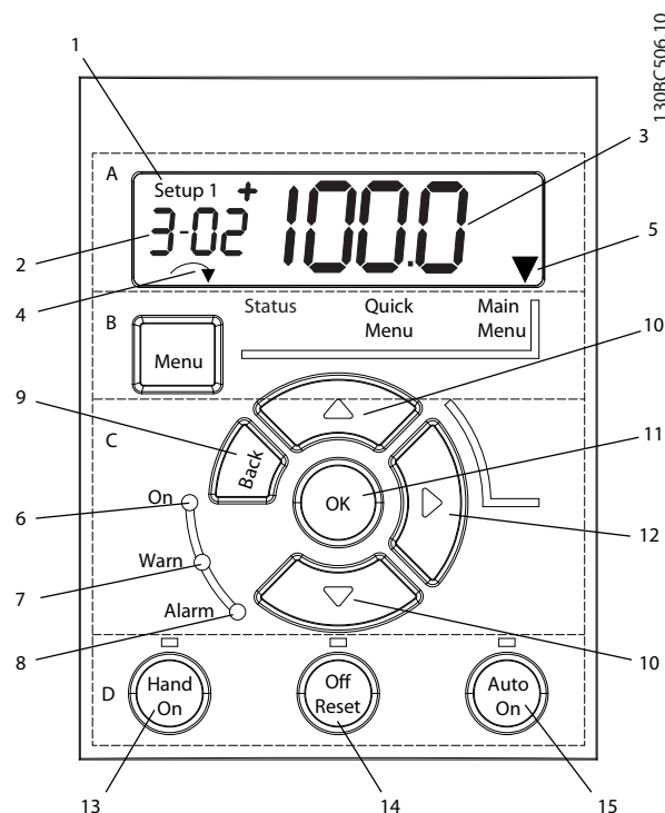
Illustration 3.1 Vue du NLCP
