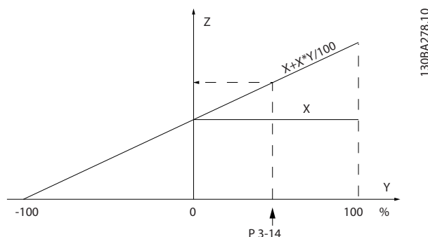
Illustration 4.4 Référence réelle
