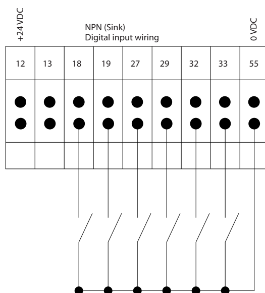
Illustration 1.4 NPN (dissipateur)
