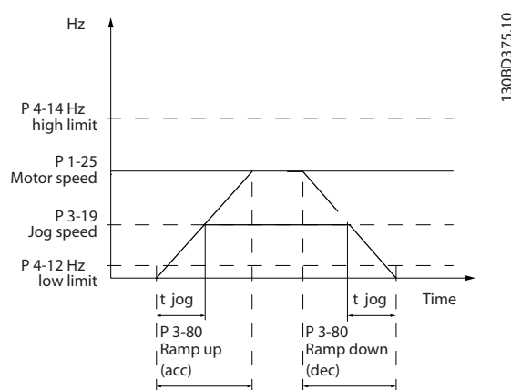
Illustration 4.6 Temps de la rampe de jogging
