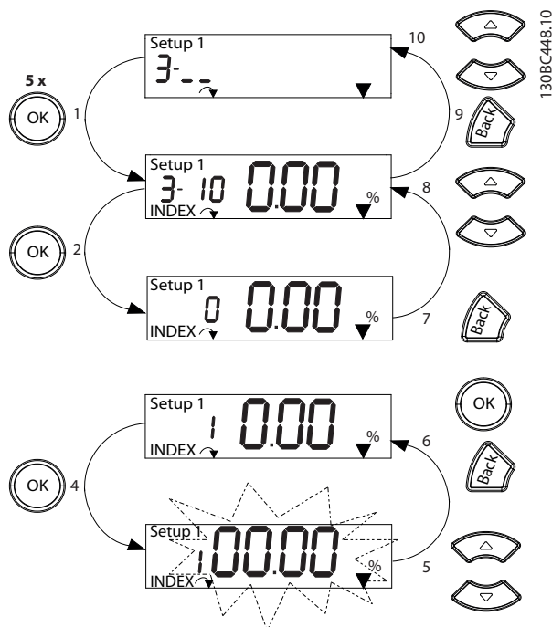
Illustration 3.7 Interactions dans Main Menu - Paramètres de tableau
