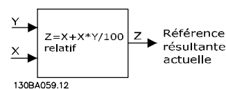
Illustration 4.3 Référence prédéfinie relative
