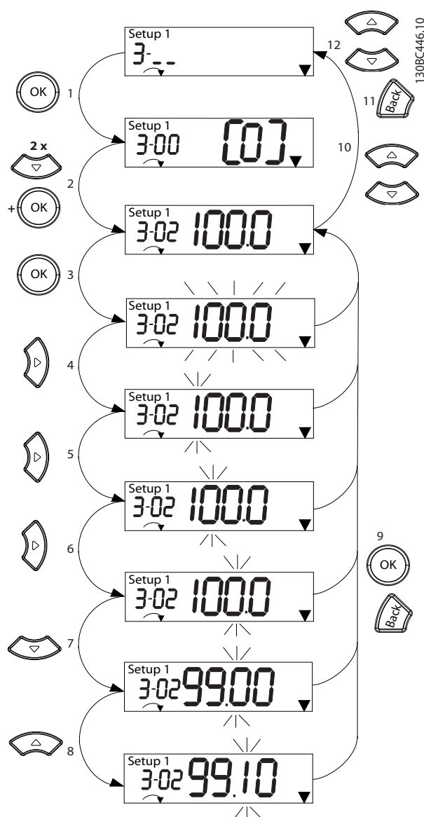
Illustration 3.5 Interactions dans Main Menu - Paramètres continus
