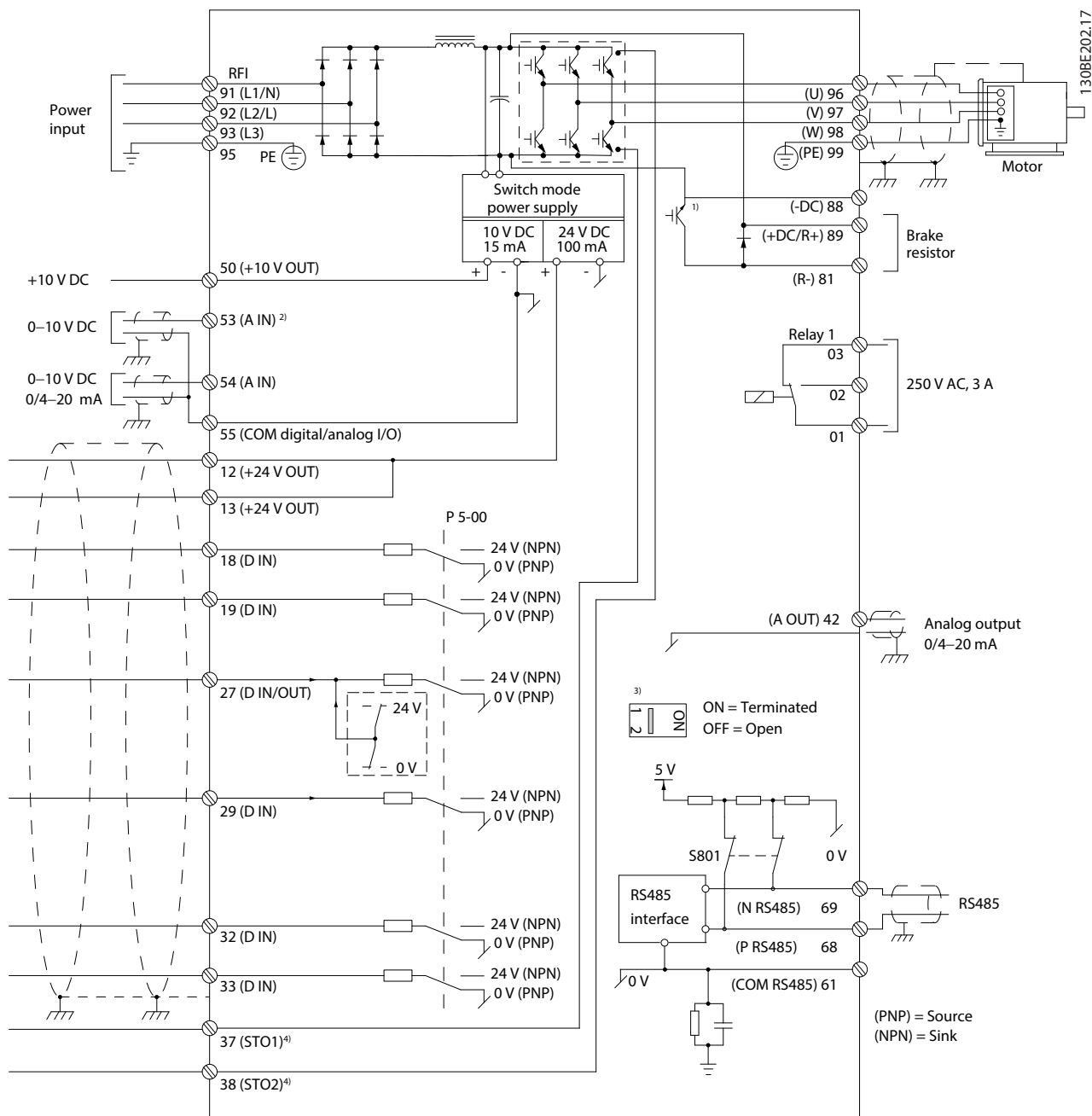
Illustration 1.2 Dessin schématique du câblage de base
