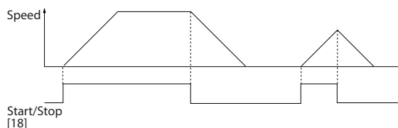
Illustration 1.6 Marche/arrêt
