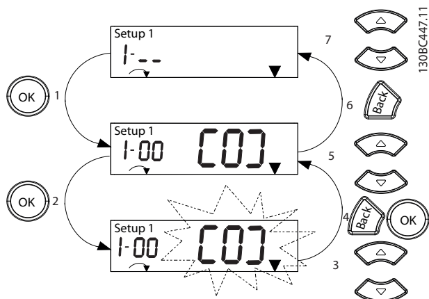
Illustration 3.6 Interactions dans Main Menu - Paramètres énumérés
