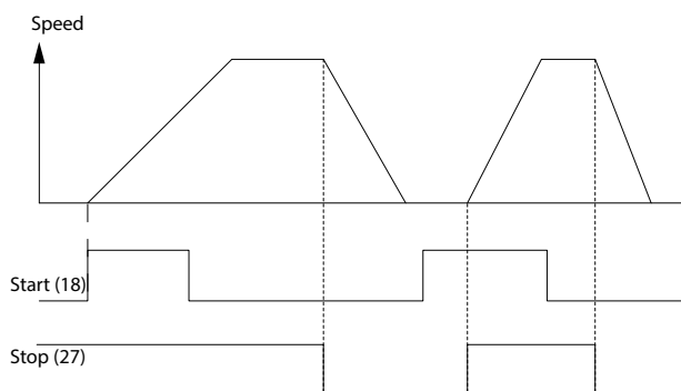
Illustration 1.7 Marche/arrêt par impulsion
