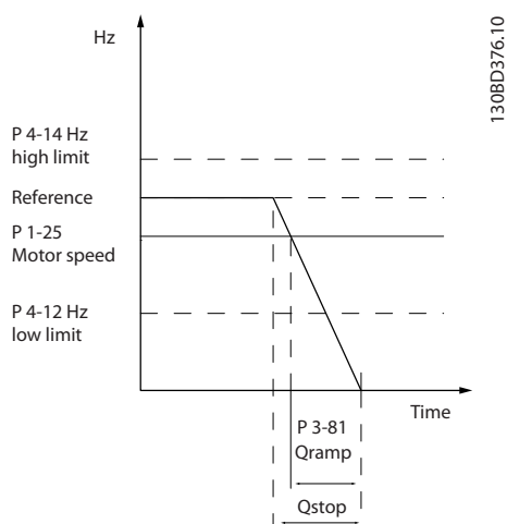
Illustration 4.7 Temps rampe arrêt rapide
