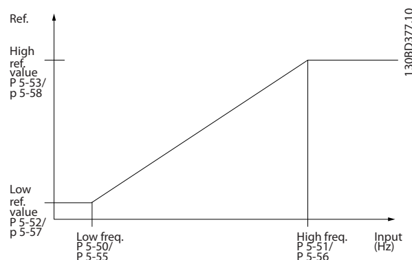
Illustration 4.12 Entrée impulsions
