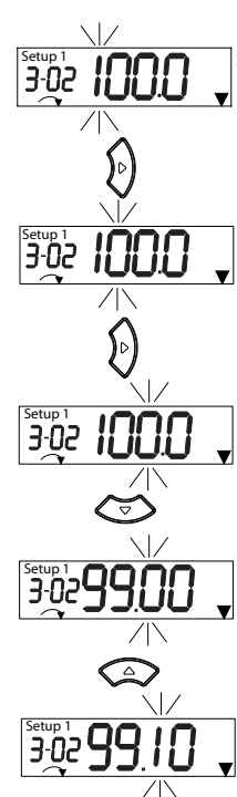
Illustration 3.3 Fonction de la touche droite
