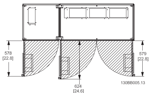
Illustration 3.7: Plads foran IP21/IP54 kapslingstyper, stelstørrelse F2
