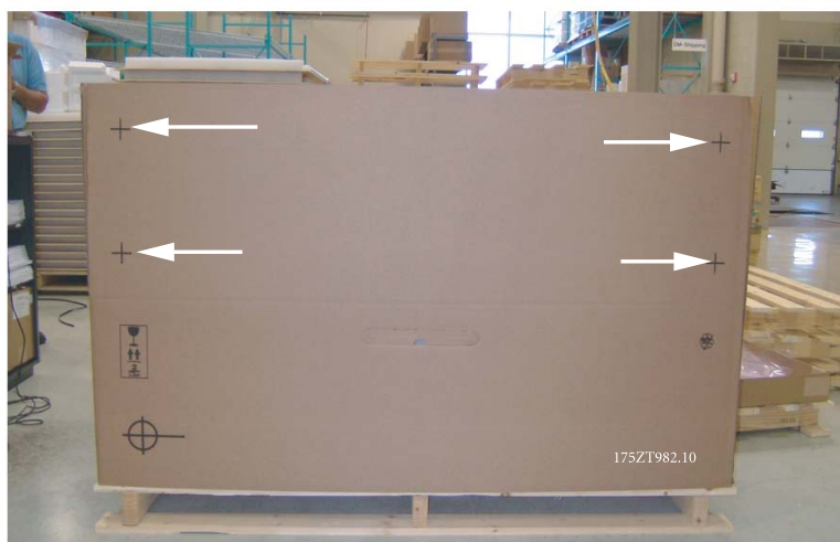
Illustration 3.2: Monteringsskabelon
