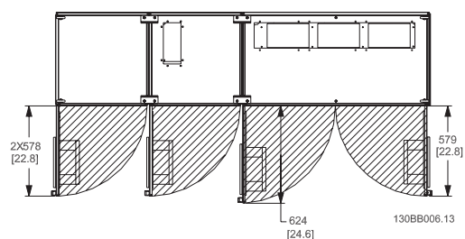
Illustration 3.8: Plads foran IP21/IP54 kapslingstyper, stelstørrelse F4
