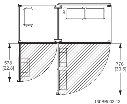
Illustration 3.5: Plads foran IP21/IP54 kapslingstype, stelstørrelse F1
