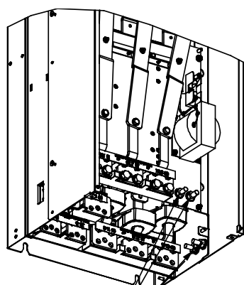
JORD- KLEMMER
