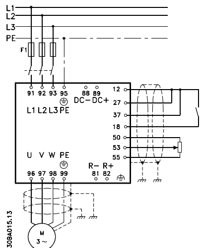
Illustration 3.1: I diagrammet vises en grundlæggende installation, herunder forsyningsstrøm, motor, start/stop-tast og potentiometer til hastighedsjustering.
