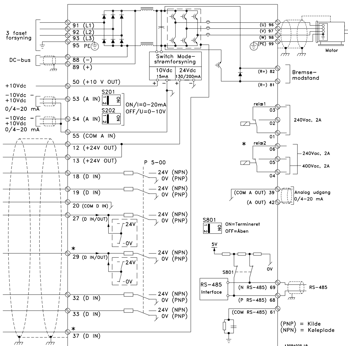
Illustration 4.10: Diagrammet viser alle elektriske klemmer uden optioner.
