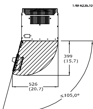
Illustration 3.4: Plads foran IP21/IP54-kapslingstyper, stelstørrelse D1 og D2.
