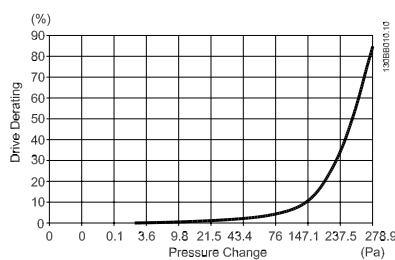
Illustration 3.12: E-stel derating vs. trykændringer (lille ventilator), P250T5 og P355T7-P400T7
