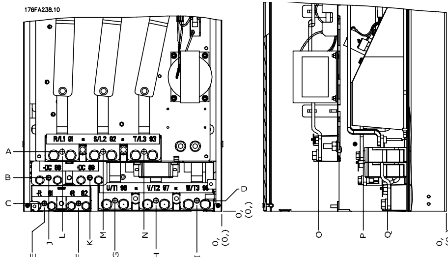
Illustration 3.9: Placering af effektilslutninger, stelstørrelse D3 og D4
