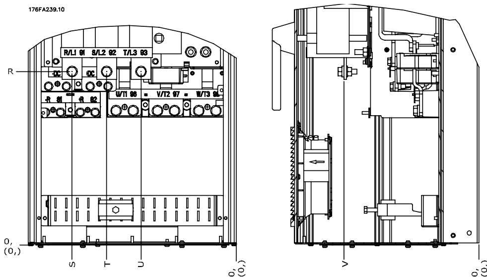
Illustration 3.10: Placering af effektilslutninger med afbryderkontakt, stelstørrelse D1 og D2
