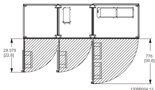
Illustration 3.6: Plads foran IP21/IP54 kapslingstype, stelstørrelse F3
