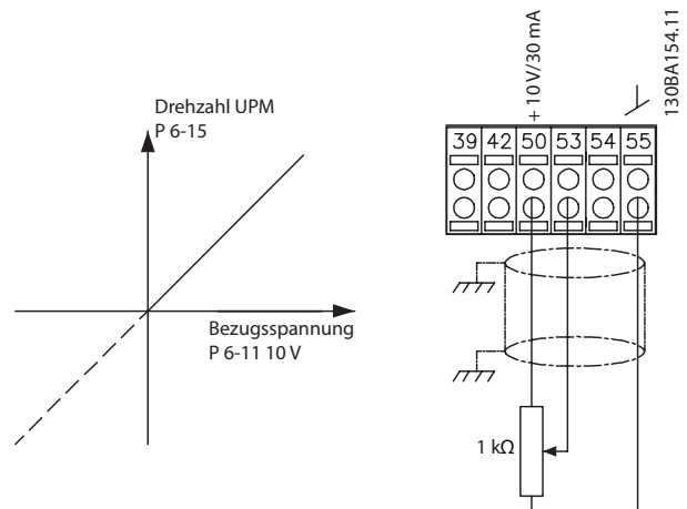
Abbildung 3.59 Potenziometer Sollwert
