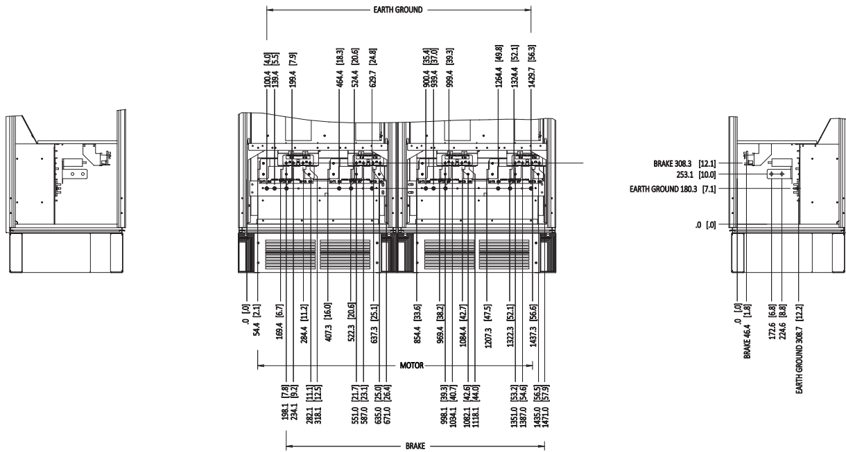
Abbildung 3.16 Anordnung der Klemmen – Vorderansicht, linke und rechte Seitenansicht. Die Stopfbuchsenplatte befindet sich 42 mm unter NN.
