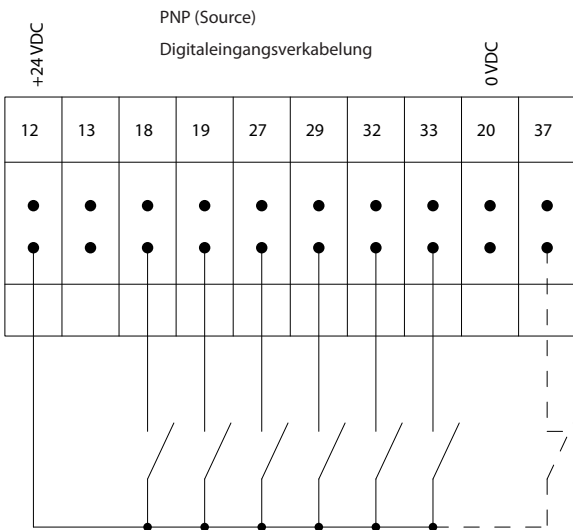
Abbildung 3.52 (PNP) = Quelle
