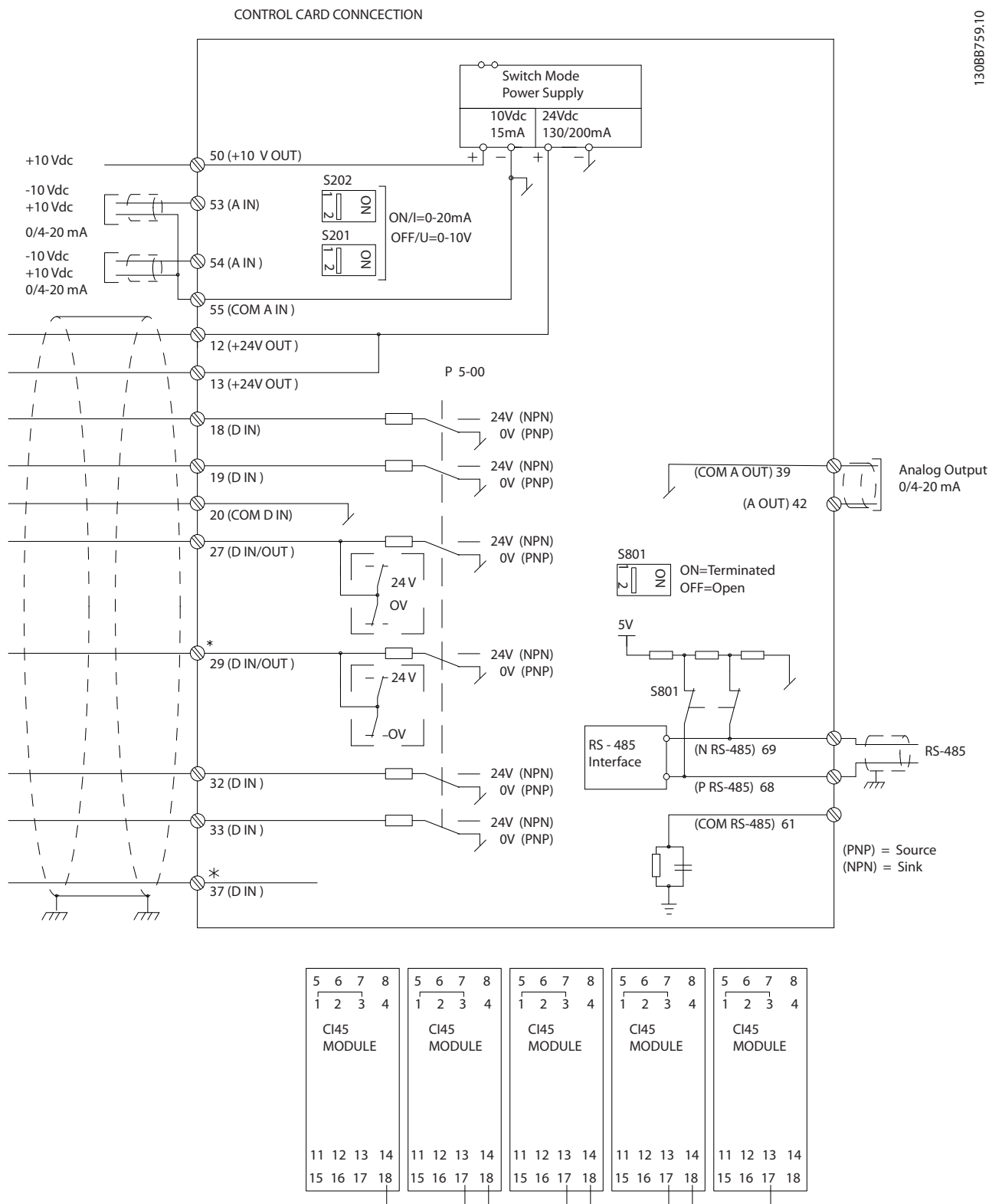
Abbildung 3.50 Anschlussplan
