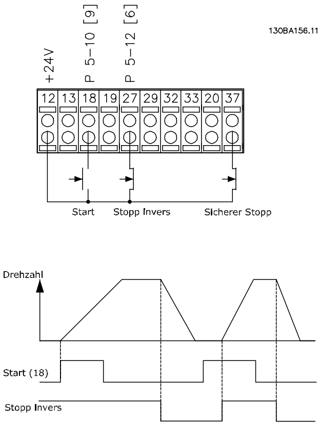
Abbildung 3.57 Verdrahtung Puls-Start/Stop
