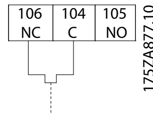
Ilustración 3.47 Termistor de la resistencia de frenado
