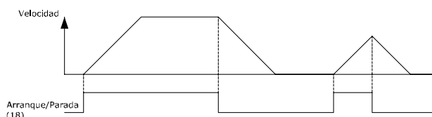
Ilustración 3.56 Cableado arranque/parada
