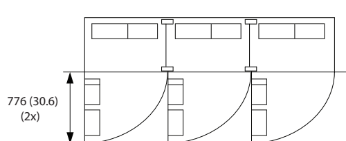
Ilustración 3.11 Espacio delante de un alojamiento de tamaño F14
