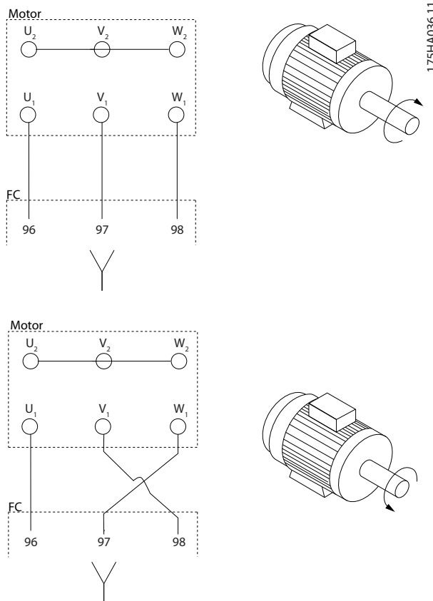
Ilustración 3.45 Cableado para giro del motor en sentido horario y antihorario
