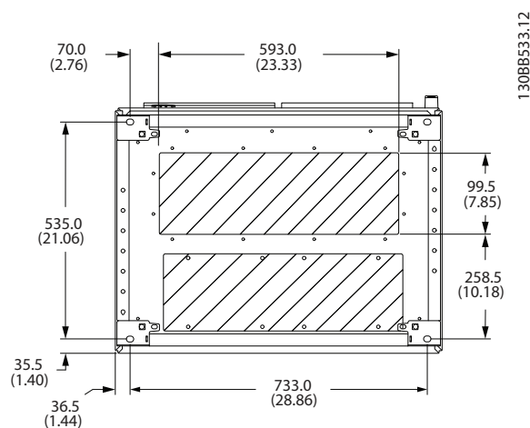
Ilustración 3.24 F8: entrada de cable vista desde la parte inferior del convertidor de frecuencia
