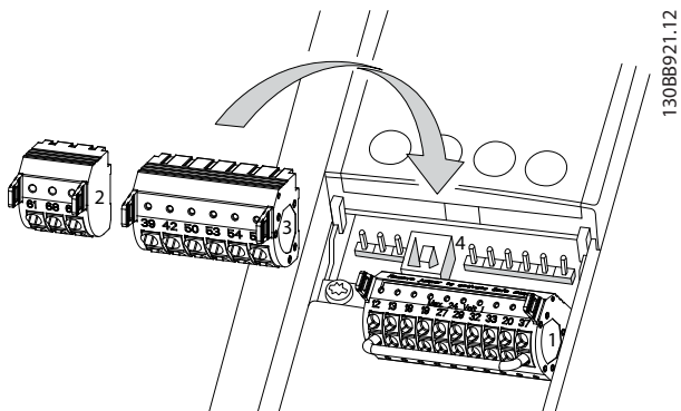
Ilustración 3.48 Desconexión de los terminales de control
