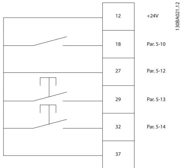
Ilustración 3.58 Aceleración/desaceleración
