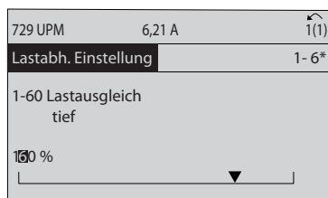
Abbildung 5.8 Displaybeispiel
