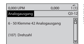
Abbildung 6.8 7. Schritt: Wählen Sie die verschiedenen Optionen mit den Auf/Ab-Navigationsstasten. Drücken Sie [OK].
