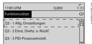
Abbildung 6.5 4. Schritt: Optionen der Funktionssätze werden angezeigt. Wählen Sie 03-1 Allgemeine Einstellungen. Drücken Sie [OK].
