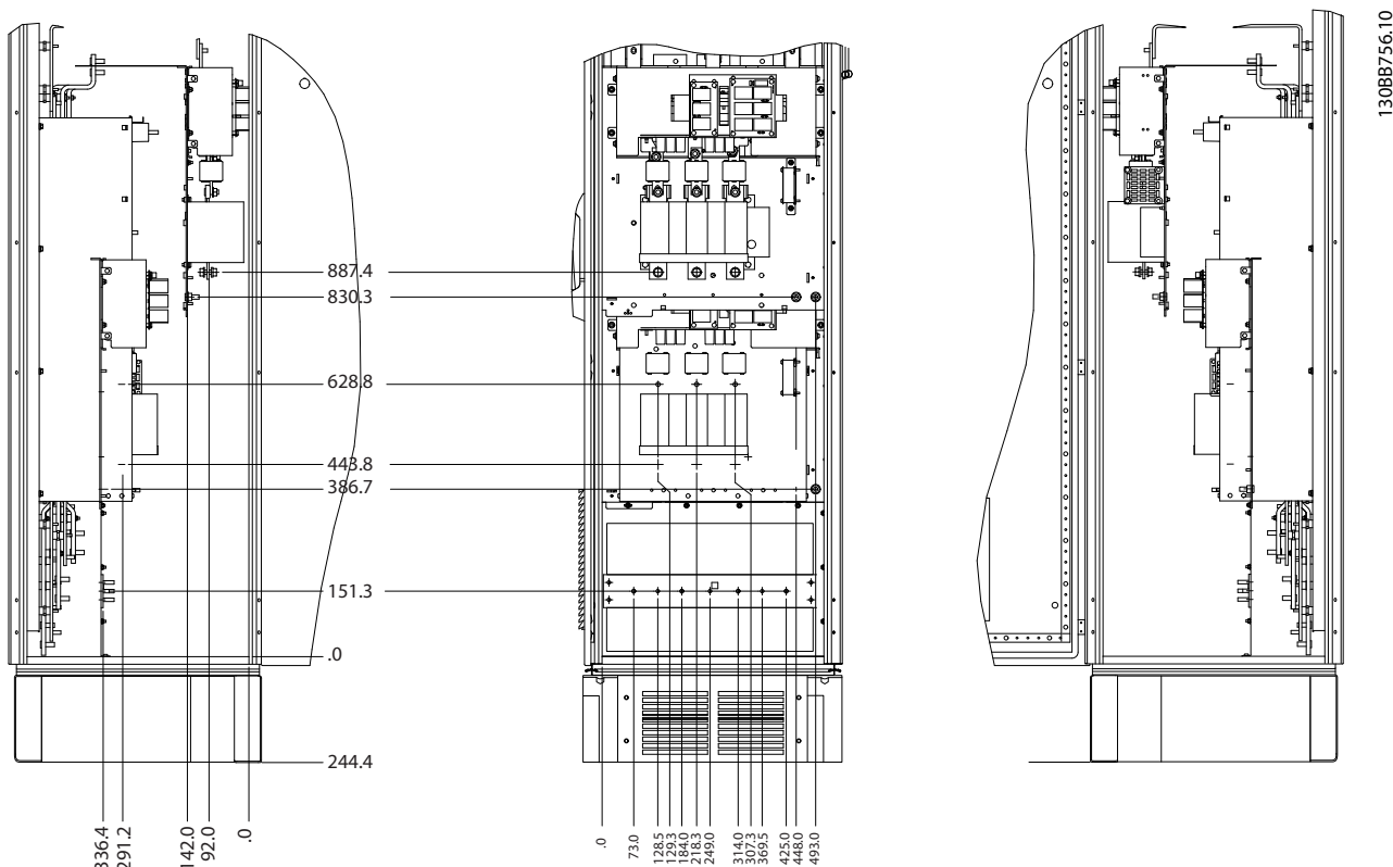
Kuva 3.14 Liitinten paikat - Optiokaappi (näkömä vasemmalta, edestä ja oikealta).
