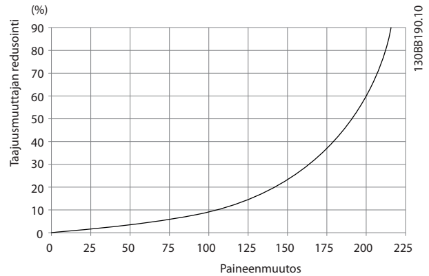
Kuva 3.16 F-kehyskesken redusointi vrt. paineenmuutos
