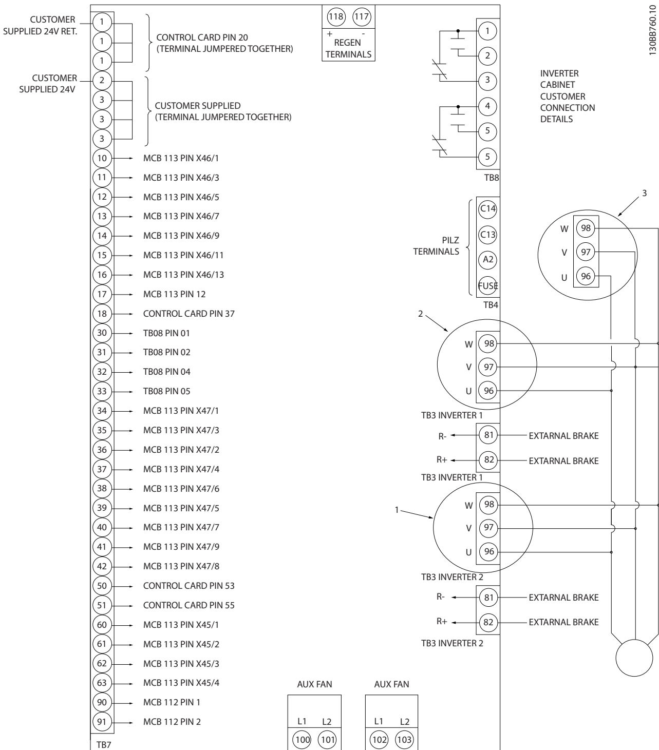
Kuva 4.10 Kaavio, jossa näkyvät kaikki sähköliittimet ilman optioita
