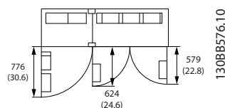
Kuva 3.8 Tila IP21/IP54-kotelointityypin, F12-kehyskoon edessä
