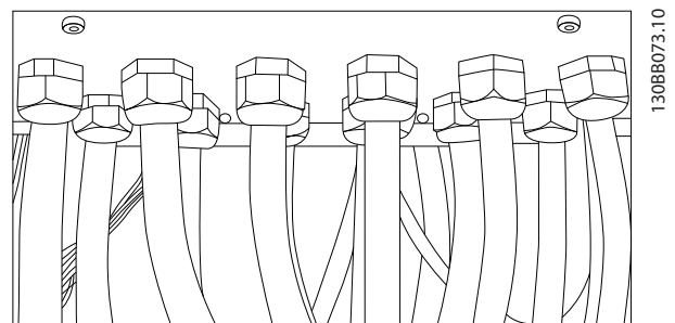
Kuva 3.17 Esimerkki läpivientilevyn asianmukaisesta asennamisesta.
