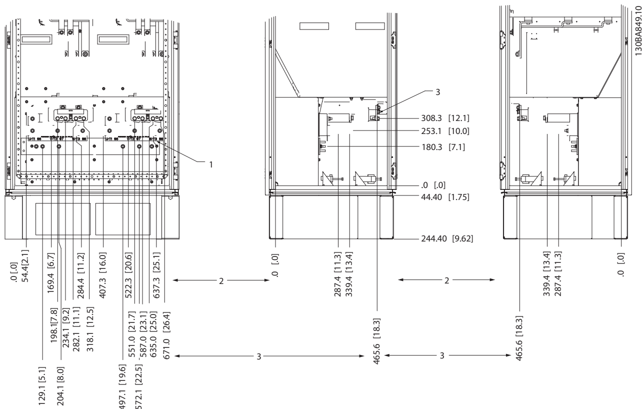
Kuva 3.11 Liitinten paikat - Vaihtosuuntaajakaappi (näkymä edestä, vasemmalta ja oikealta). Läpivientilevy on 42 mm .0-tason alapuolella.
