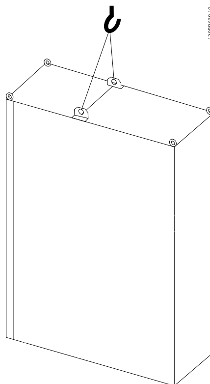
Kuva 3.2 Suositeltava nostotapa, kehyskoko F9/F10.
