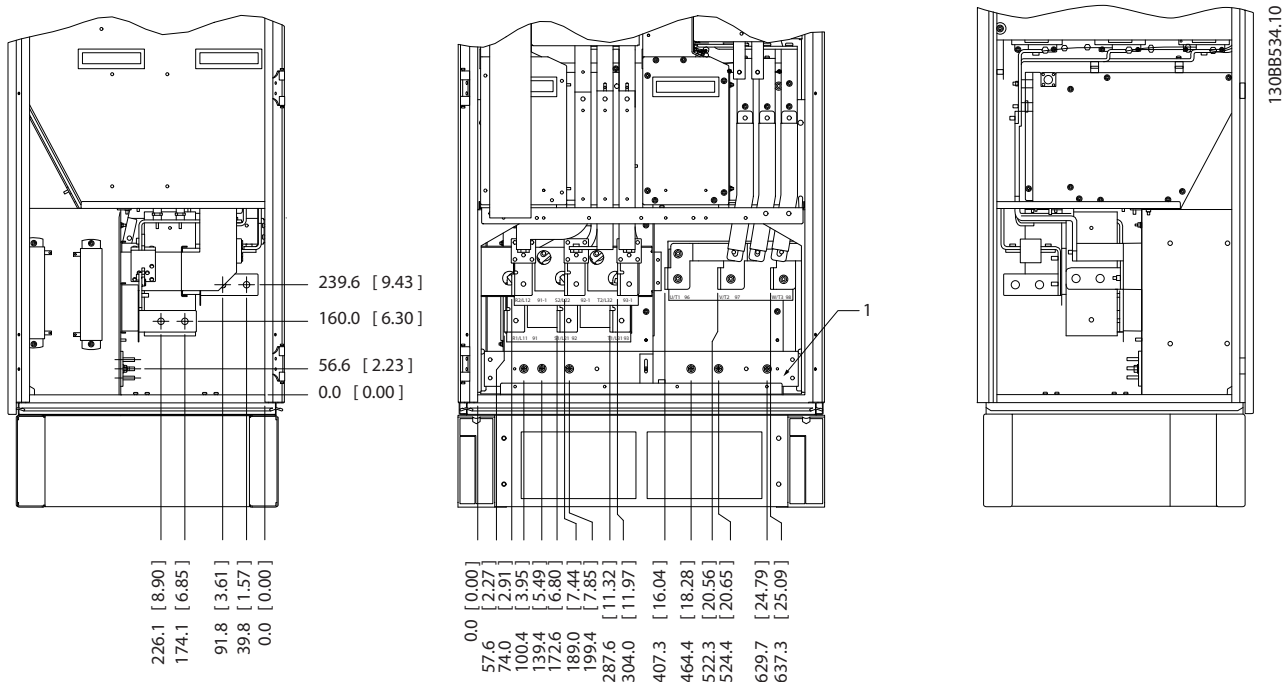
Kuva 3.13 Liitinten paikat - Tasasuuntaaja (näkömä vasemmalta, edestä ja oikealta). Lämpivientilevy on 42 mm .0-tason alapuolella.
