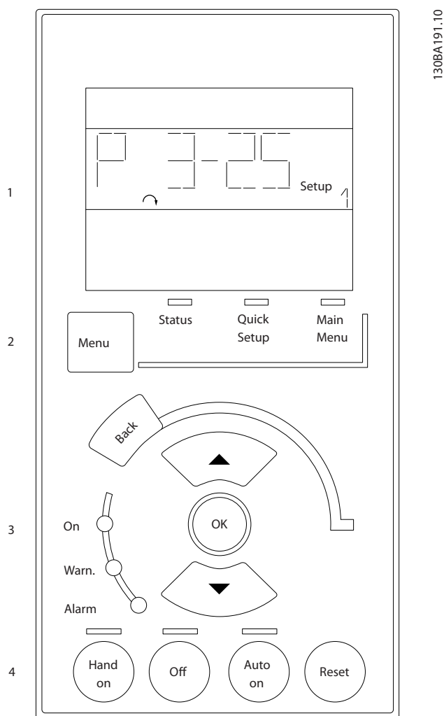
Kuva 5.1 Numeerinen paikallisohtauspaneeli (LCP)
