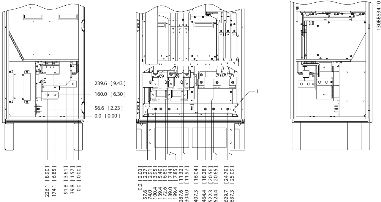
Kuva 3.10 Liitinten paikat - Vaihtosuuntaaja- ja tasasuuntaajakaappi - F8 ja F9 (näkymä edestä vasemmalta ja oikealta). Läpivientilevy on 42 mm .0-tason alapuolella.
