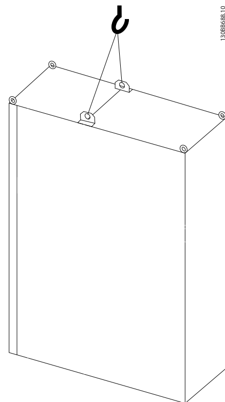
그림 3.2 들어 올리는 방법(권장), 프레임 용량 F9/F10.
