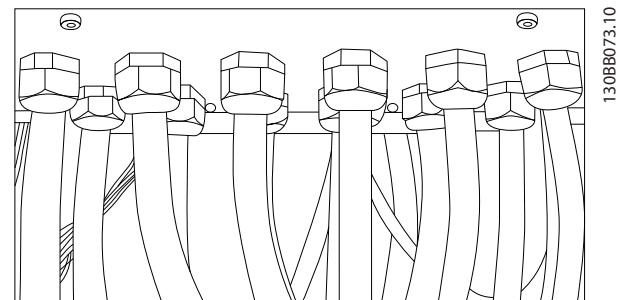
그림 3.17 글랜드 플레이트의 올바른 설치 예
