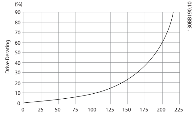
그림 3.16 F 프레임 용량 감소와 압력 변화 간 비교 인버터 통풍량: 985 m³/h (580 cfm)
