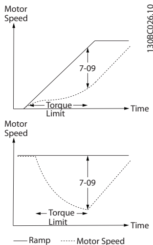
Abbildung 3.51 Drehzahlabweichung zwischen Rampe und Ist Drehzahl
