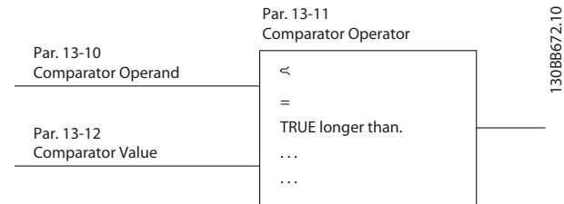
Abbildung 3.54 Vergleichler
