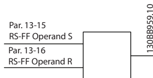
Abbildung 3.55 Reset/Set Flip Flops
