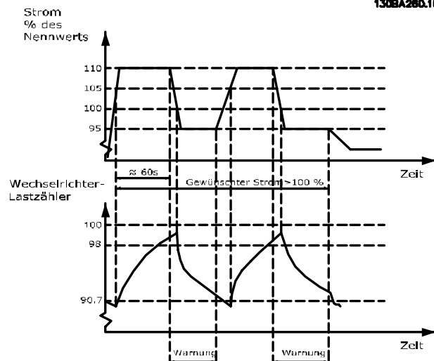
Abbildung 3.64 Ausgangsstrom bei Überlastbedingung
