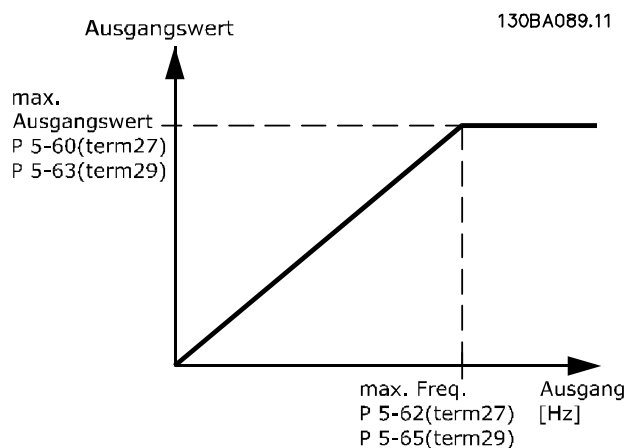
Abbildung 3.40 Konfiguration der Pulsausgänge
