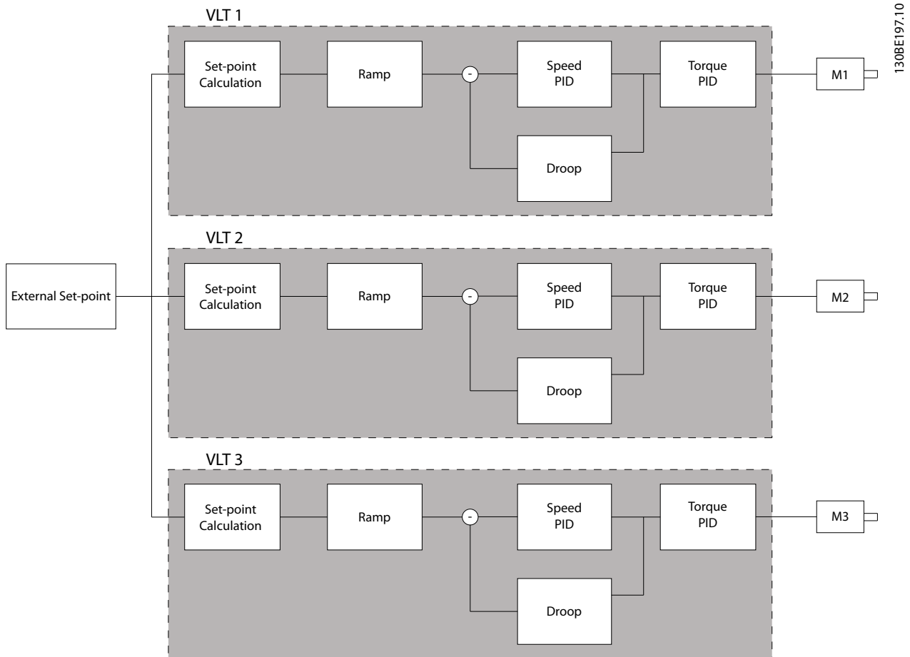
Abbildung 3.47 Drehzahlregler Änderungsgeschwindigkeit
