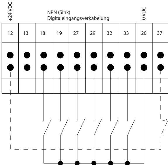
Abbildung 1.4 (NPN) = Verbraucher
