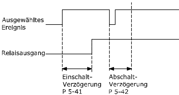
Abbildung 3.38 Aus Verzögerung, Relais
