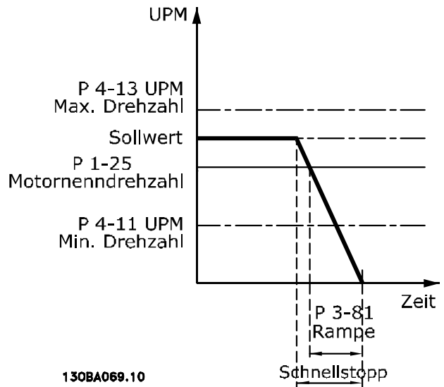
130BA069.10 Abbildung 3.28 Rampenzeit Schnellstopp
