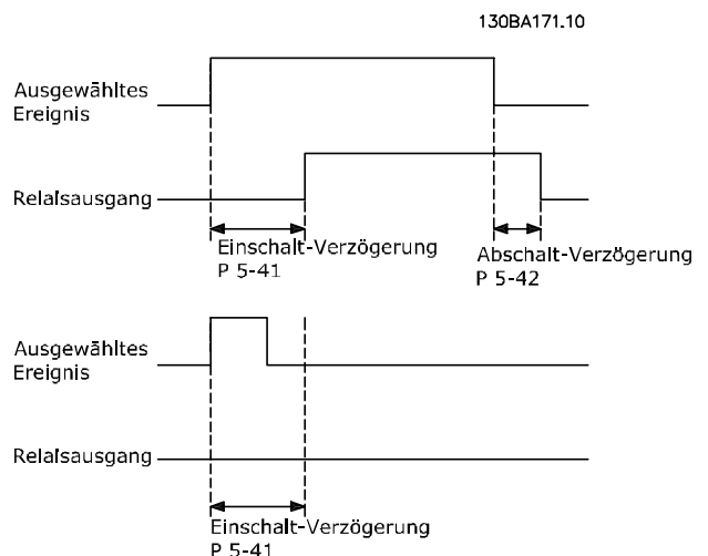
Abbildung 3.37 Ein Verzögerung, Relais
