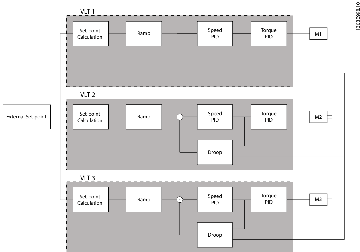
Abbildung 3.48 Drehzahltrimmung
