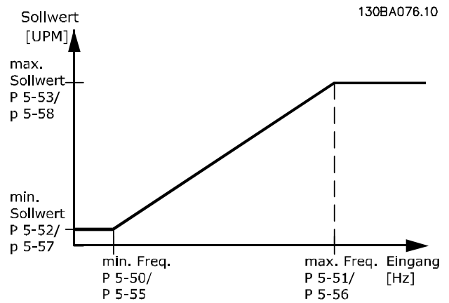
Abbildung 3.39 Pulseingang
