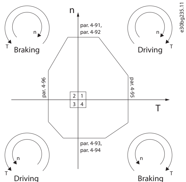
Abbildung 3.34 Directional Limits (richtungsabhängige Begrenzung)
