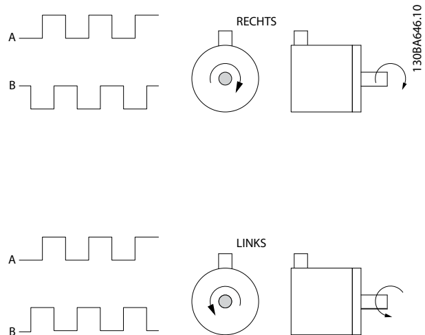
Abbildung 3.42 Drehgeber-Drehrichtung
