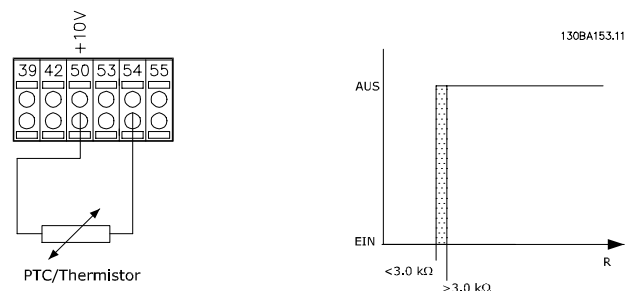
Abbildung 3.14 PTC-Thermistorverbindung - Analogeingang
