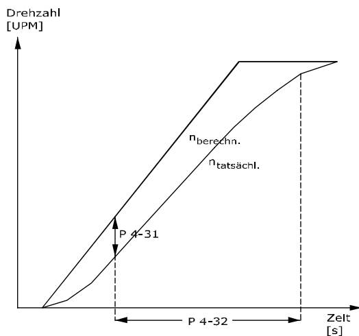
Abbildung 3.31 Drehgeber max. Fehlabweichung
