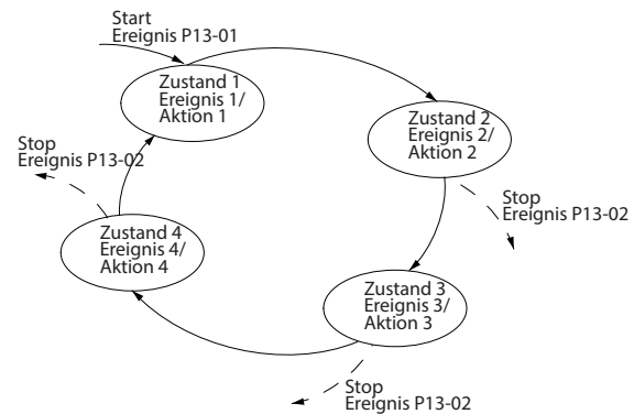
Abbildung 3.53 Ereignisse und Aktionen
