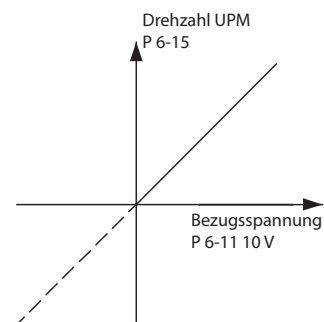
Abbildung 1.9 Potenziometer Sollwert
