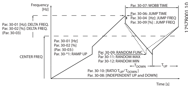
Abbildung 3.72 Wobbel-Funktion
