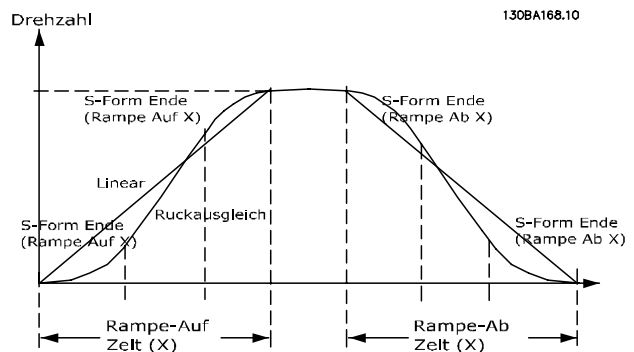
Abbildung 3.26 Lineare Rampenzeiten
