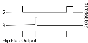
Abbildung 3.56 Flip Flop-Ausgänge
