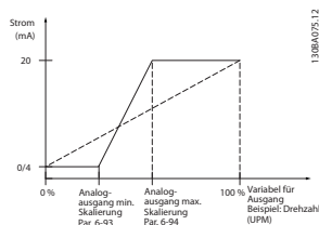
Abbildung 3.45 Ausgang max. Skalierung
