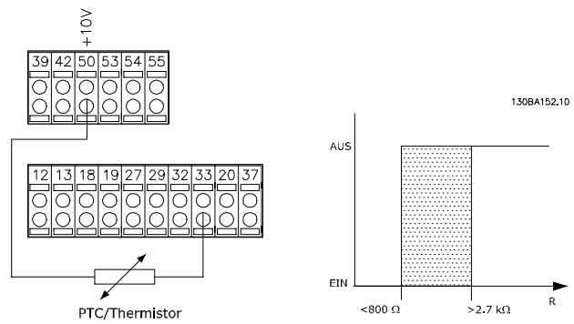
Abbildung 3.13 PTC-Thermistorverbindung - Digitaleingang
