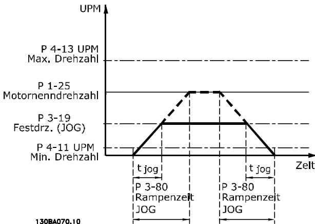
130BA070.10 Abbildung 3.27 Rampenzeit JOG
