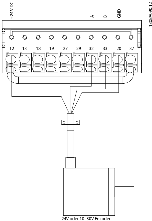
Abbildung 3.41 Drehgeberverbindung
