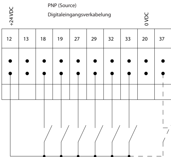
Abbildung 1.3 (PNP) = Quelle
