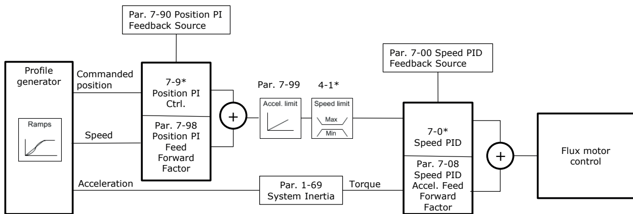
Abbildung 4.3 Positionierungs- und Synchronisierungsmodus
