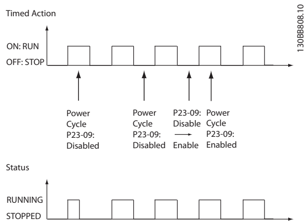
Abbildung 3.70 Reaktivierungstest-Diagramm
