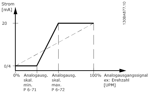
Abbildung 3.46 Ausgang max. Skalierung
