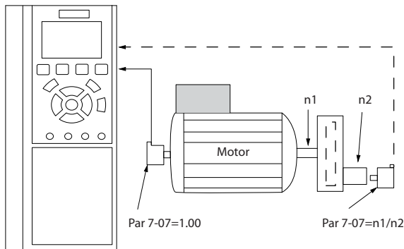
Abbildung 3.50 Drehzahlregler Getriebeübersetzung
