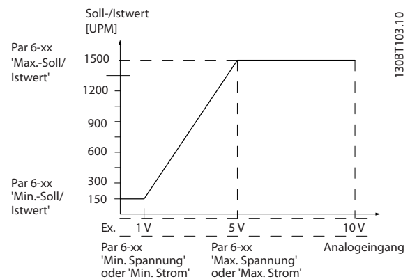
Abbildung 3.43 Analogeingang 1
