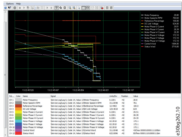
Abbildung 3.67 Detaillierte Serviceprotokollansicht, 250 ms
