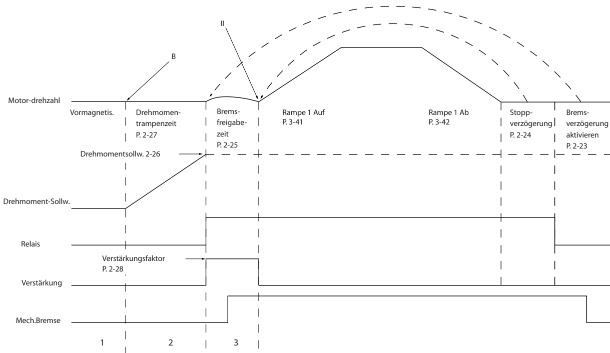
Abbildung 3.20 Sequenz zum Lüften der Bremse bei mechanischer Bremsansteuerung für Vertikalförder- und Hubanwendungen
