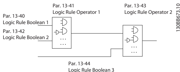
Abbildung 3.57 Logikregeln
