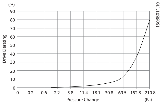
图 3.3 E 机箱的降额与 降容 变频器气流量: 850 cfm (1445 m³/h)
