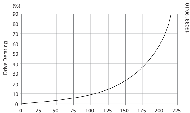
图 3.4 F 机箱的降额与 降容 变频器气流量: 580 cfm (985 m³/h)
