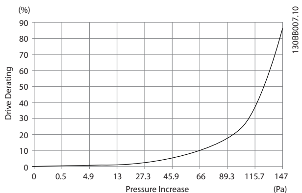
图 3.2 D 机箱的降额与 降容 变频器气流量: 450 cfm (765 m³/h)
