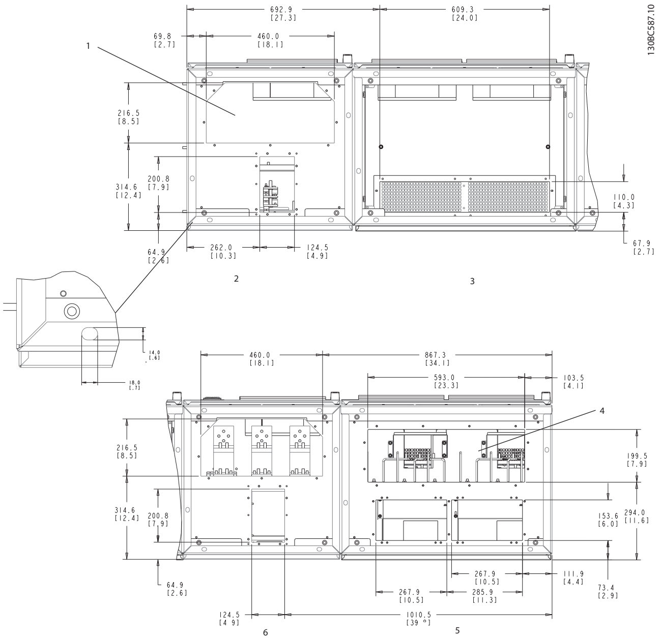
底视图, F18
