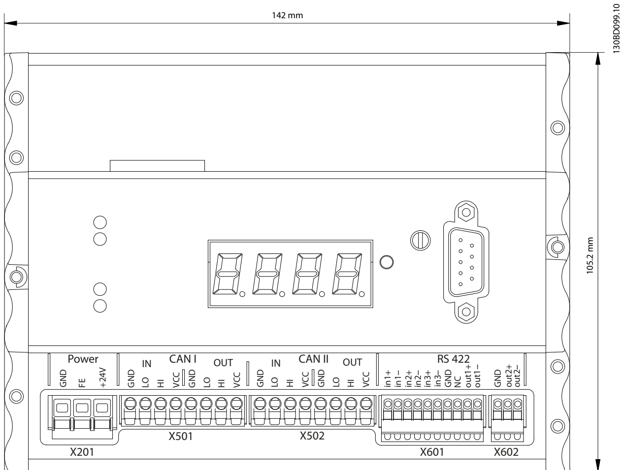
Abbildung 11.2 Vorderansicht
