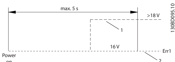
Abbildung 8.1 Unterspannung bei Netz-Ein
