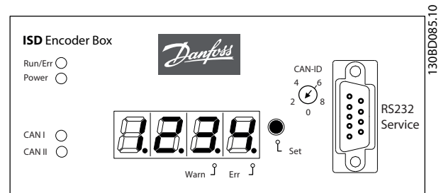
Abbildung 4.1 Geberbox-Display
