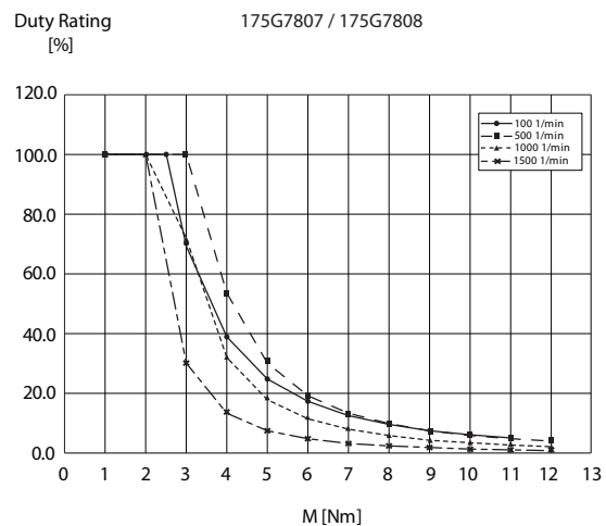
图 12.18 175G7807/08/15/16/23/24 伺服电机的 S3 特性曲线
