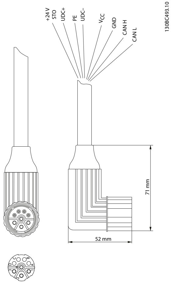
图 4.11 馈电电缆
