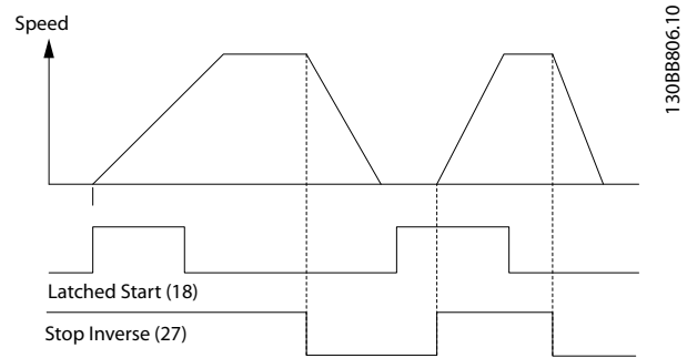
Abbildung 6.3 Puls-Start/Stop invers
