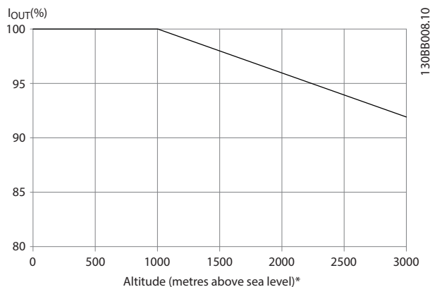
Abbildung 8.10 Höhenabhängige Leistungsreduzierung
