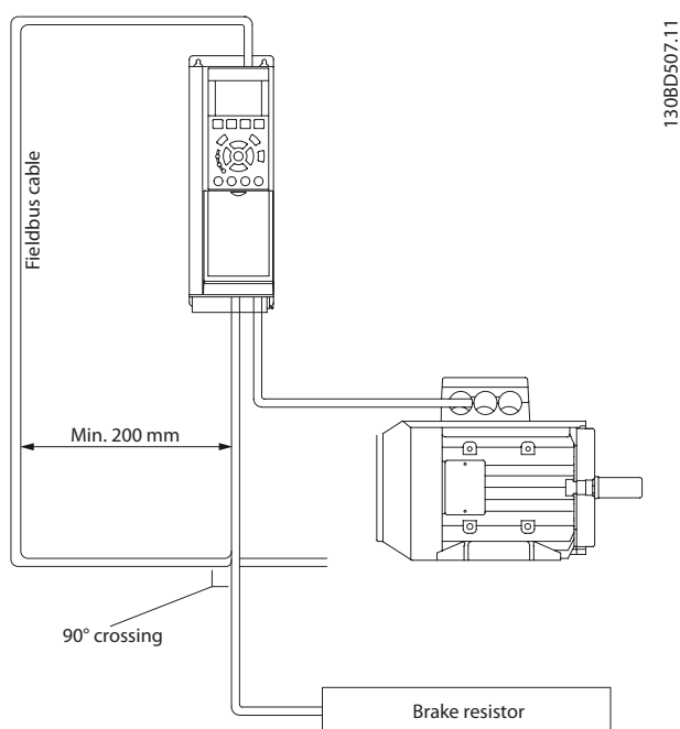
Bild 12.4 Kabeldragning
