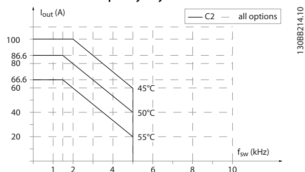
Bild 6.33 Nedstämpling för utström med switchfrekvens och omgivande temperatur för kapslingstyp C2, SFAVM. Obs! Diagrammet är ritat med strömmen som absolut värde och gäller för både hög och normal belastning.
