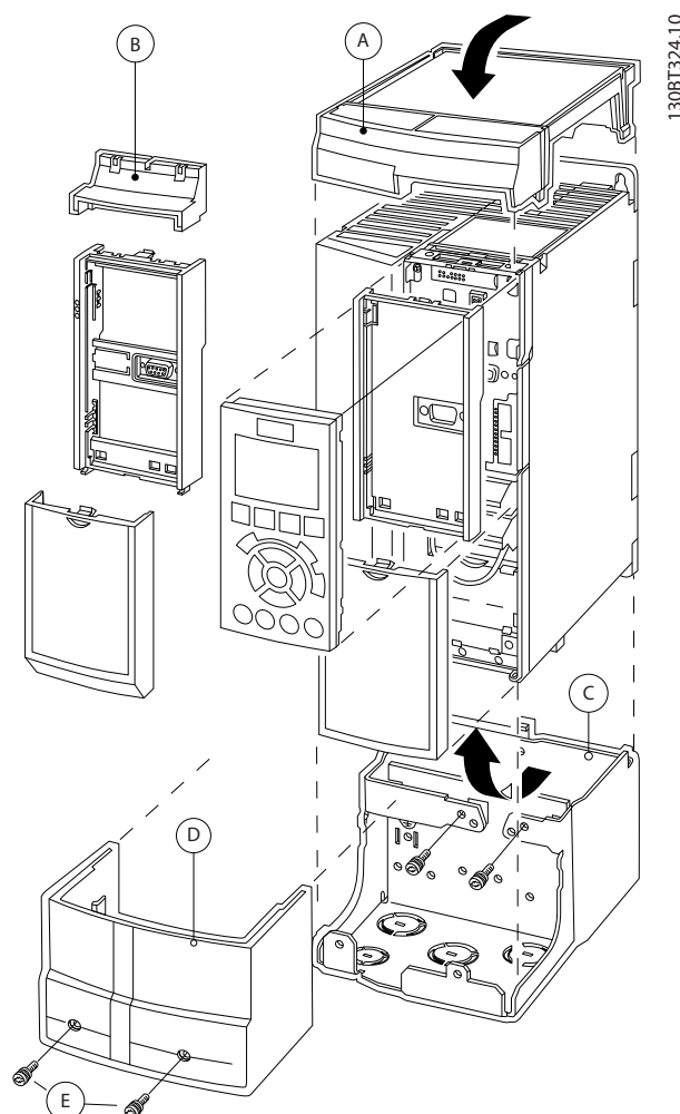
Bild 11.24 Kapslingstyp A3
