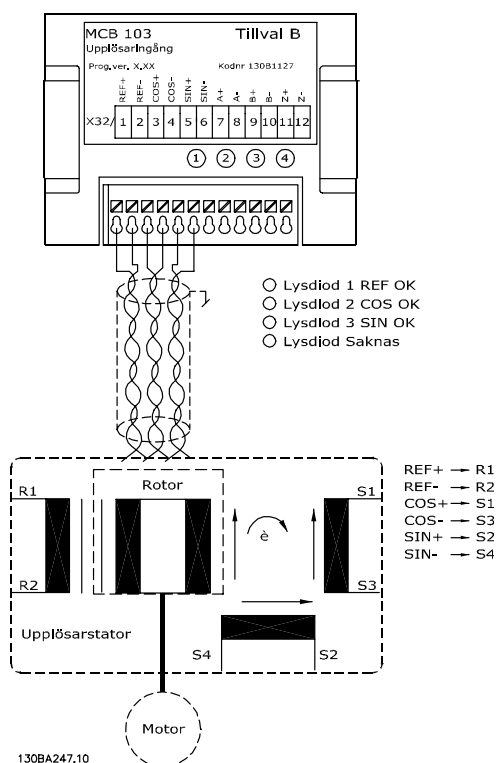
Bild 11.6 MCB 103 resolveringång
