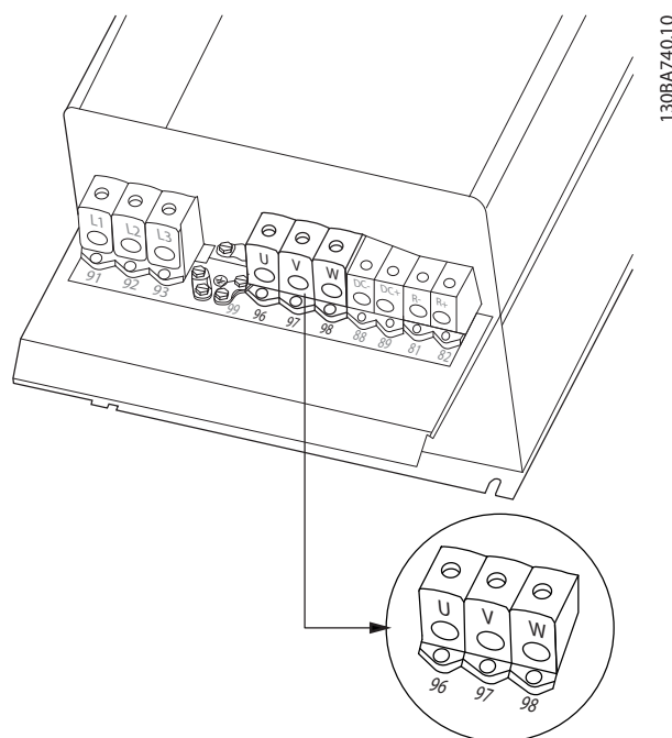
Bild 9.36 Motoranslutning för kapsling C3 och C4
