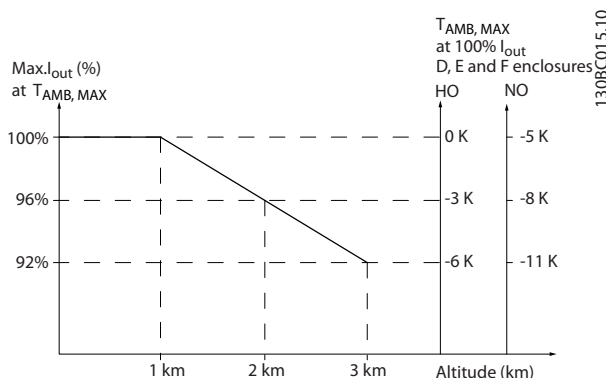
Bild 5.2 Nedstämpling av utström kontra höjd vid T_{AMB, MAX} för kapslingstyp D3h.
