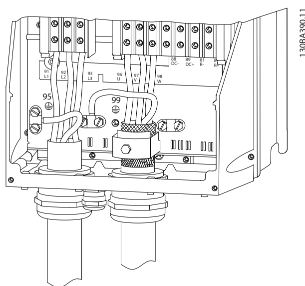
Bild 9.35 Motoranslutning kapsling C1 och C2 (IP 21/ NEMA-typ 1 och IP 55/66/NEMA-typ 12)
