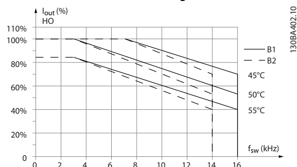
Bild 6.6 Nedstämpling av I_{out} för olika T_{AMB, MAX} för kapslingstyp B1 och B2, vid 60° AVM i läget Hög överbelastning (160 % övermoment)
