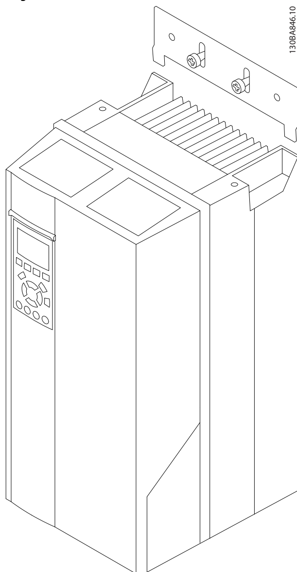
Bild 11.32 Positionering
