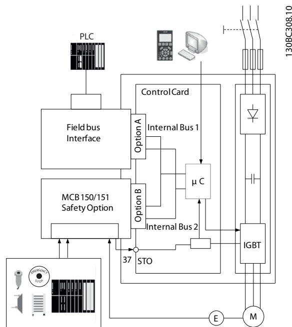
Bild 11.19 Säkert frekvensomformarsystem
