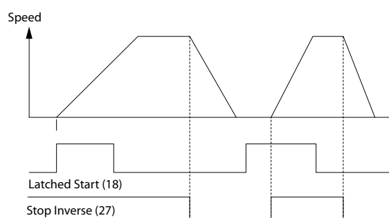
Bild 10.2 Pulsstart/pulsstopp, inverterat
