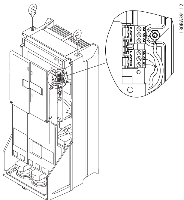
Bild 9.43 Plintar för reläanslutning (Kapslingstyp C1 och C2).
