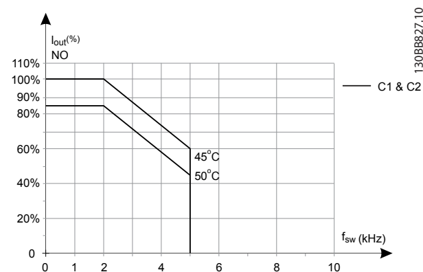
Bild 6.30 Nedstämpling för utström med switchfrekvens och omgivande temperatur för 600 V-frekvensomformare, kapslingstyp C; SFAVM, NÖ
