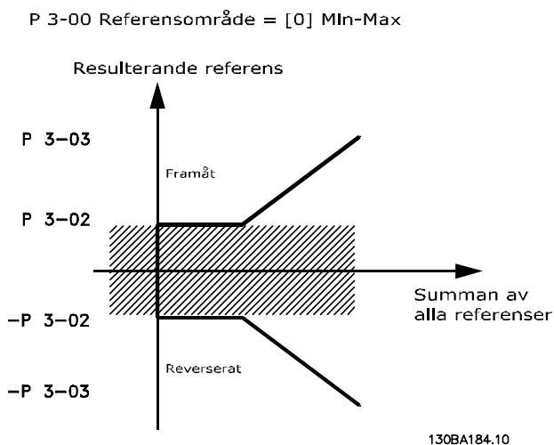
Bild 3.14 Samband mellan resulterande referens och summan av alla referenser
