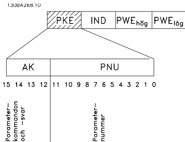
Bild 12.10 PKE-fält
