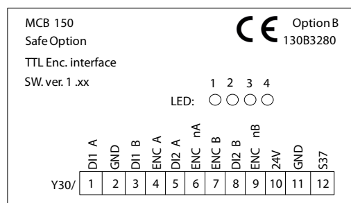
Bild 11.20 MCB 150
