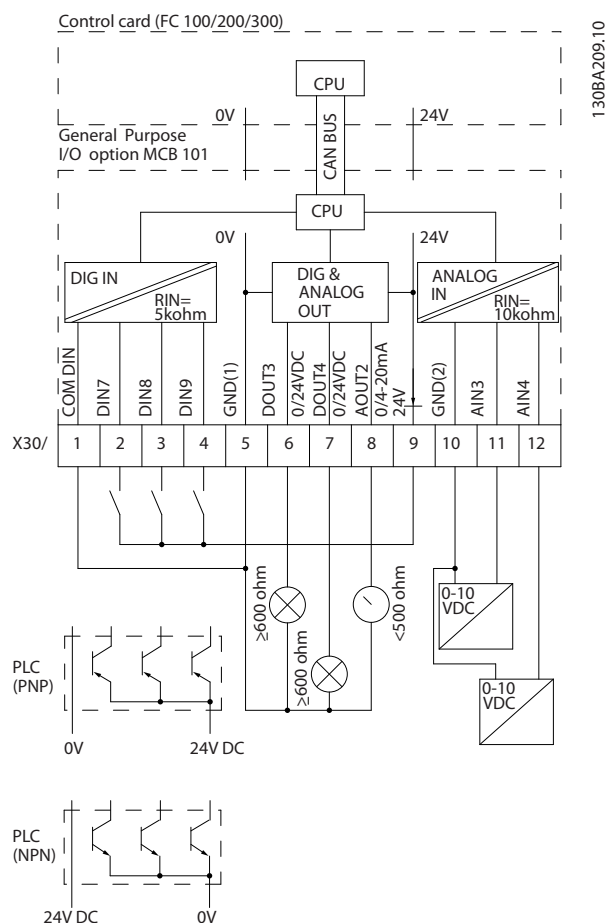
Bild 11.2 Kopplingsschema
