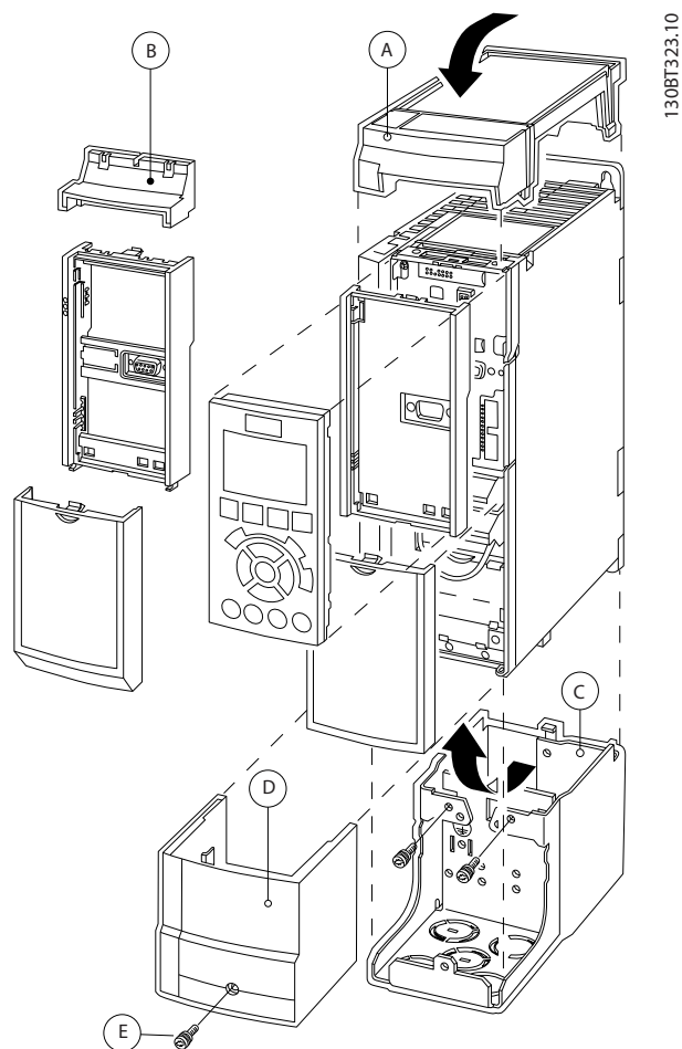
Bild 11.23 Kapslingstyp A2
