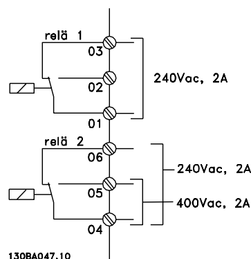
Bild 9.41 Reläutgångarna 1 och 2
