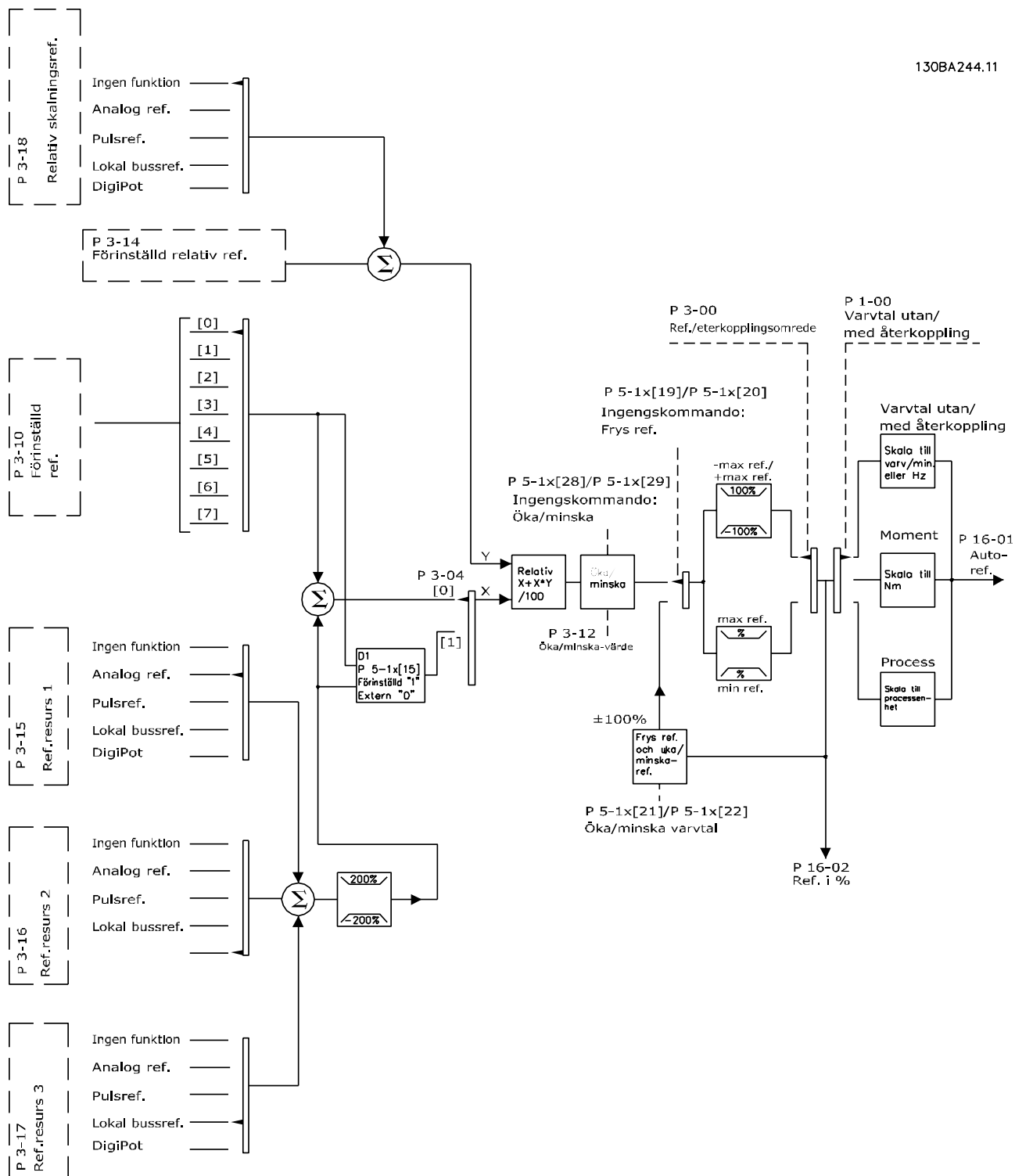
Bild 3.13 Extern referens
