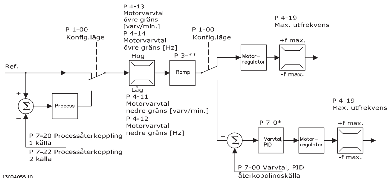
Bild 3.6 Styrstruktur i VVC plus -konfigurationer med och utan återkoppling
