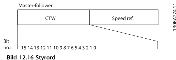
Bild 12.16 Styrord
