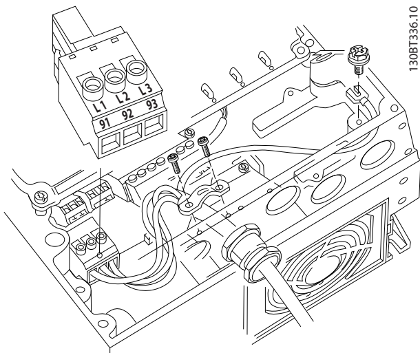
Bild 9.21 Anslutning till nät och jordning utan frångiljare
