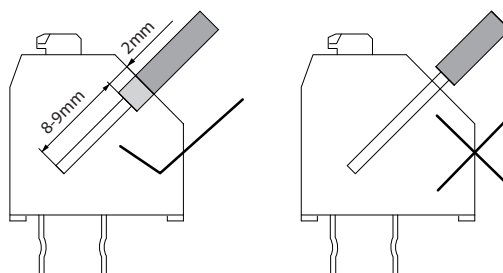
Bild 11.11 Korrekt ledningsdragnig
