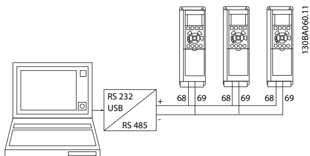
Bild 12.2 Parallellkopplingar
