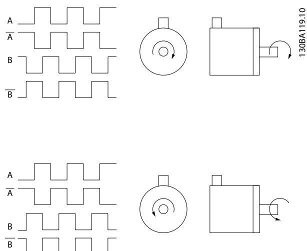
Bild 11.5 Rotationsriktning
