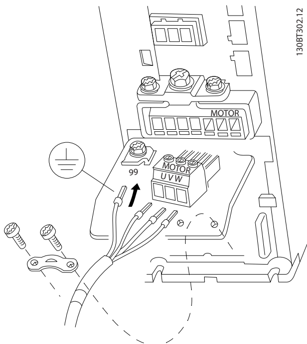
Bild 9.30 Motoranslutning för kapsling A1, A2 och A3
