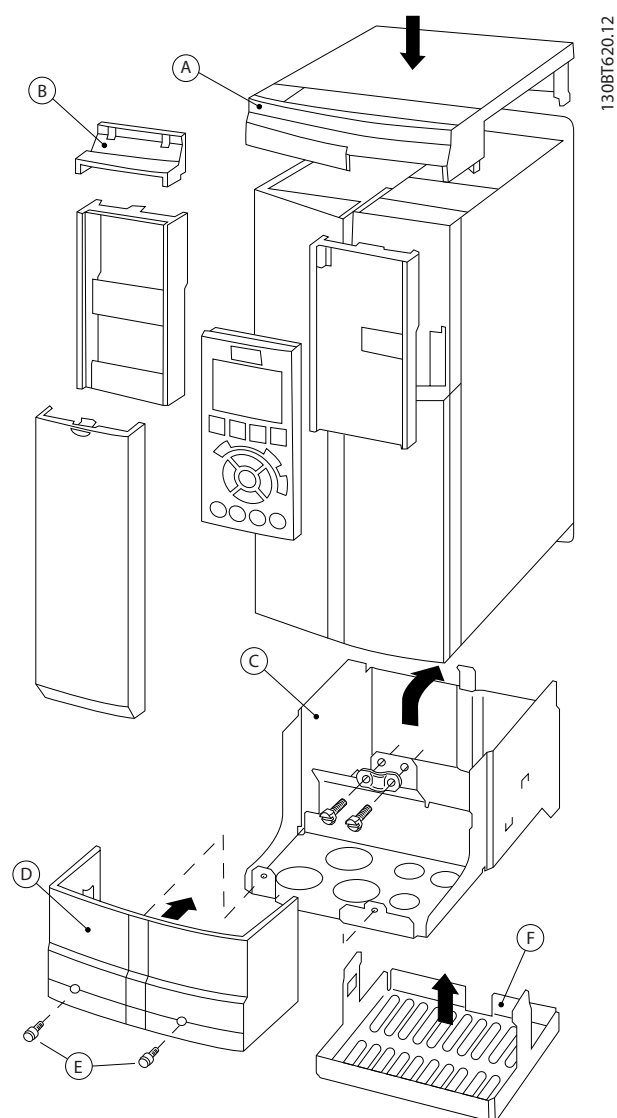
Bild 11.25 Kapslingstyp B3
