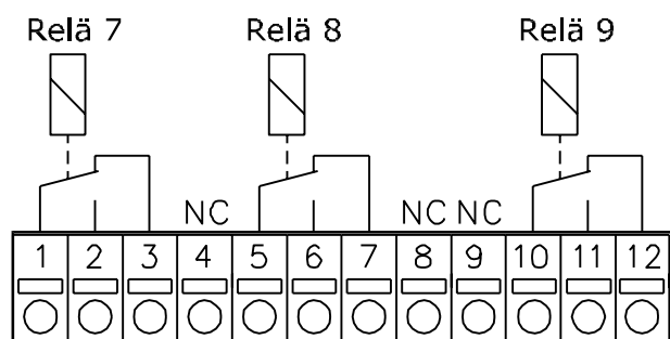
Bild 11.10 Reläer
