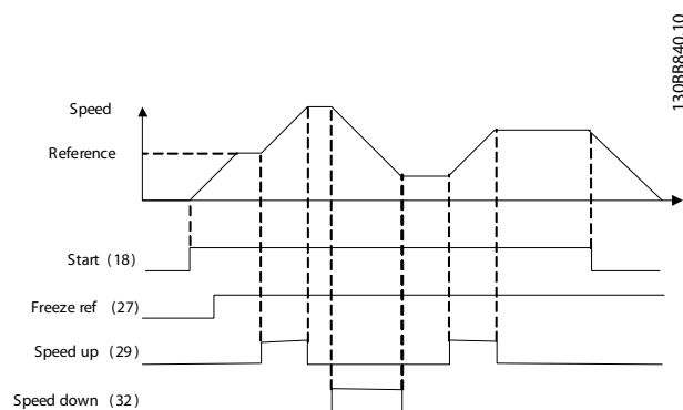
Bild 10.3 Öka/minska varvtal
