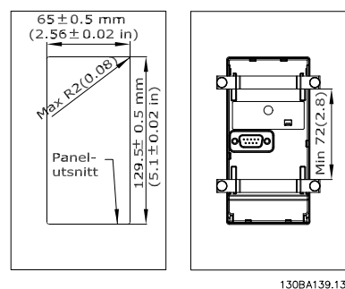
Bild 11.29 Dimensioner
