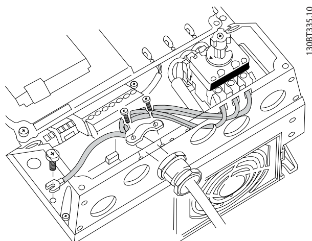
Bild 9.22 Anslutning till nät och jordning med frångiljare
