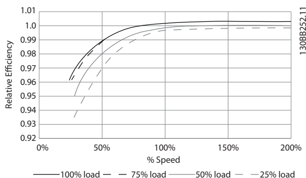
Bild 6.35 Typiska verkningsgradskurvor
