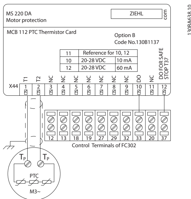
Bild 11.15 Installation av MCB 112
