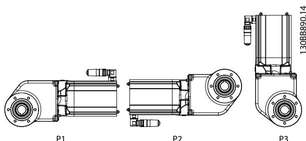
Bild 4.8 OneGearDrive
