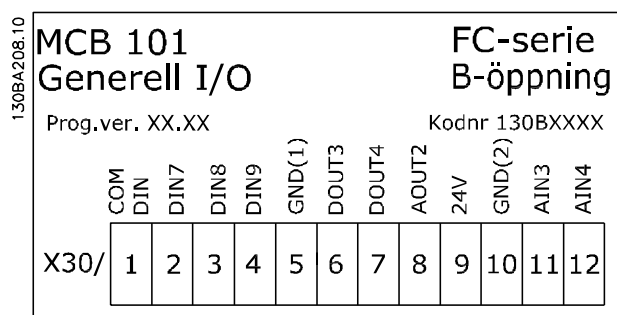
Bild 11.1 Tillvalet MCB 101
