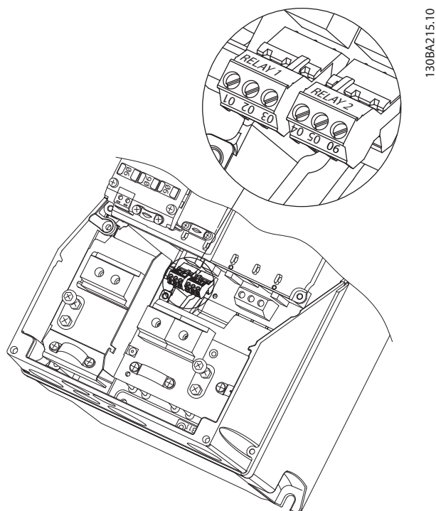
Bild 9.44 Plintar för reläanslutning (Kapslingstyp A5, B1 och B2).
