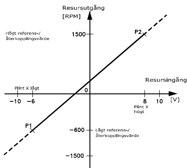
Bild 3.18 Skalning av referensutgång
