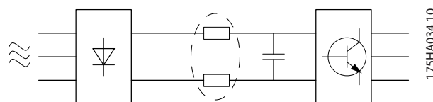
Bild 5.4 Mellankretsspolar
