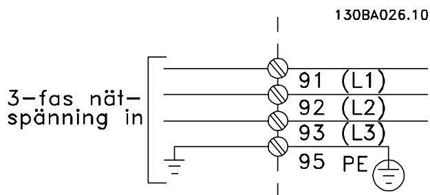
Bild 9.16 Nätanslutning
