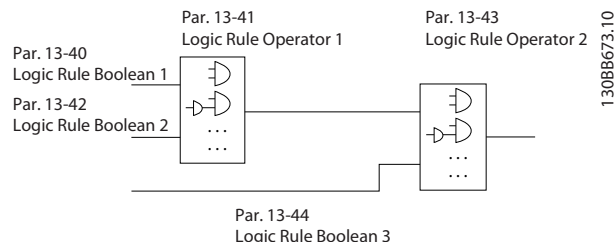
Bild 4.7 Logiska regler
