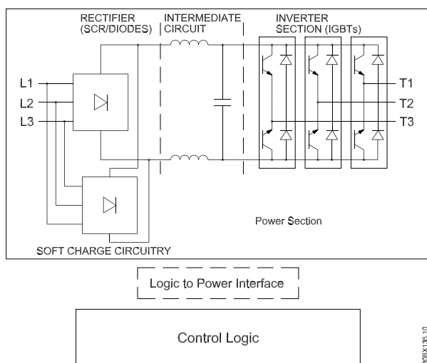
Bild 3.1 Intern styrlogik
