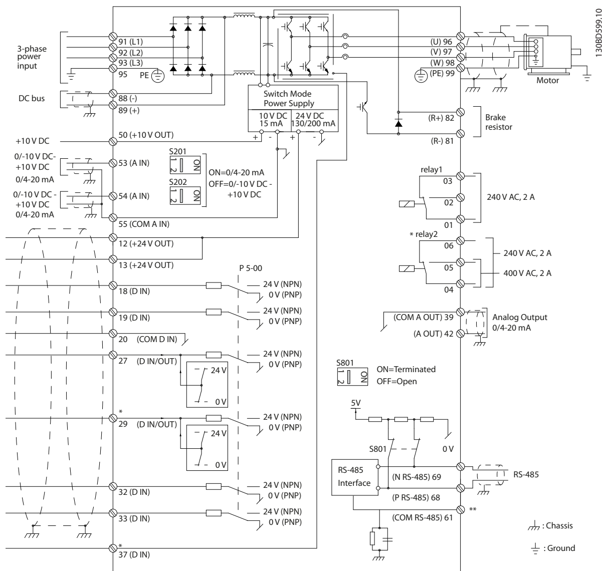
Bild 3.2 Grundläggande kopplingsschema
