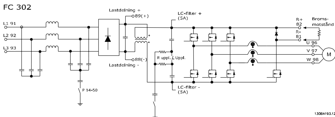
Bild 3.5 Styrprincip FC 302
