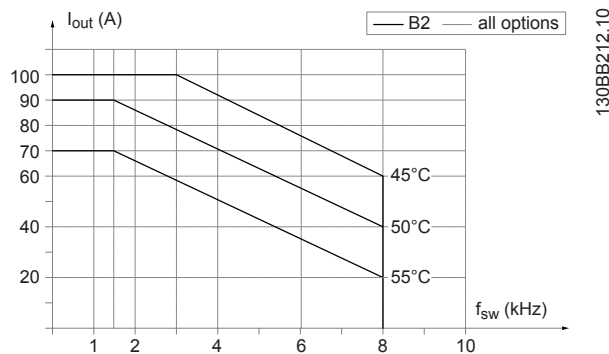
Bild 6.19 Nedstämpling för utström med switchfrekvens och omgivande temperatur för kapslingstyp B2 och B4, SFAVM. Obs! Diagrammet är ritat med strömmen som absolut värde och gäller för både hög och normal belastning.
