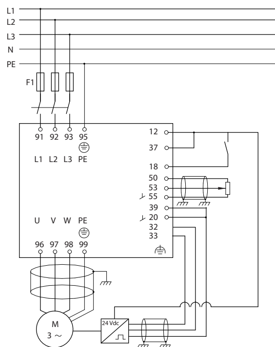
Bild 10.7 Exempel – varvtalsregleringsanslutningar
