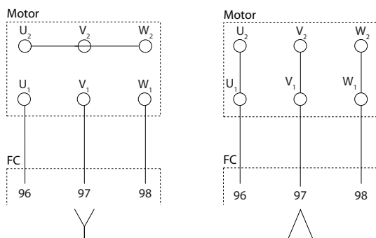
Bild 9.29 Y/D-anslutningar
