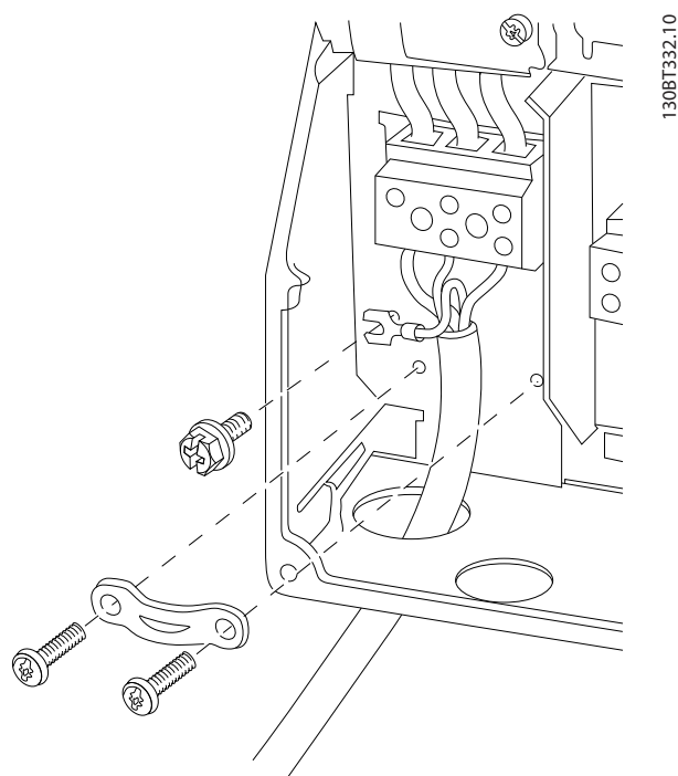
Bild 9.23 Nätanslutning kapsling B1 och B2
