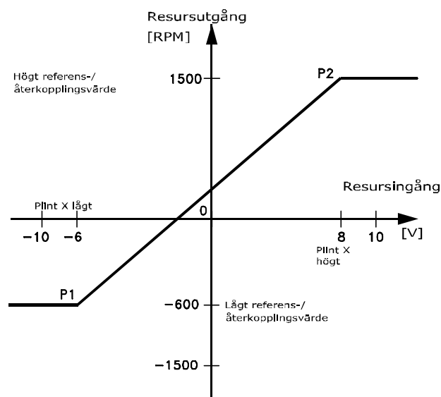
Bild 3.17 Skalning av analog referens och återkoppling och pulsreferens och pulsåterkoppling
