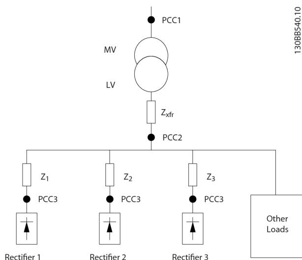
Bild 5.5 Litet distributionssystem
