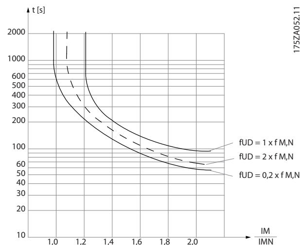
Illustration 3.11 ETR-funktioner
