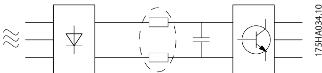
Illustration 3.24 Mellemkredsspoler
