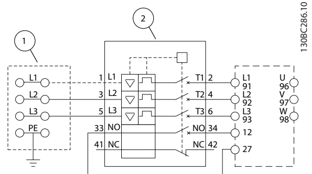
Illustration 3.4 Kun stort apparat: Afbryder og netafbryder
