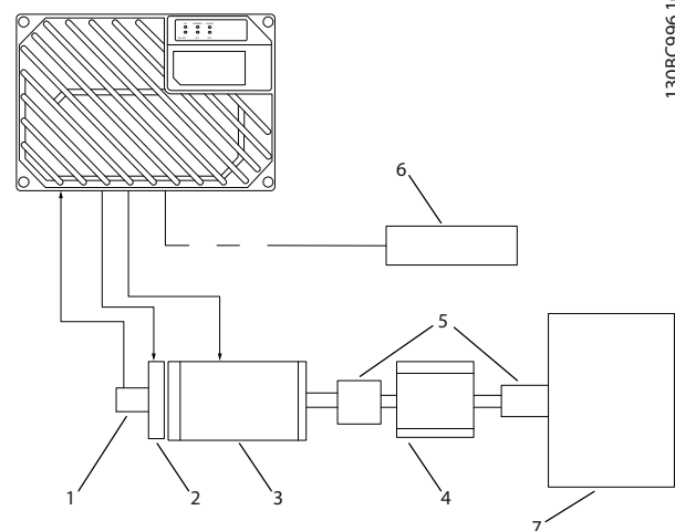
Illustration 4.7 Grundlæggende opsætning for hastighedsstyring med lukket sløjfe
