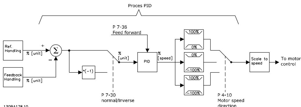
Illustration 4.9 PID-processtyringsdiagram
