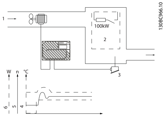
Illustration 4.10 PID-processtyring i ventilationssystem
