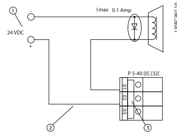
Illustration 4.21 Mekanisk bremsestyring
