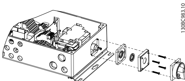
Illustration 3.10 Placering af afbryder, netforsyningside, stort apparat
