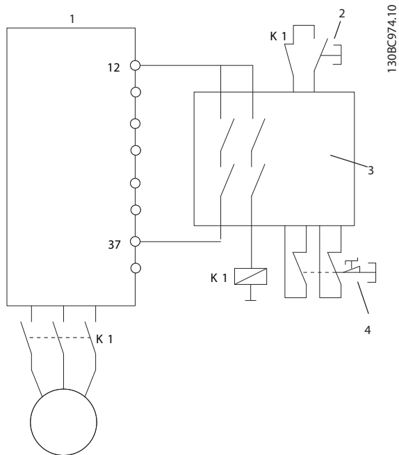
Illustration 4.27 STO-kategori 4 eksempel
