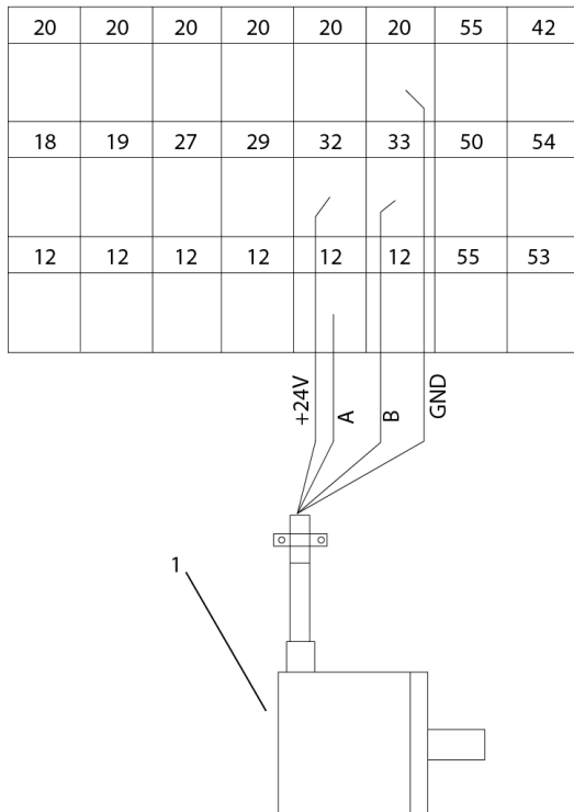
Illustration 4.5 Encoderforbindelse til frekvensomformeren
