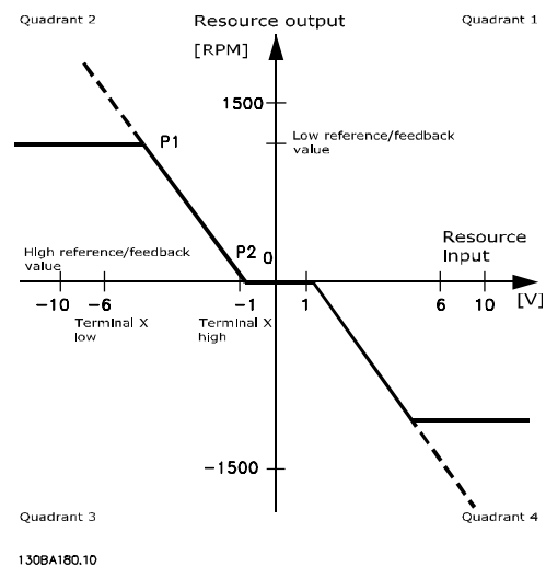
Illustration 2.16 Reversér dødbånd
