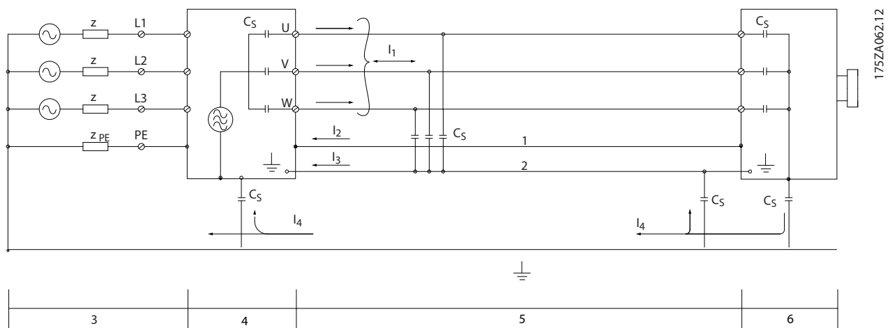
Illustration 2.8 Eksempel - Lækstrøm
