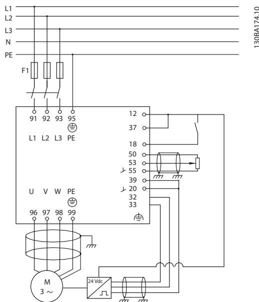
Illustration 4.8 Eksempel - hastighedsstyringstilslutninger
