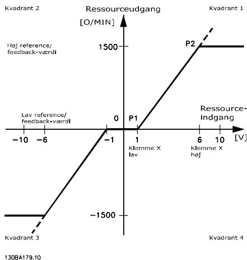
Illustration 2.15 Dødbånd
