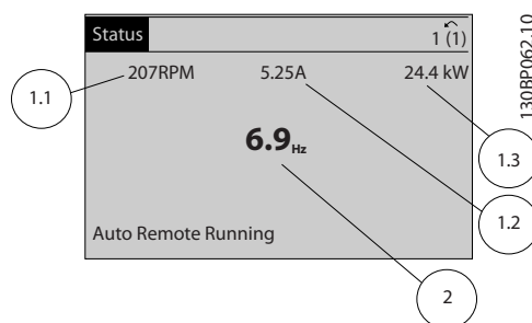
Εικόνα 4.3 Οθόνη κατάστασης II - Παράδειγμα
