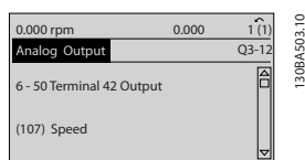
Εικόνα 5.8 Βήμα 7: Χρησιμοποιήστε τα πλήκτρα πλοήγησης πάνω/κάτω για να επιλέξετε μεταξύ διαφορετικών επιλογών. Πατήστε [OK].
