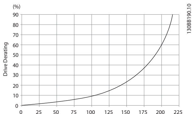
Εικόνα 3.36 Υποβιβασμός ισχύος περιβλήματος F1, F2, F3, F4 έναντι Μεταβολής της πίεσης Ροή αέρα μετατροπέα συχνότητας: 580 cfm (985 m 3 /h)
