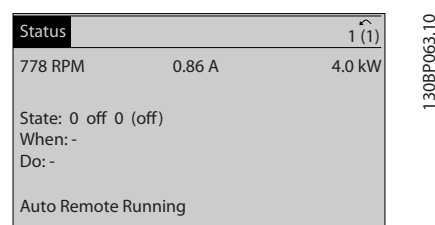
Εικόνα 4.4 Οθόνη κατάστασης III - Παράδειγμα
