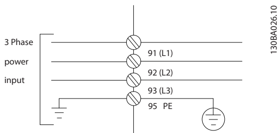
Εικόνα 3.50 Συνδέσεις καλωδίου ρεύματος
