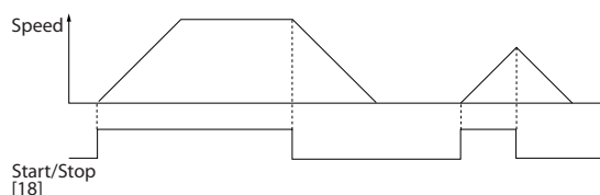
Εικόνα 3.83 Καλωδίωση εκκίνησης/διακοπής
