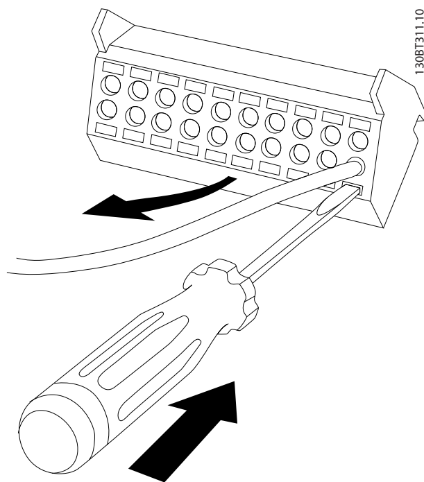
Εικόνα 3.75 Αφαίρεση καλωδίου
