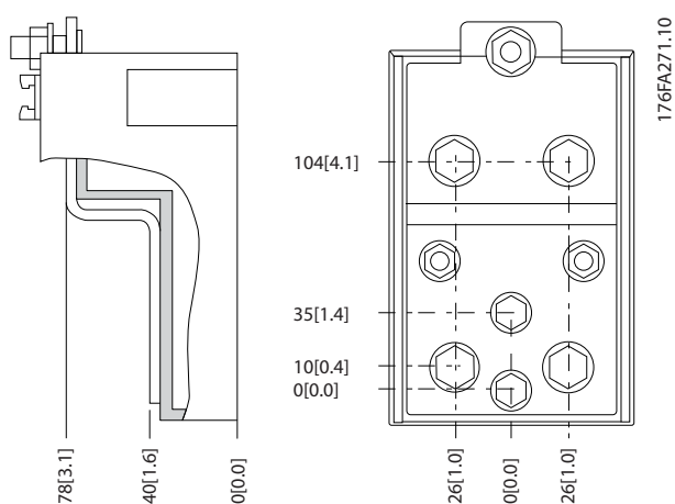
Εικόνα 3.26 Λεπτομέρεια ακροδέκτη
