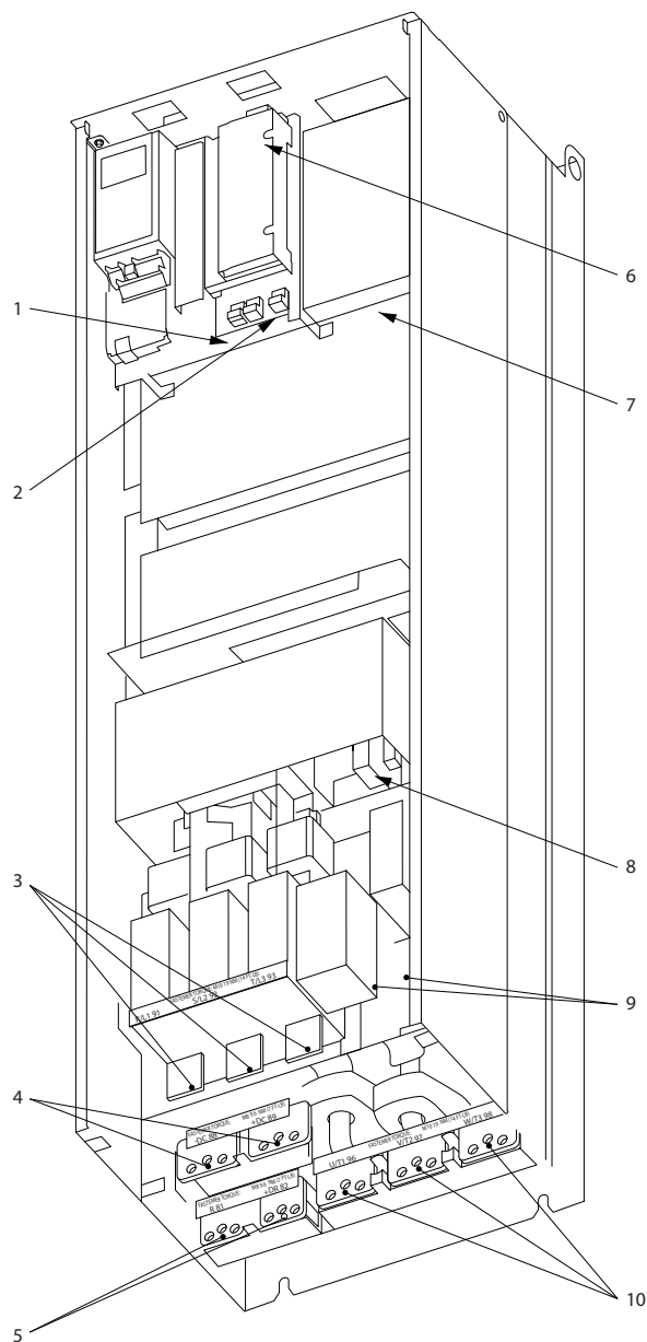
Εικόνα 3.55 Compact IP00 (Πλαίσιο) με αποξεύκτη, ασφάλεια και φίλτρο RFI, Τύπος περιβλήματος D4
