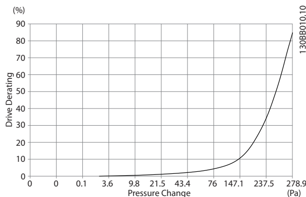
Εικόνα 3.34 Υποβιβασμός ισχύος περιβλήματος E έναντι Μεταβολής Πίεσης (Μικρός ανεμιστήρας), P315T4 και P450T7 Ροή αέρα μετατροπέα συχνότητας: 650 cfm (1105 m³/h)
