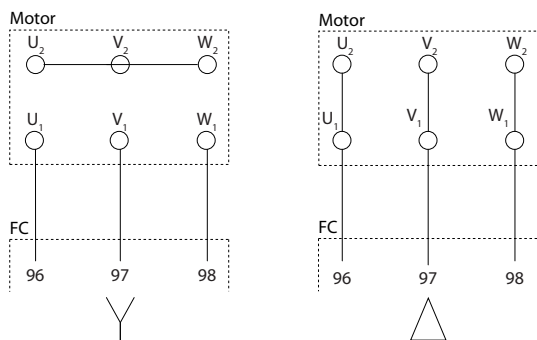
Εικόνα 3.51 Αστεροειδής σύνδεση/σύνδεση δέλτα
