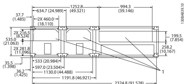
Εικόνα 3.44 Τύπος περιβλήματος F4
