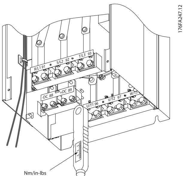
Εικόνα 3.65 Σύσφιξη κοχλίων με ροπόκλειδο
