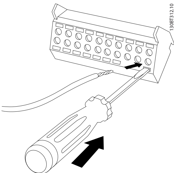
Εικόνα 3.74 Εισαγωγή καλωδίου
