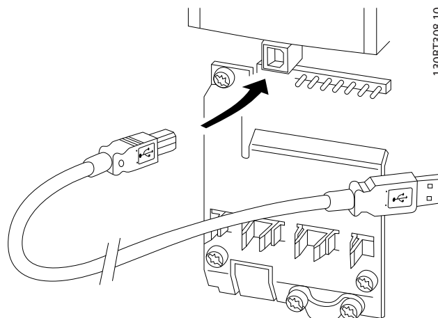
Εικόνα 4.22 Για τις συνδέσεις των καλωδίων σημάτων ελέγχου, ανατρέξτε στην ενότητα Ακροδέκτες σημάτων ελέγχου.
