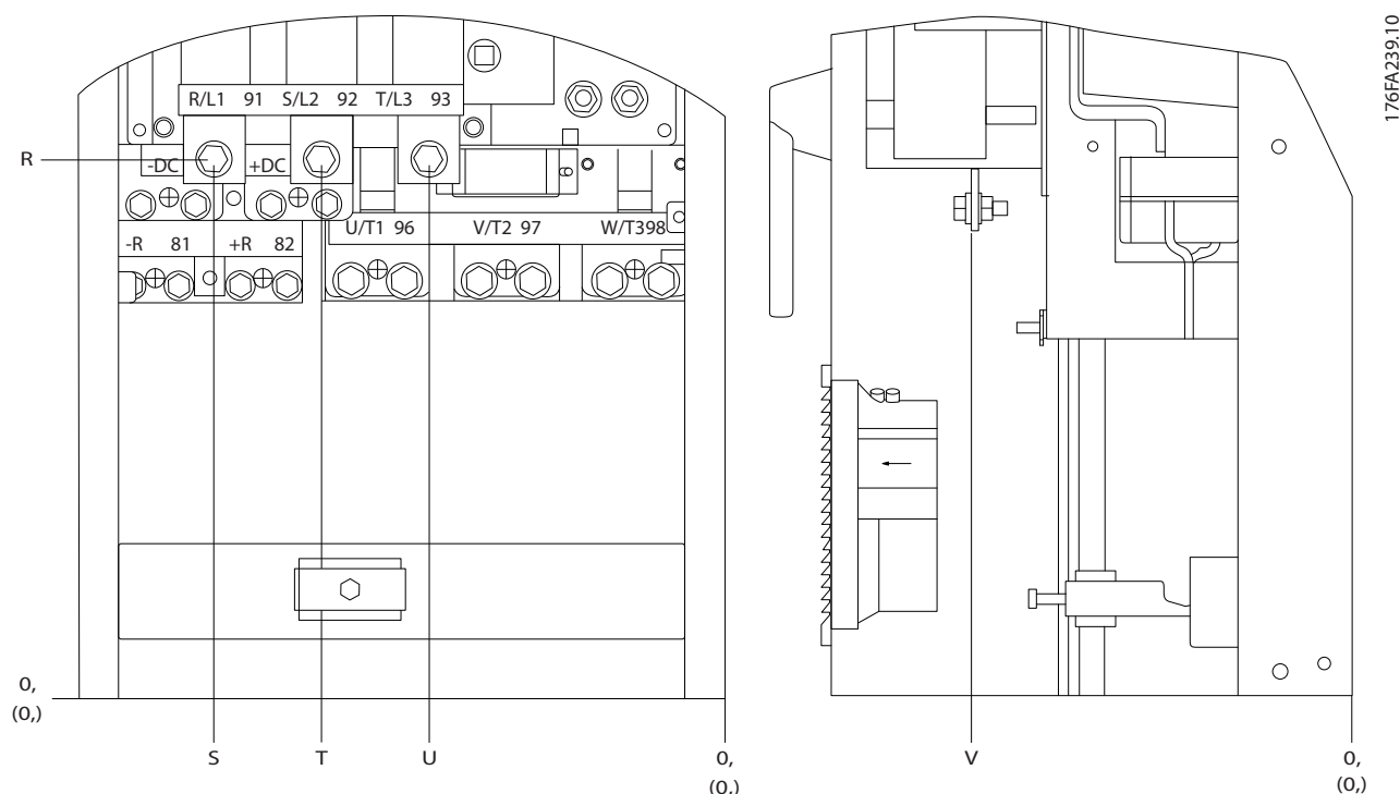
Εικόνα 3.19 Θέση συνδέσεων τροφοδοσίας με διακόπτη απόζευξης,
