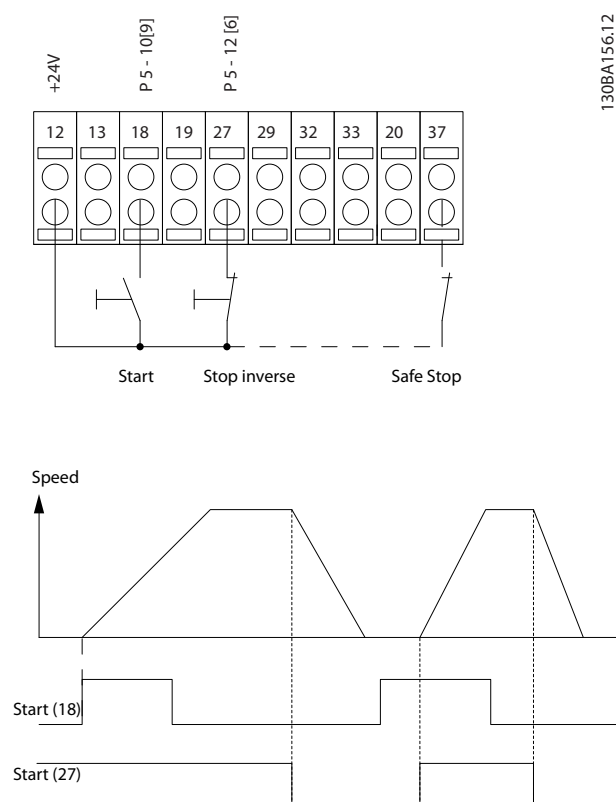
Εικόνα 3.84 Καλωδίωση έναρξης/διακοπής παλμού
