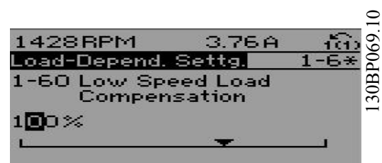
Εικόνα 4.19 Παράδειγμα οθόνης.
