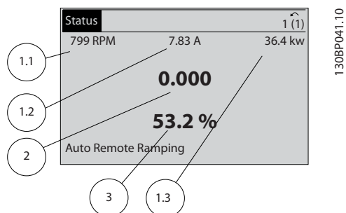
Εικόνα 4.2 Οθόνη κατάστασης I - Παράδειγμα
