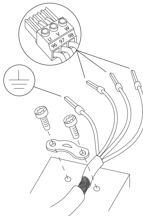
Abbildung 2.4 Motoranschluss
