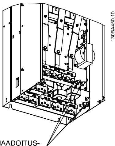
Kuva 3.40: Maadoitusliitinten sijainti IP00, kehyskoot D
