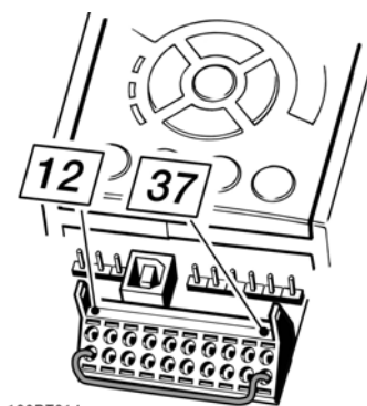
Kuva 2.1: Hyppyjohdin liittimen 37 ja 24 V:n tasavirran välissä
