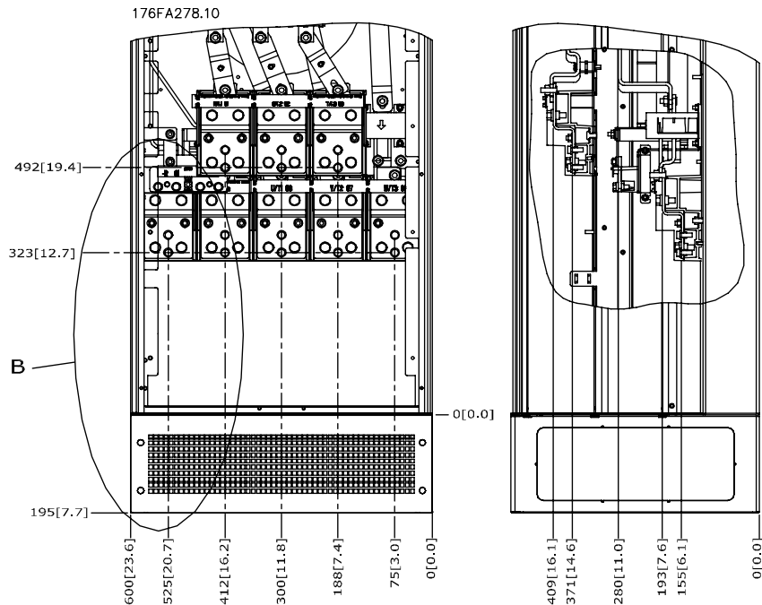
Kuva 3.12: IP21 (NEMA-tyyppi 1) ja IP54 (NEMA-tyyppi 12) kotelon virtakytkeäntöjen paikat
