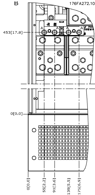
Kuva 3.13: IP21 (NEMA-tyyppi 1) ja IP54 (NEMA-tyyppi 12) kotelon virtakytkeäntöjen paikat (yksityiskohta B)
