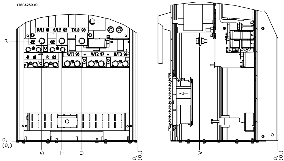
Kuva 3.11: Erotuskytkimellä varustettujen virtakytkentöjen paikka, D1- ja D2-kehyskoko
