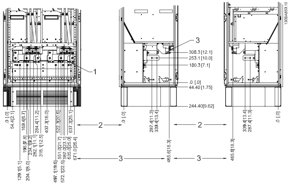
Kuva 3.19: Liitinten paikat - vaihtosuuntauskaappi - F1 ja F3 (näkymä edestä, vasemmalta ja oikealta)
