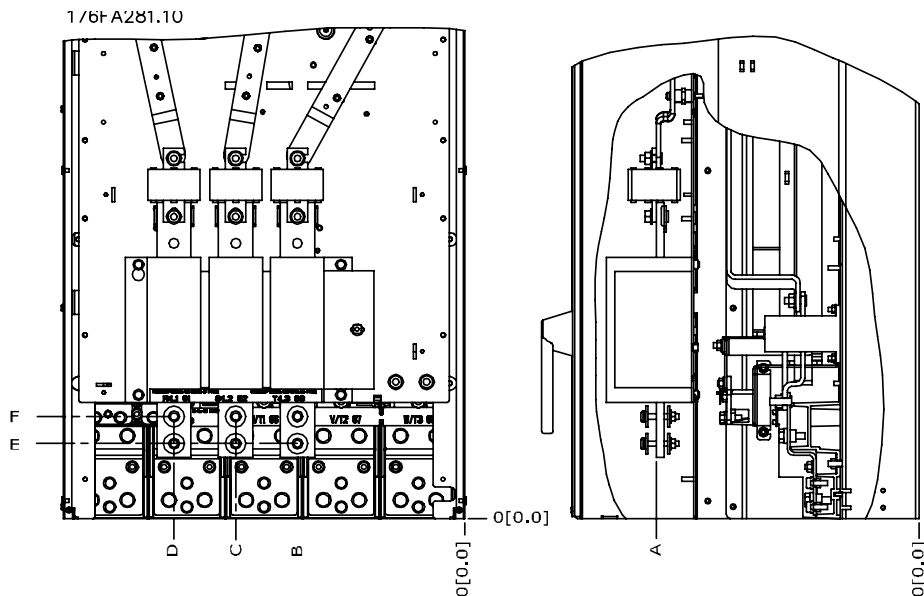
Kuva 3.17: IP00-koteloinnin virtakytkentöjen katkaisinten paikat
