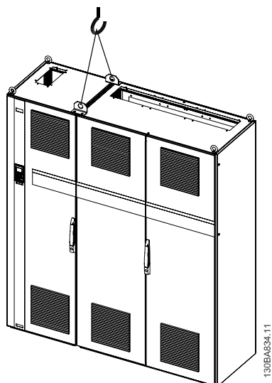
Kuva 3.5: Suositeltava nostotapa, kehyskoko F2.
