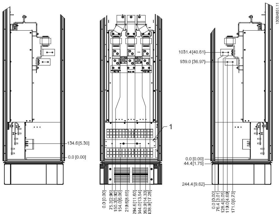
Kuva 3.22: Liitinten paikat - Optiokaappi (näkymä vasemmalta, edestä ja oikealta)
