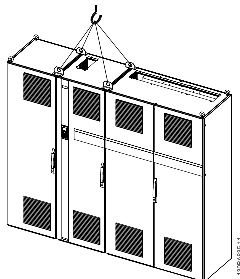
Kuva 3.7: Suositeltava nostotapa, kehyskoko F4.
