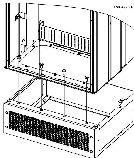
Kuva 3.35: Taajuusmuuttajan asennus jalustalle
