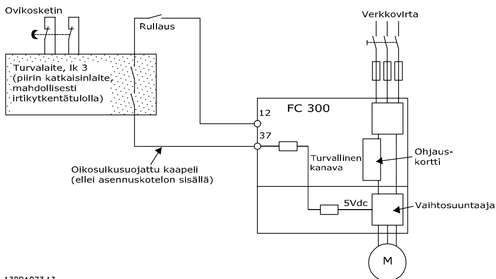
130BA073.13 Kuva 2.2: Kuvaus asennuksen olennaisista ominaisuuksista pysäytysluokan 0 (EN 60204-1) saavuttamiseksi turvallisuusluokan 3 (EN 954-1) mukaisesti.
