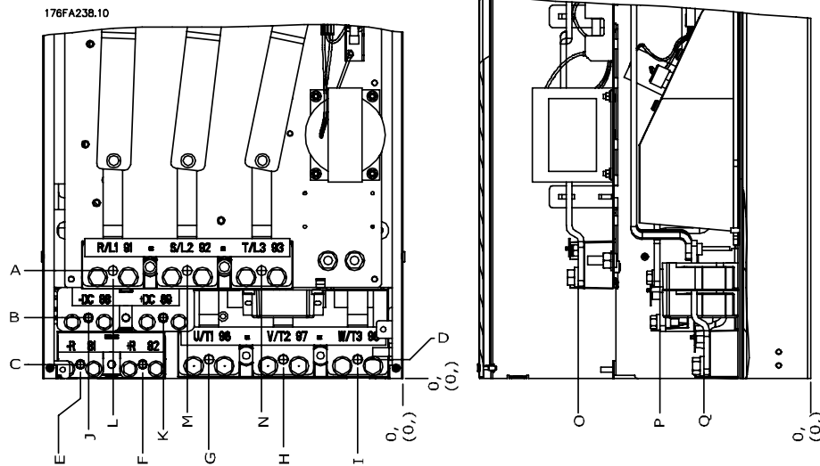
Kuva 3.10: Virtakytkentöjen sijainti, D3- ja D4-kehyskoot
