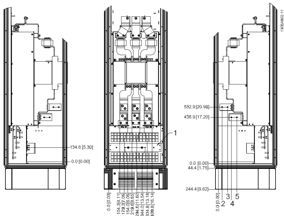
Kuva 3.23: Liitinten paikat - Optiokaappi katkaisimella / muotittiin valetulla kotelokytkimellä (näkymä vasemmalta, edestä ja oikealta)
