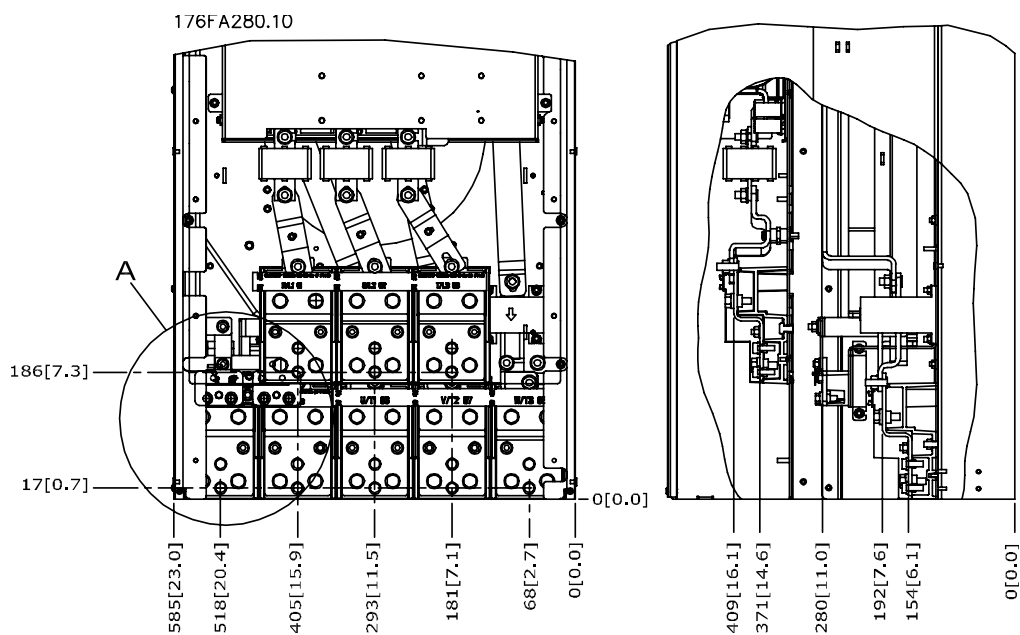
Kuva 3.15: IP00 kotelon virtakytkentöjen paikat
