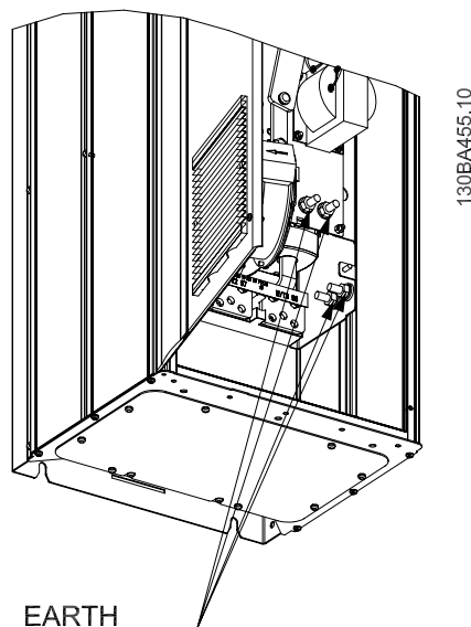
Kuva 3.41: Maadoitusliitinten sijainti, IP21 (NEMA-tyyppi 1) ja IP54 (NEMA-tyyppi 12)
