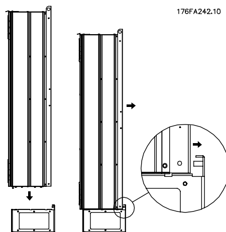
Kuva 3.33: Taajuusmuuttajan asennus jalustalle.
