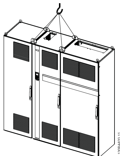
Kuva 3.6: Suositeltava nostotapa, kehyskoko F3.
