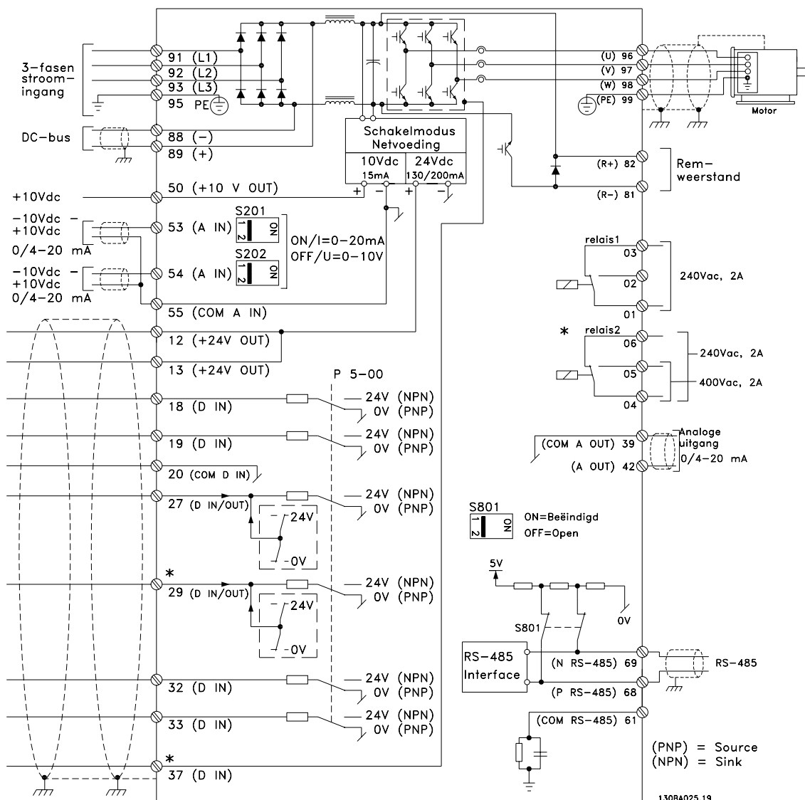
Afbeelding 3.53: Schema met alle elektrische klemmen zonder opties.
