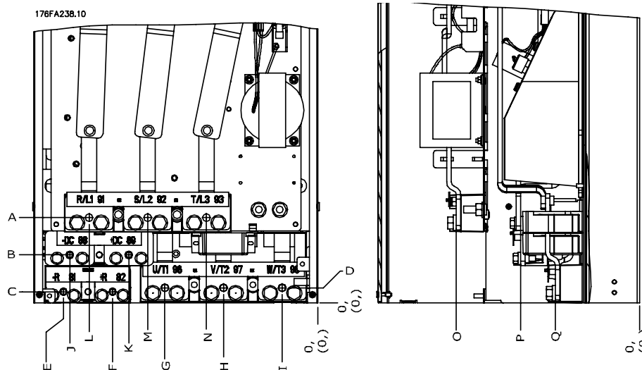
Afbeelding 3.10: Positie van voedingsaansluitingen, framegrootte D3 en D4
