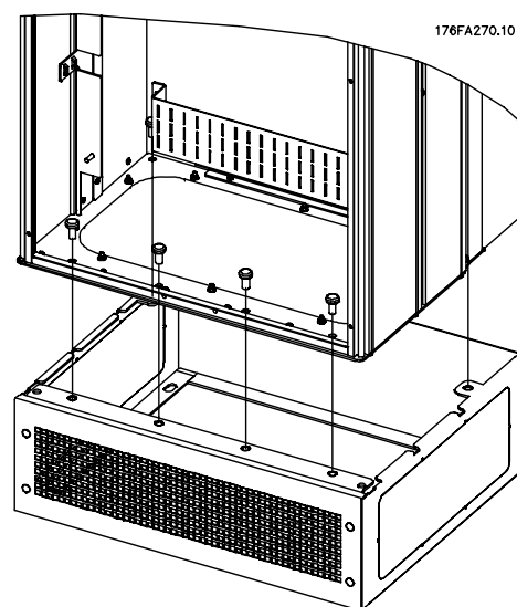
Afbeelding 3.35: De omvormer op de voet bevestigen
