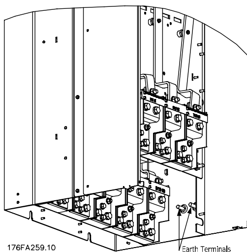
Afbeelding 3.44: Positie van aardklemmen IP 00, ,framegrootte E
