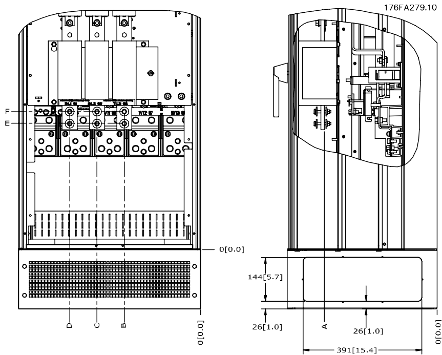
Afbeelding 3.14: Aansluitpositie voedingskabel van werkschakelaar voor IP21 (NEMA type 1) en IP54 (NEMA type 12) behuizingen
