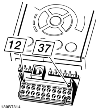
Afbeelding 2.1: Geleiderbrug (jumper) tussen klem 37 en 24 V DC
