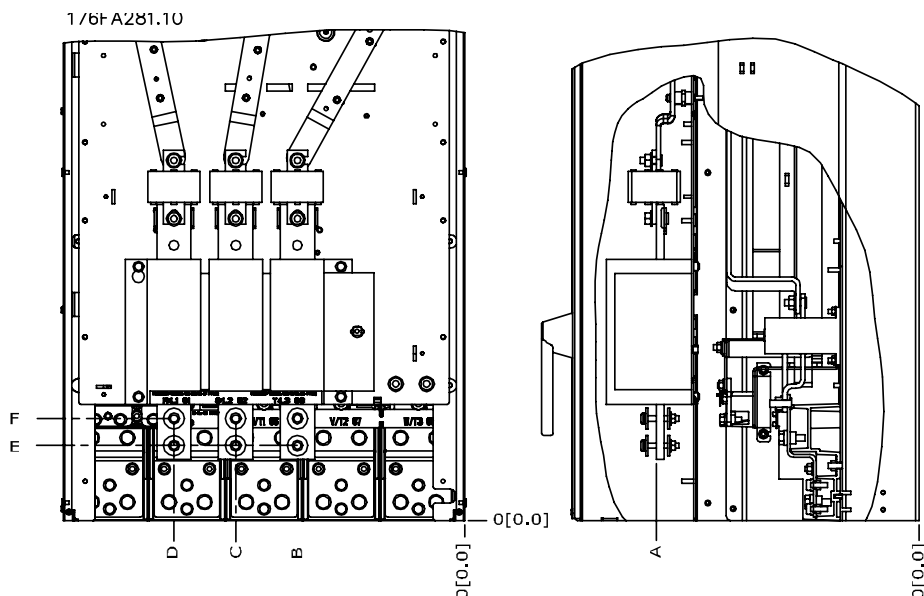
Afbeelding 3.17: Aansluitposities voedingskabel van werkschakelaar voor IP00 behuizing
