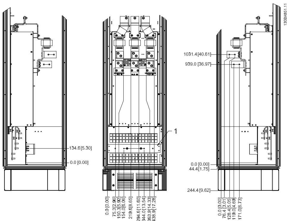
Afbeelding 3.22: Klemposities – optiekast (zijaanzicht links, vooraanzicht en zijaanzicht rechts)
