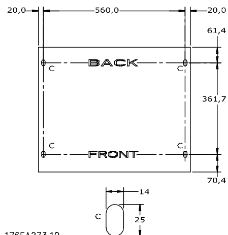
Afbeelding 3.34: Boormal voor bevestigingsgaten in de vloer
