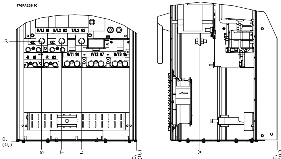
Afbeelding 3.11: Positie van voedingsaansluitingen met werkschakelaar, framegrootte D1 en D2
