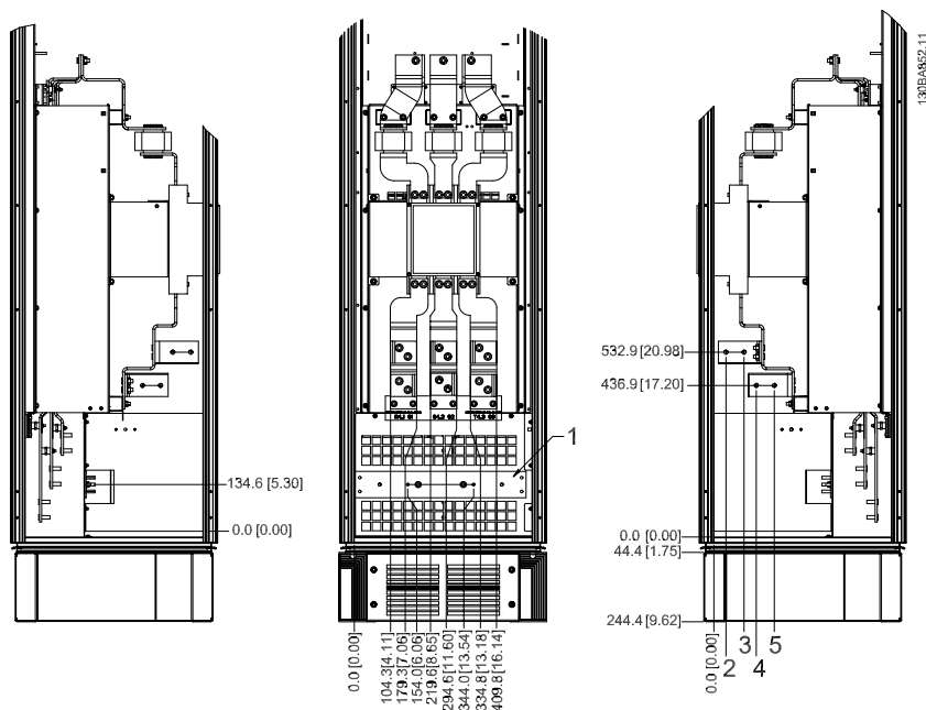
Afbeelding 3.23: Klemposities – optiekast met stroomonderbreker/schakelaar met gegoten behuizing (vooraanzicht, zijaanzicht links en rechts)
