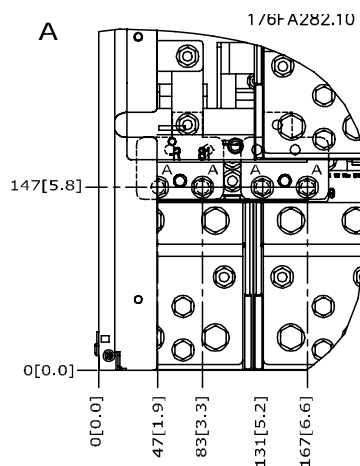
Afbeelding 3.16: Aansluitposities voedingskabels voor IP00 behuizing
