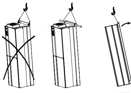
Afbeelding 3.3: Aanbevolen hijsmethode, framegrootte D en E .
