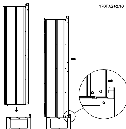
Afbeelding 3.33: De omvormer op de voet bevestigen
