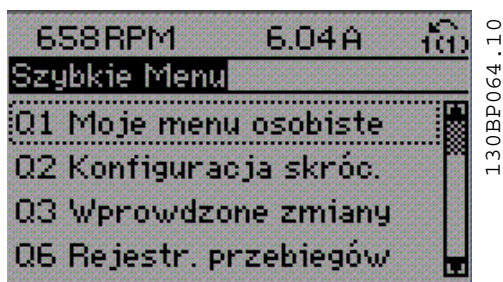
Ilustracja 5.1: Wygląd Szybkiego menu.
