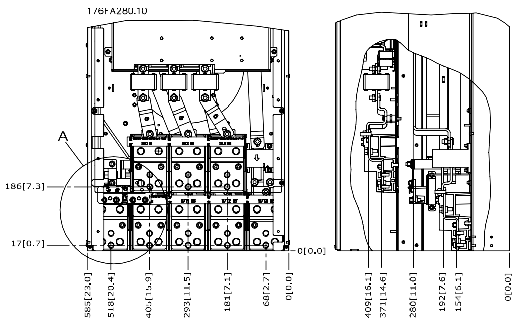
Ilustracja 3.15: Położenie złączy zasilania w obudowie IP00
