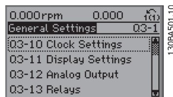
Ilustracja 5.6: Krok 5: Za pomocą przycisków nawigacji góra/dół przewinąć listę do odpowiedniej pozycji, tzn. Q3-12 Wyjścia analogowe . Naciśnąć przycisk [OK].
