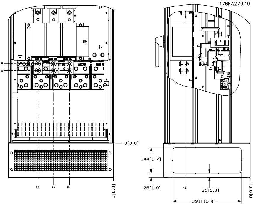
Ilustracja 3.14: Położenie złączy zasilania wyłącznika w obudowie IP21 (NEMA Typ 1) i IP54 (NEMA Typ 12)
