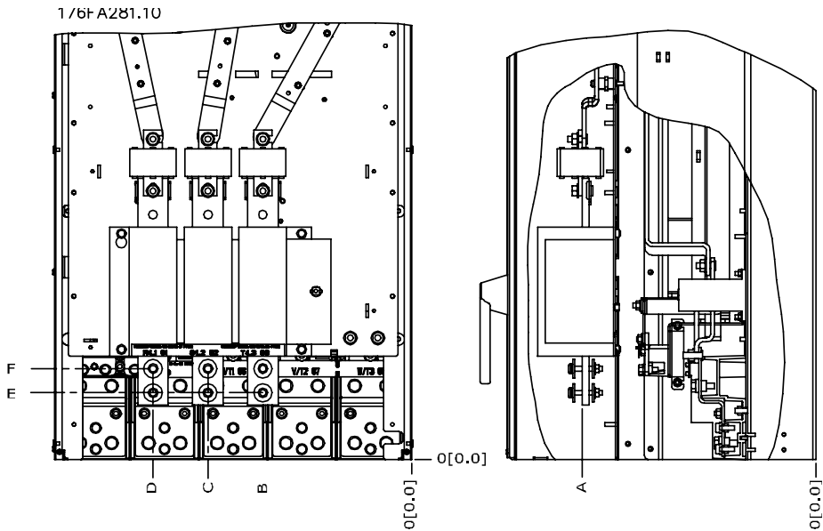
Ilustracja 3.17: Położenie złączy zasilania wyłącznika w obudowie IP00
