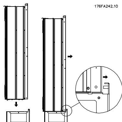
Ilustracja 3.33: Montaż przetwornicy częstotliwości na podstawie.
