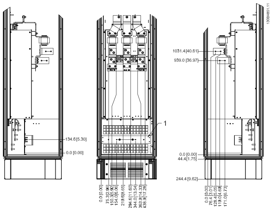
Ilustracja 3.22: Położenie zacisków - szafka opcji (widok od lewej, od przodu i od prawej)
