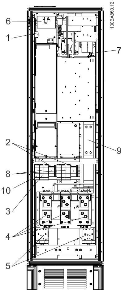
Ilustracja 3.45: Szafka prostownika, rozmiar ramy F1, F2, F3 i F4
