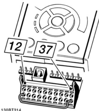
Ilustracja 2.1: Zworka mostkująca między zaciskiem 37 i 24 VDC.
