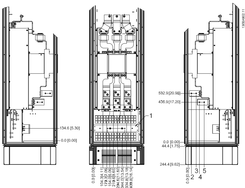
Ilustracja 3.23: Położenie zacisków - szafka opcji z wyłącznikiem/przełącznikiem w obudowie formowanej (widok od lewej, od przodu i od prawej)
