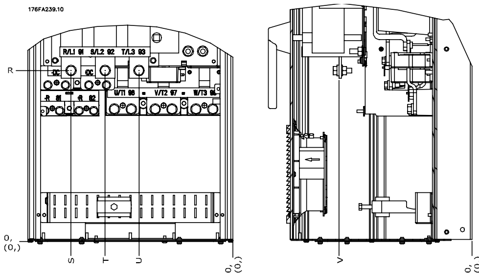
Ilustracja 3.11: Położenie złączy zasilania z przełącznikiem odcinającym, rozmiar ramy D1 i D2
