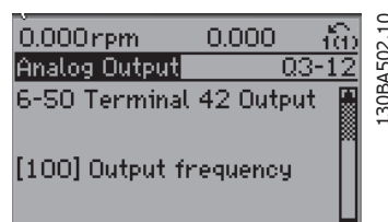
Ilustracja 5.7: Krok 6: Wybrać parametr 6-50 Zacisk 42. Wyjście . Naciśnąć przycisk [OK].
