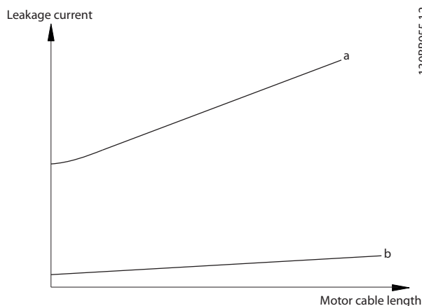
Рисунок 2.31 Влияние длины кабеля и мощности на ток утечки, P_a > P_b
