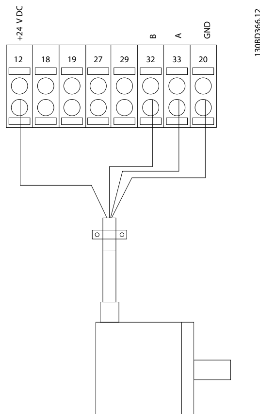
Рисунок 6.2 Энкодер 24 В или 10–30 В
