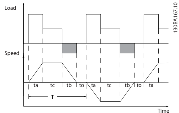
Рисунок 2.35 Типичный цикл торможения
