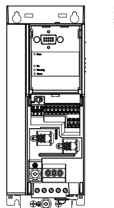
Illustration 7.2 Réglage d'usine du commutateur de terminaison
