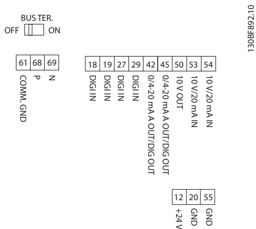
Illustration 5.17 Bornes de commande
