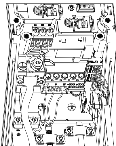
Illustration 5.11 Boîtiers IP54 de tailles I2, I3, I4
