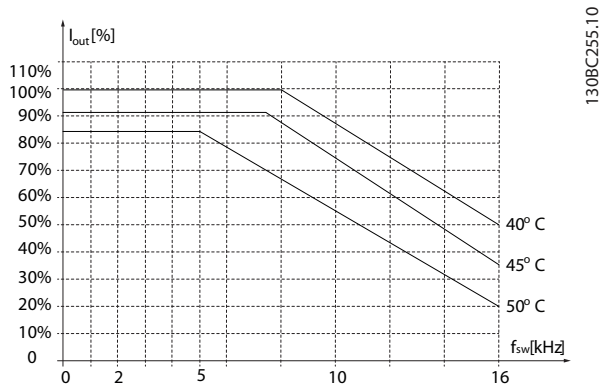
Illustration 3.45 0,75-4,0 kW (1,0-5,4 HP), 400 V, boîtier de taille I2, IP54
