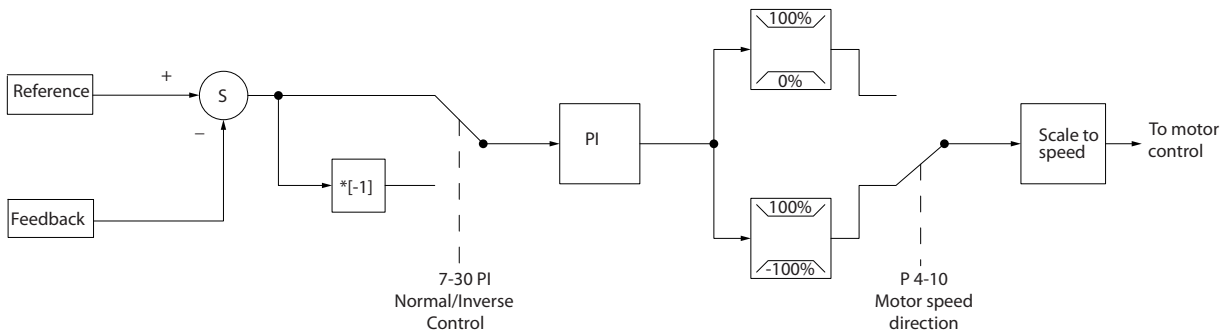
Illustration 3.19 Structure de contrôle en boucle fermée
