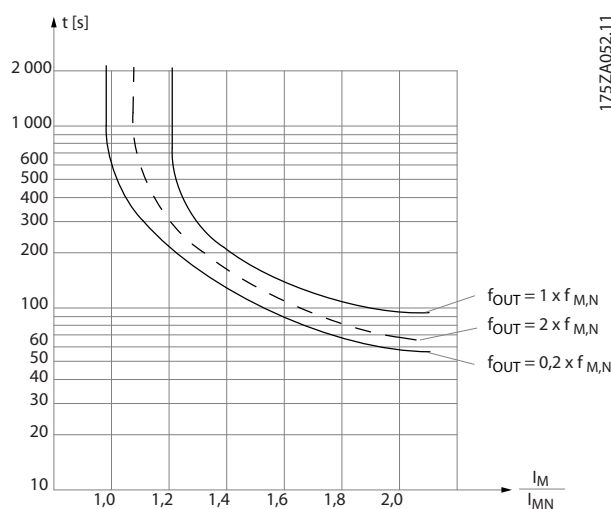
Illustration 3.56 Courbe caractéristique de la protection thermique du moteur
