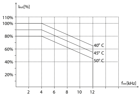
Illustration 3.33 30-37 kW (40-50 HP), 400 V, boîtier de taille H6, IP20
