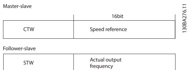
Illustration 7.17 Fréquence de sortie réelle (MAV)
