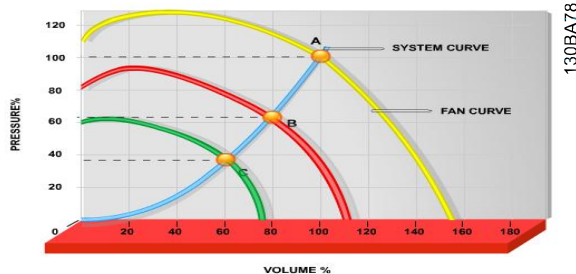
Illustration 3.1 Courbes de ventilateur (A, B et C) pour des volumes de ventilation réduits
