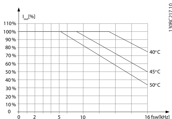
Illustration 3.22 0,25-0,75 kW (0,34-1,0 HP), 200 V, boîtier de taille H1, IP20
