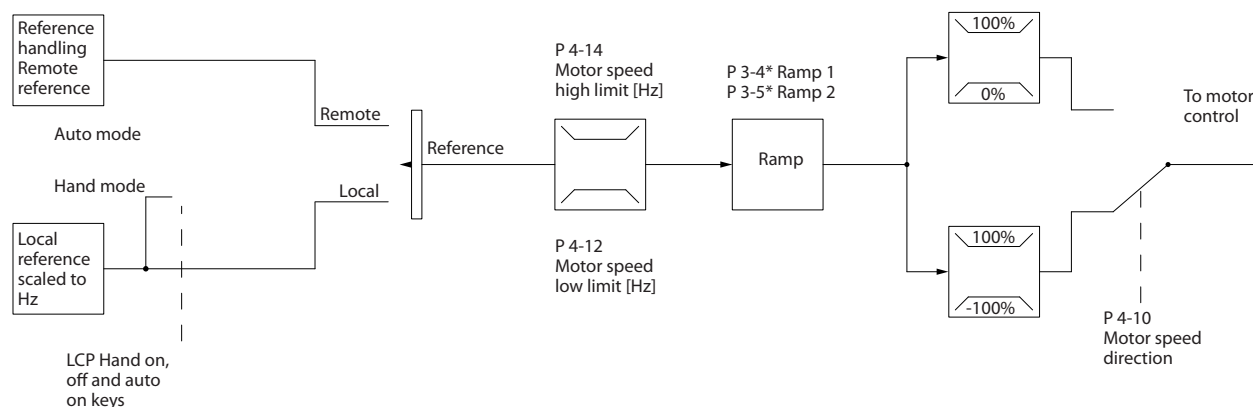
Illustration 3.17 Structure en boucle ouverte
