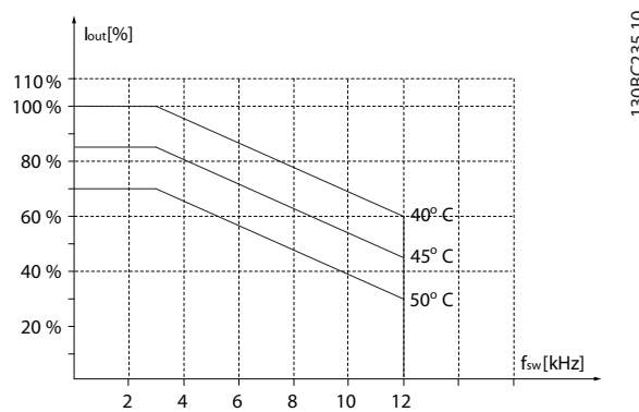
Illustration 3.40 90 kW (120 HP), 400 V, boîtier de taille H8, IP20
