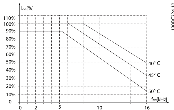
Illustration 3.29 11-15 kW (15-20 HP), 400 V, boîtier de taille H4, IP20
