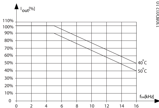
Illustration 3.47 11-18,5 kW (15-25 HP), 400 V, boîtier de taille I4, IP54
