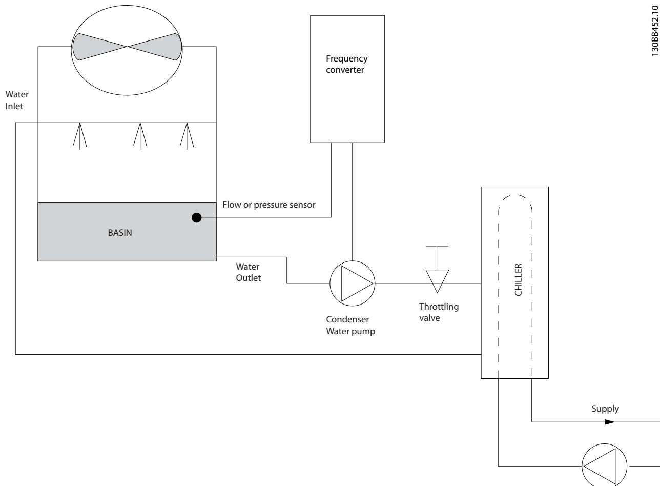
Illustration 3.14 Pompes de condenseur
