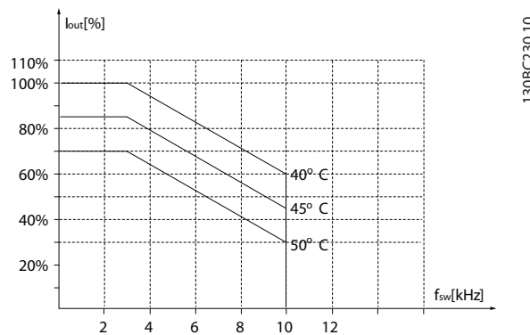
Illustration 3.35 22-30 kW (30-40 HP), 600 V, boîtier de taille H6, IP20
