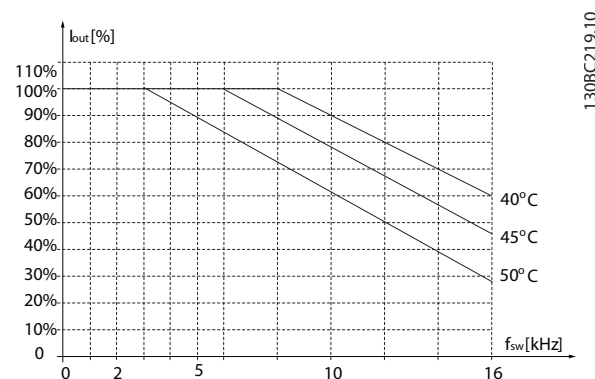
Illustration 3.24 2,2 kW (3,0 HP), 200 V, boîtier de taille H2, IP20
