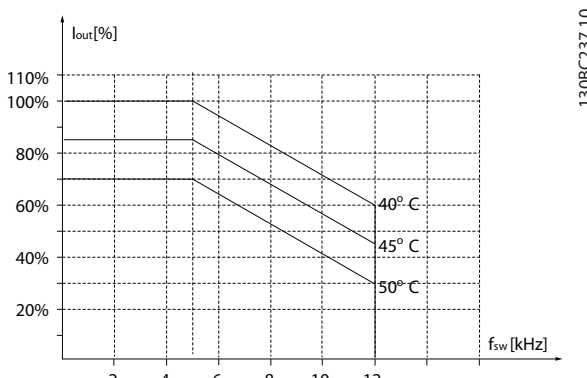
Illustration 3.42 2,2-3 kW (3,0-4,0 HP), 600 V, boîtier de taille H9, IP20
