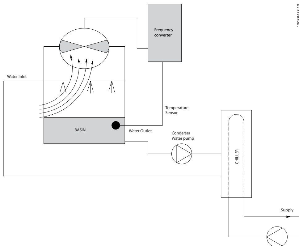
Illustration 3.13 Ventilateur de tour de refroidissement
