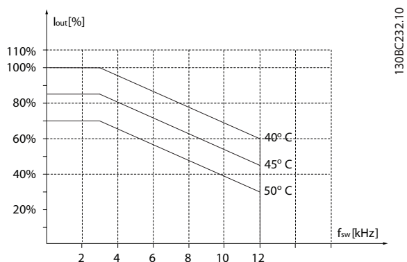
Illustration 3.37 55-75 kW (74-100 HP), 400 V, boîtier de taille H7, IP20
