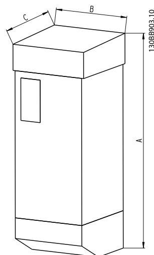
Illustration 4.7 Dimensions (voir données dans le Tableau 4.4)
