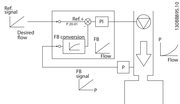
Illustration 3.20 Conversion du signal de retour
