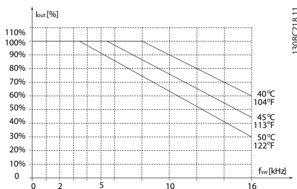
Illustration 3.23 0,37-1,5 kW (0,5-2,0 HP), 400 V, boîtier de taille H1, IP20
