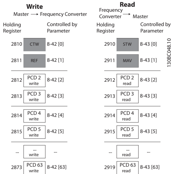
Illustration 7.14 Accès via écriture/lecture PCD
