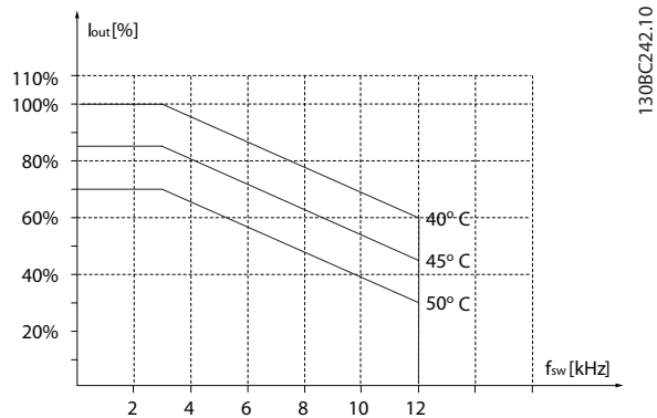
Illustration 3.50 45-55 kW (60-74 HP), 400 V, boîtier de taille I7, IP54
