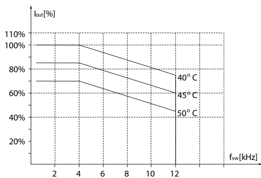
Illustration 3.32 15-18,5 kW (20-25 HP), 200 V, boîtier de taille H6, IP20
