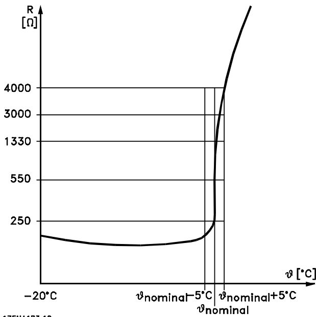
175HA183.10 Illustration 3.57 Arrêt dû à une haute température de moteur
