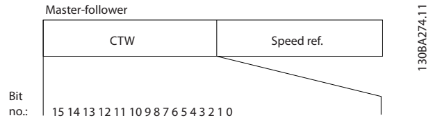
Illustration 7.15 Mot de contrôle selon le profil FC
