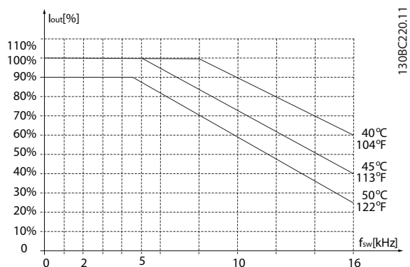
Illustration 3.25 2,2-4,0 kW (3,0-5,4 HP), 400 V, boîtier de taille H2, IP20
