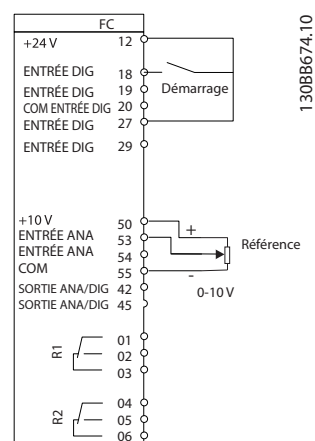
Illustration 6.2 Câblage du variateur de fréquence
