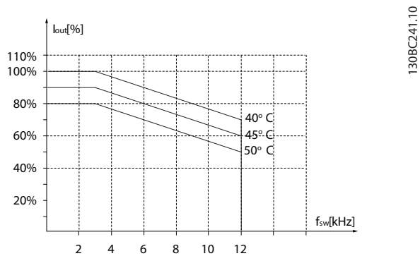
Illustration 3.49 37 kW (50 HP), 400 V, boîtier de taille I6, IP54
