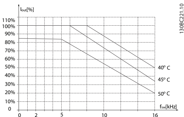
Illustration 3.26 3,7 kW (5,0 HP), 200 V, boîtier de taille H3, IP20
