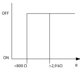
Illustration 3.58 Entrée digitale/alimentation 10 V
