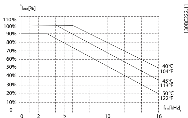
Illustration 3.27 5,5-7,5 kW (7,4-10 HP), 400 V, boîtier de taille H3, IP20
