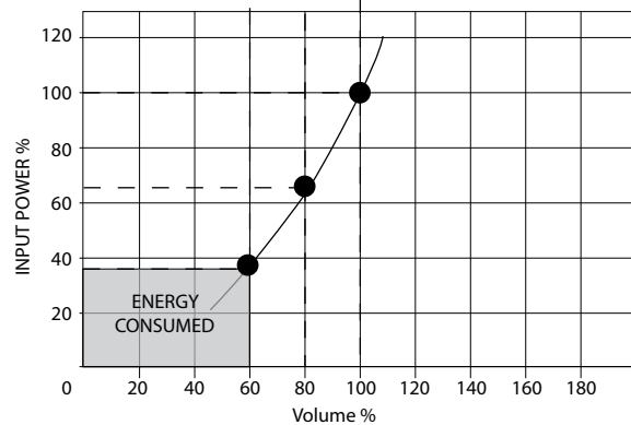
Illustration 3.2 Économies d'énergie réalisées grâce au variateur de fréquence
