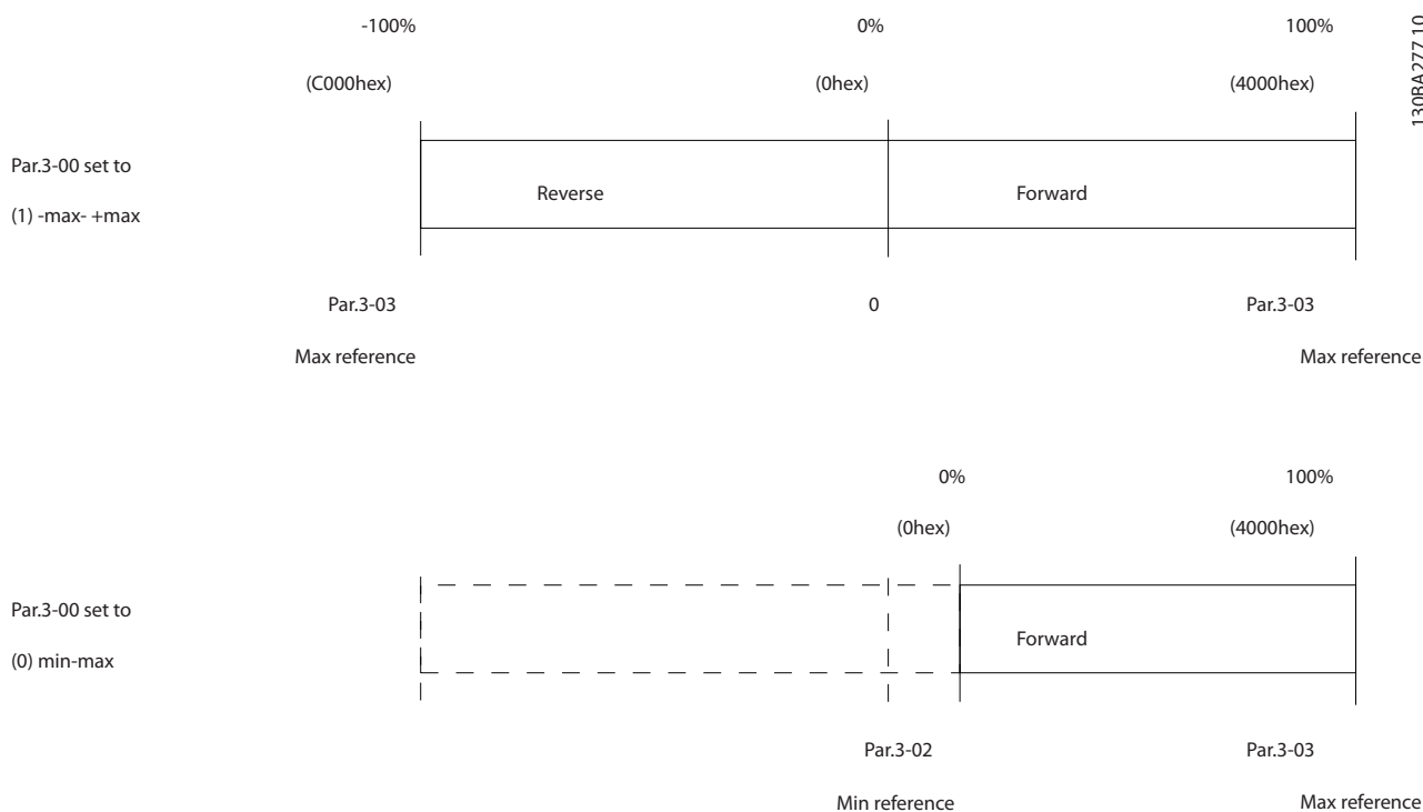
Illustration 7.18 Référence et MAV
