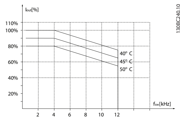
Illustration 3.48 22-30 kW (30-40 HP), 400 V, boîtier de taille I6, IP54
