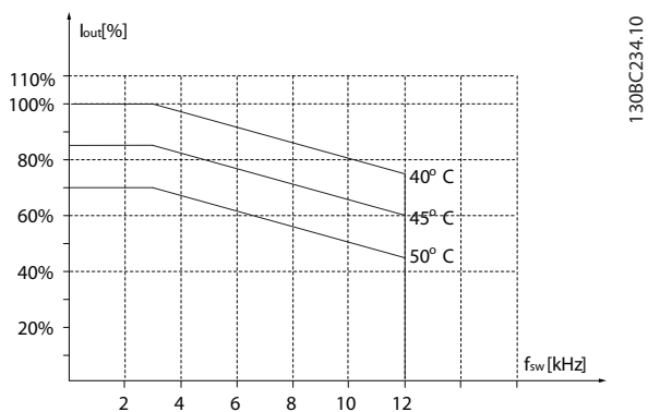
Illustration 3.39 37-45 kW (50-60 HP), 200 V, boîtier de taille H8, IP20
