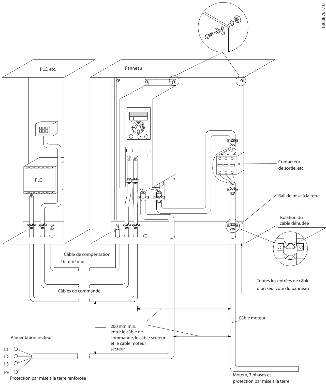
Illustration 5.16 Installation électrique conforme aux normes CEM
