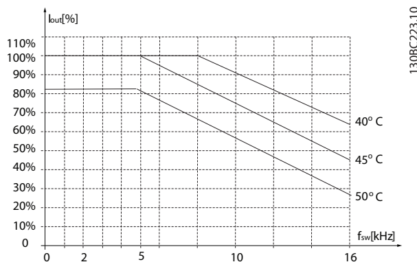
Illustration 3.28 5,5-7,5 kW (7,4-10 HP), 200 V, boîtier de taille H4, IP20
