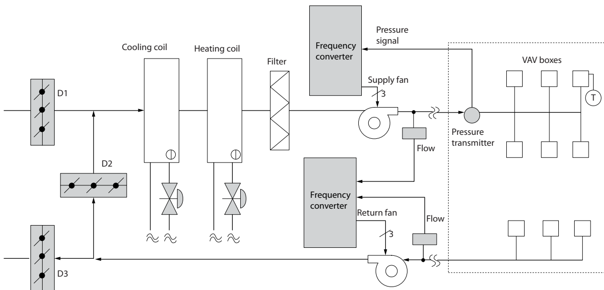
Illustration 3.11 Volume d'air variable
