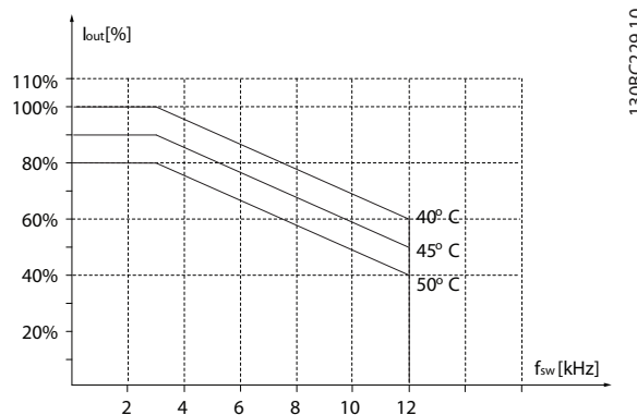
Illustration 3.34 45 kW (60 HP), 400 V, boîtier de taille H6, IP20
