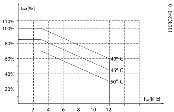
Illustration 3.51 75-90 kW (100-120 HP), 400 V, boîtier de taille I8, IP54
