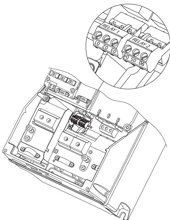
Illustration 5.14 Relais sur boîtiers de taille I6 IP54, 380-480 V, 22-37 kW (30-50 HP)
