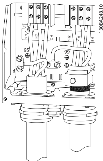
Illustration 5.15 Boîtiers de tailles I7, I8 IP54, 380-480 V, 45-55 kW (60-70 HP) IP54, 380-480 V, 75-90 kW (100-125 HP)
