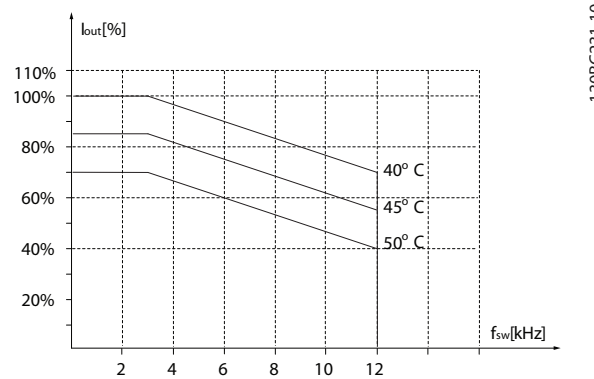
Illustration 3.36 22-30 kW (30-40 HP), 200 V, boîtier de taille H7, IP20
