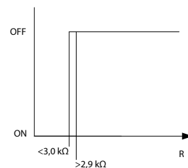
Illustration 3.59 Entrée analogique/alimentation 10 V
