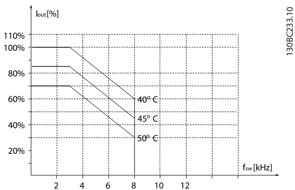
Illustration 3.38 45-55 kW (60-74 HP), 600 V, boîtier de taille H7, IP20
