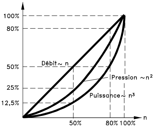
Illustration 3.3 Lois de proportionnalité
