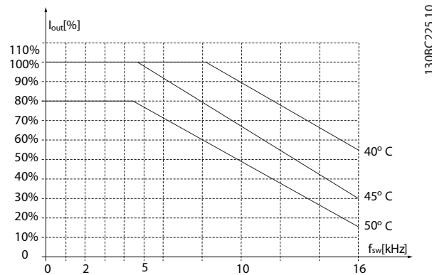
Illustration 3.30 11 kW (15 HP), 200 V, boîtier de taille H5, IP20
