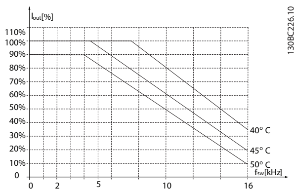
Illustration 3.31 18,5-22 kW (25-30 HP), 400 V, boîtier de taille H5, IP20
