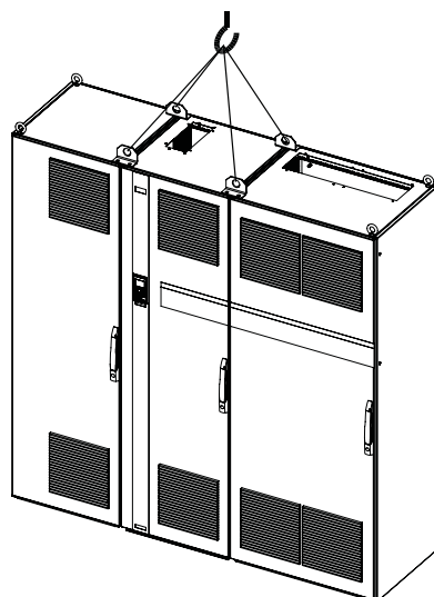
Abbildung 3.5: Empfohlenes Hebeverfahren, Baugröße F3
