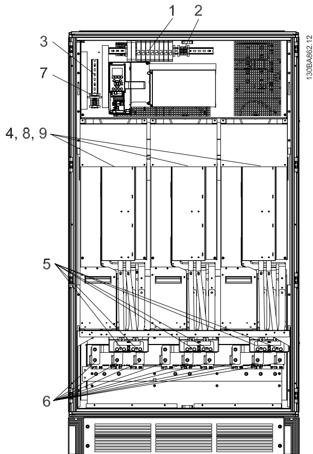
Abbildung 3.49: Wechselrichtergeräteeinheit, Baugröße F2 und F4
