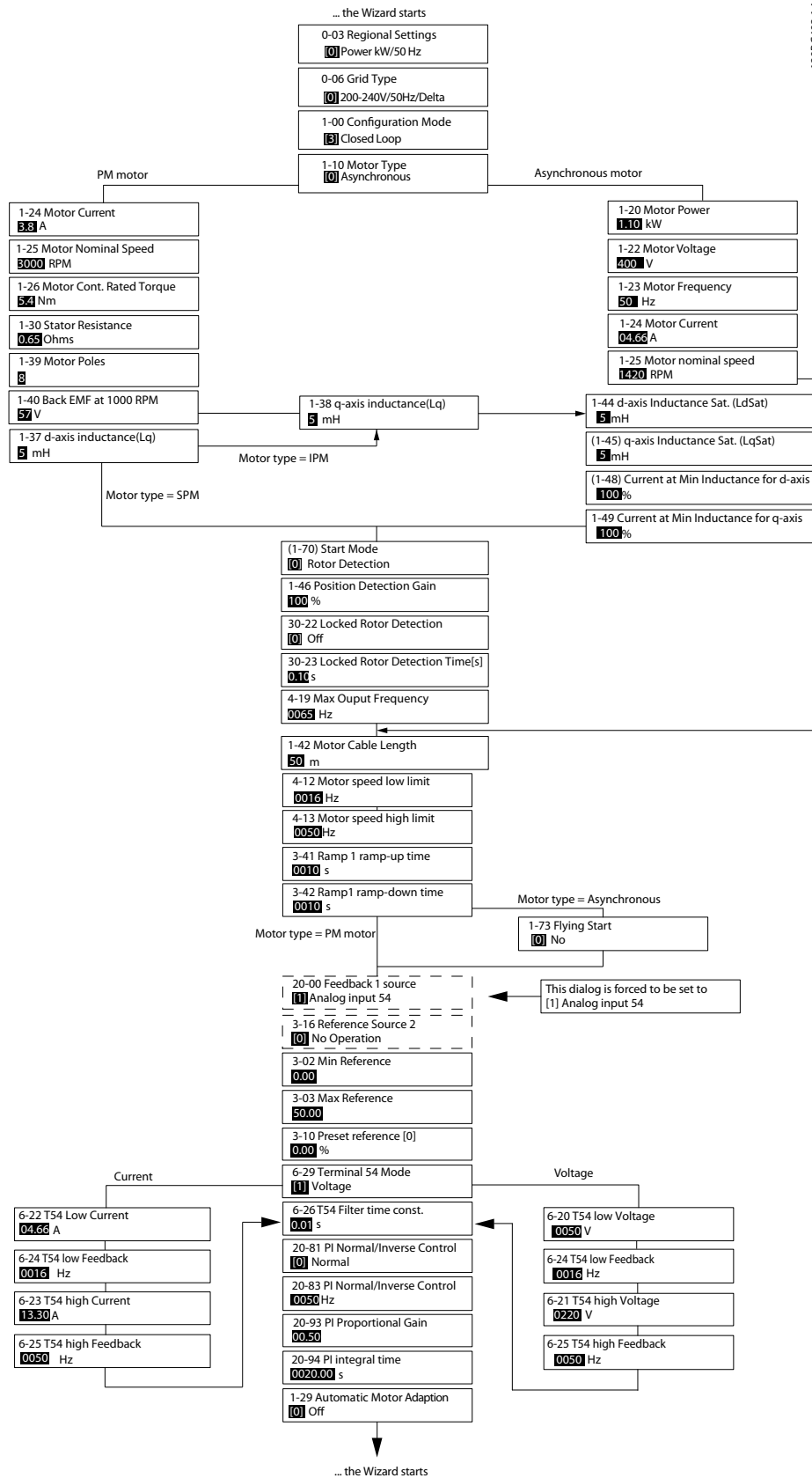
그림 6.5 폐회로 어플리케이션용 셋업 마법사
