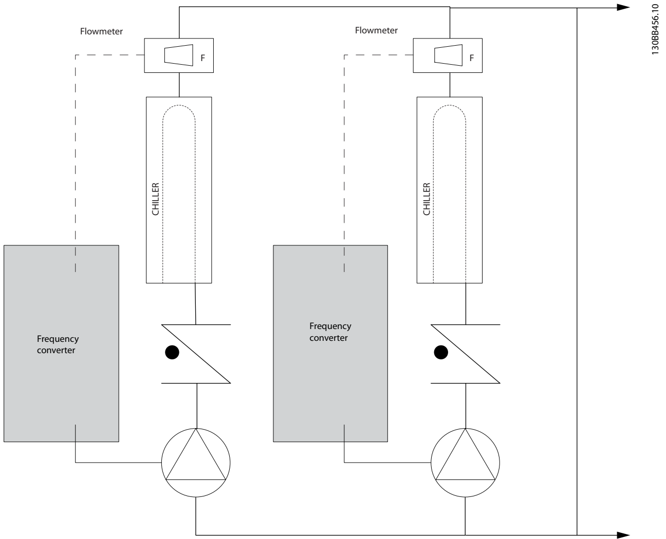
그림 3.15 1차 펌프
