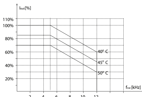
그림 3.42 2.2-3 kW (3.0-4.0 hp), 600 V, 외함 사이즈 H9, IP20
