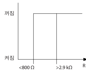
그림 3.58 디지털 입력/10 V 전원 공급
