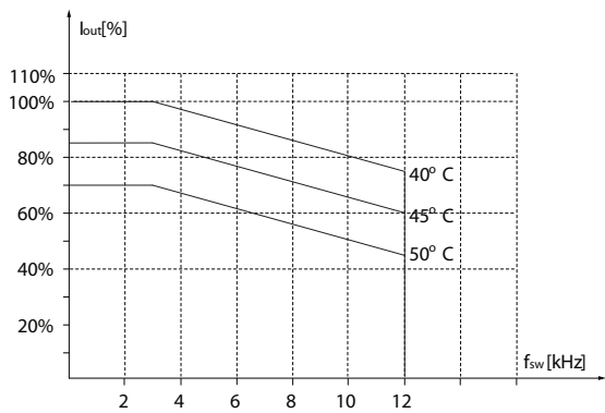
그림 3.39 37-45 kW (50-60 hp), 200 V, 외함 사이즈 H8, IP20
