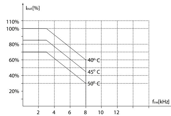
그림 3.41 75-90 kW (100-120 hp), 600 V, 외함 사이즈 H8, IP20
