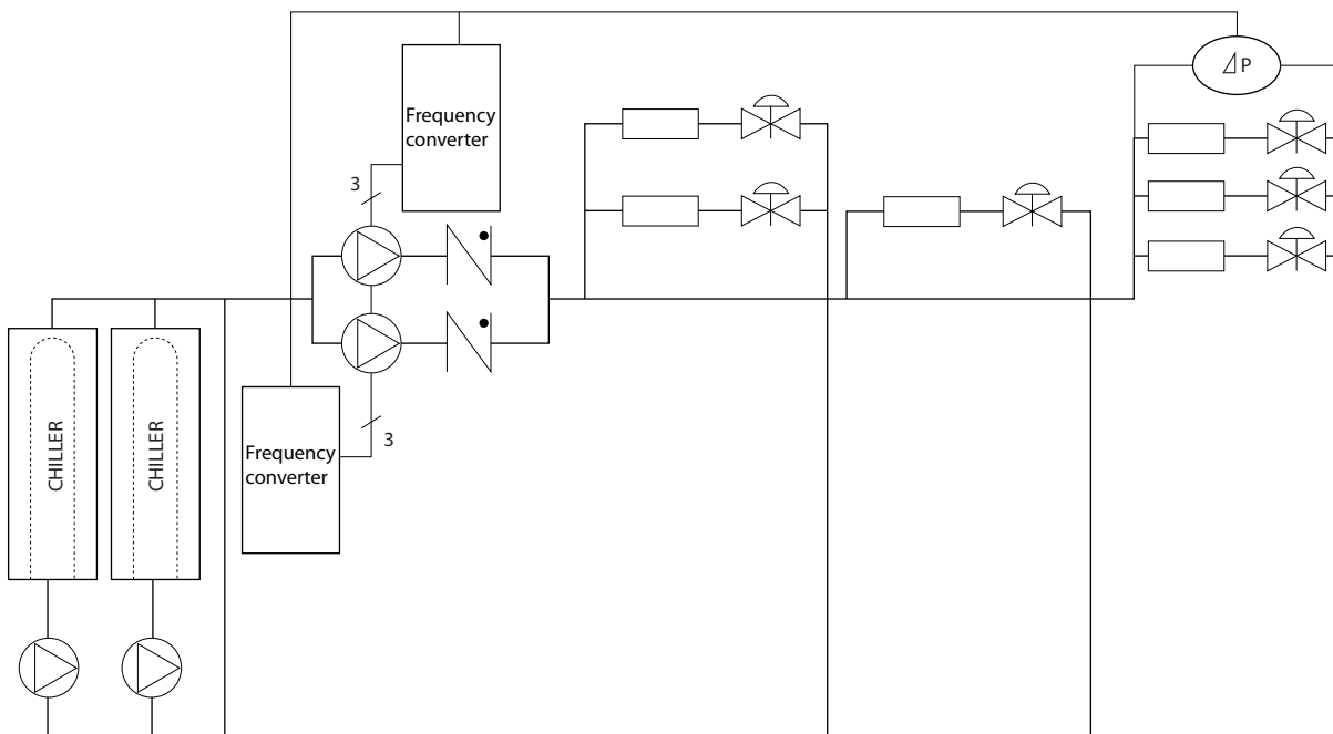
그림 3.16 2차 펌프
