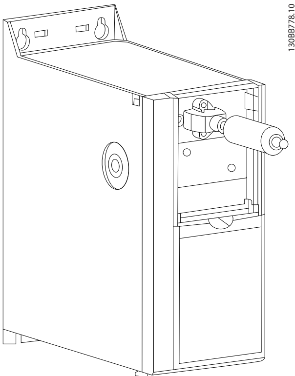
그림 4.5 케이블 연결
