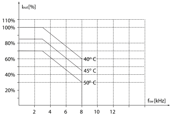
그림 3.38 45-55 kW (60-74 hp), 600 V, 외함 사이즈 H7, IP20
