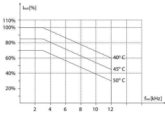
그림 3.37 55-75 kW (74-100 hp), 400 V, 외함 사이즈 H7, IP20
