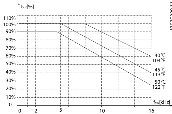
그림 3.25 2.2-4.0 kW (3.0-5.4 hp), 400 V, 외함 사이즈 H2, IP20
