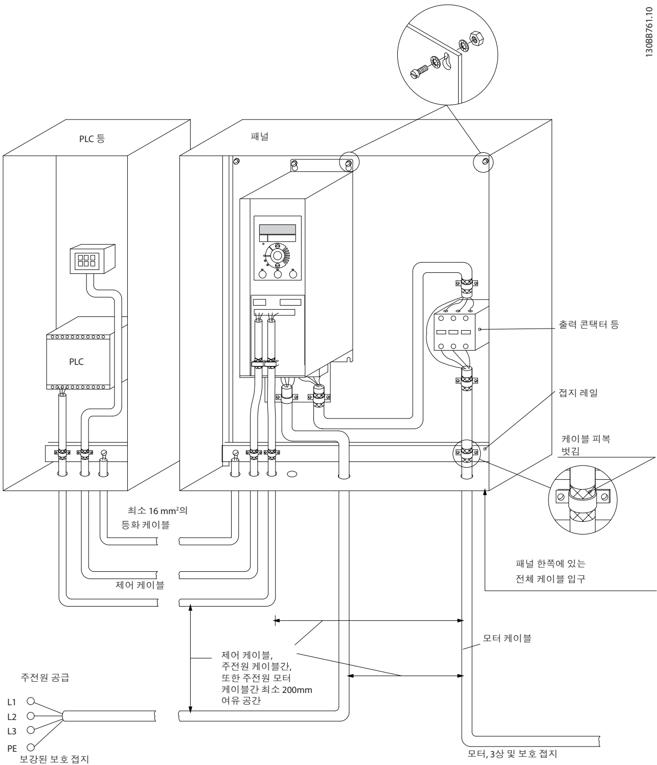
그림 5.16 EMC 규정에 따른 전기적인 설치
