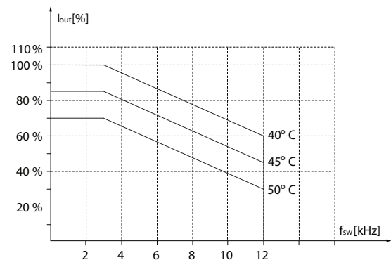
그림 3.40 90 kW (120 hp), 400 V, 외함 사이즈 H8, IP20
