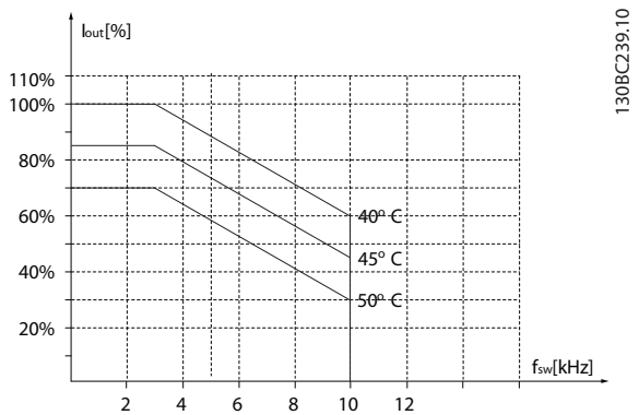
그림 3.44 11-15 kW (15-20 hp), 600 V, 외함 사이즈 H10, IP20
