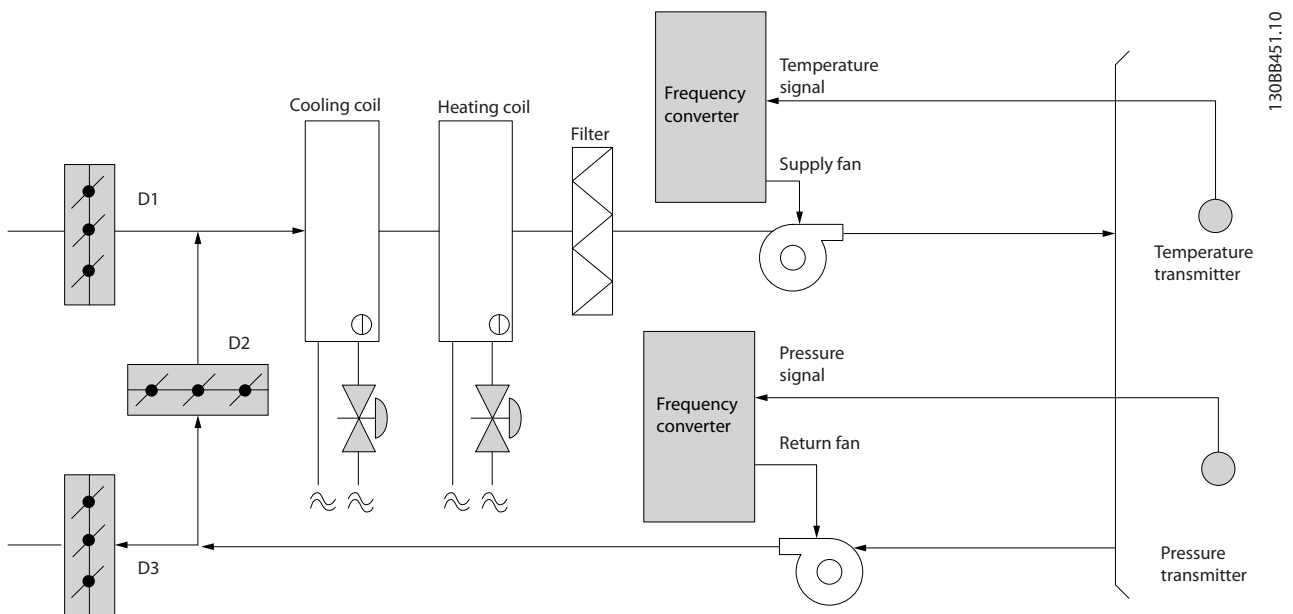
그림 3.12 일정 공기량
