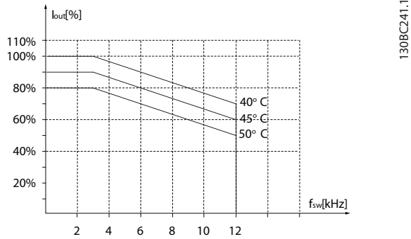
Afbeelding 3.49 37 kW (50 pk), 400 V, behuizingsgrootte 16, IP 54
