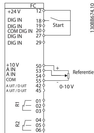
Afbeelding 6.2 Bedrading frequentieregelaar
