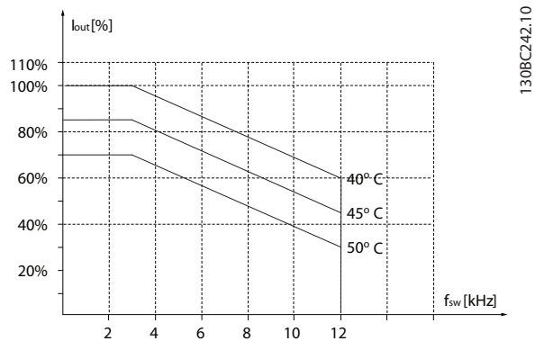
Afbeelding 3.50 45-55 kW (60-74 pk), 400 V, behuizingsgrootte 17, IP 54
