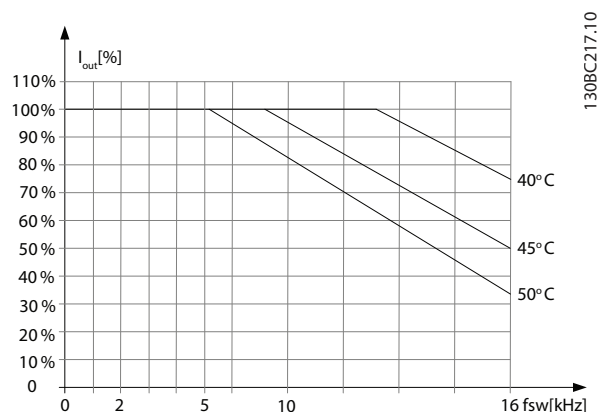
Afbeelding 3.22 0,25-0,75 kW (0,34-1,0 pk), 200 V, behuizingsgrootte H1, IP 20
