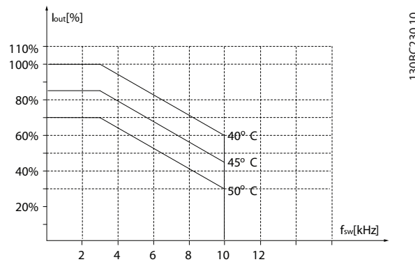
Afbeelding 3.35 22-30 kW (30-40 pk), 600 V, behuizingsgrootte H6, IP 20
