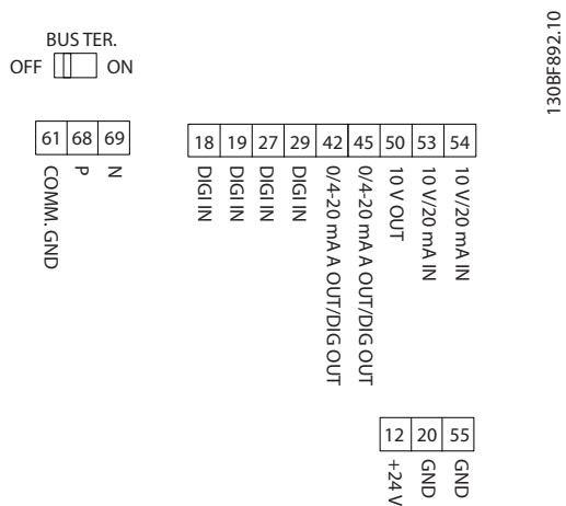
Afbeelding 5.17 Stuurklemmen
