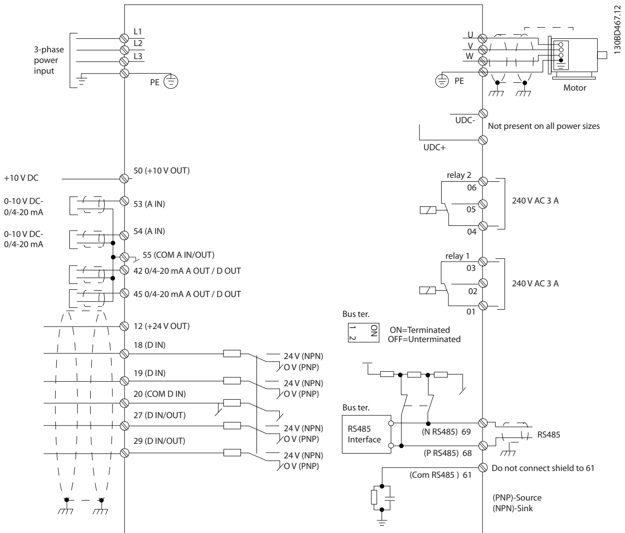
Afbeelding 5.1 Eenvoudig bedradingschema
