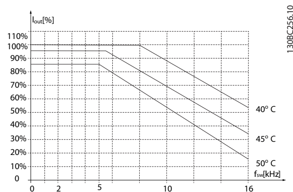
Afbeelding 3.46 5,5-7,5 kW (7,4-10 pk), 400 V, behuizingsgrootte I3, IP 54
