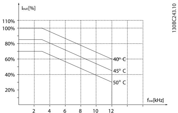
Afbeelding 3.51 75-90 kW (100-120 pk), 400 V, behuizingsgrootte 18, IP 54
