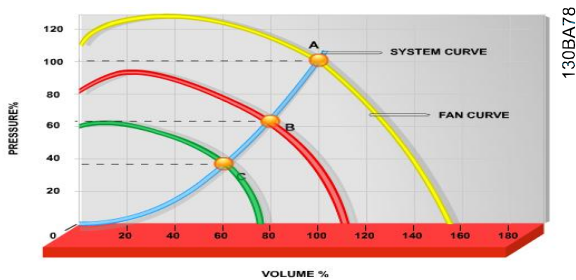
Afbeelding 3.1 Ventilatorcurves (A, B en C) voor gereduceerde ventilatorvolumes
