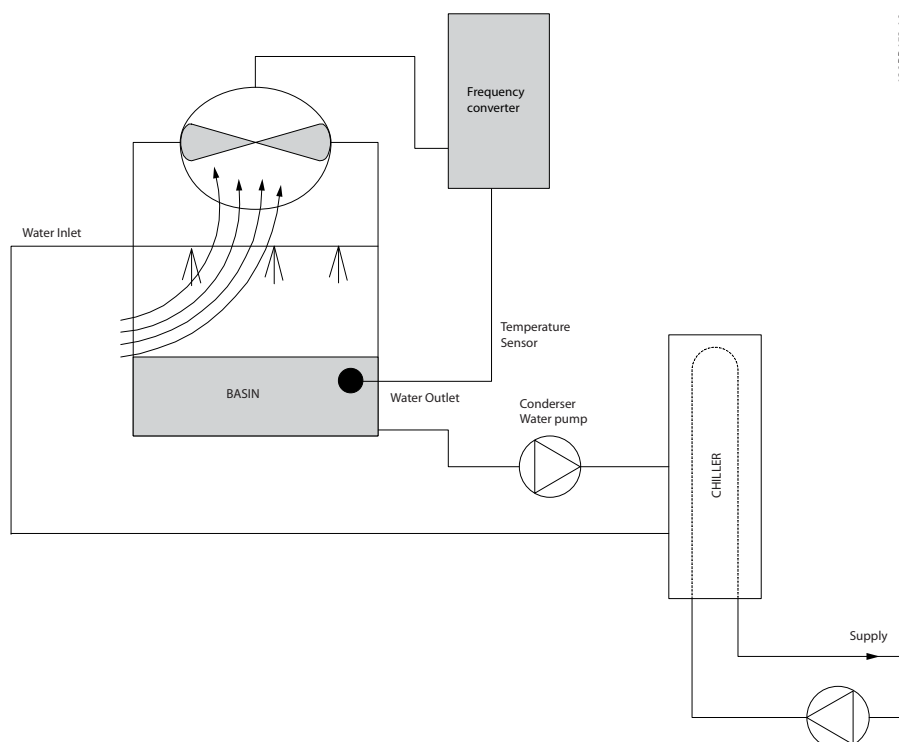
Afbeelding 3.13 Koeltorenventilator
