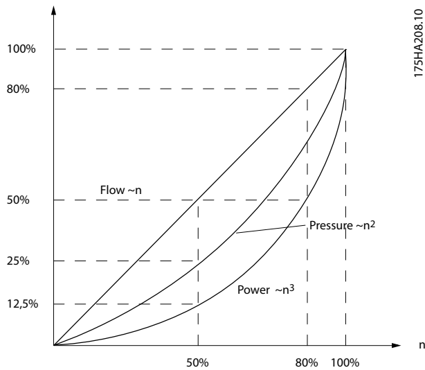
Afbeelding 3.3 Proportionaliteitswetten
