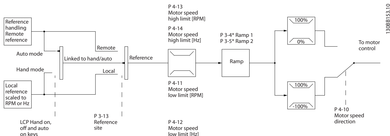
Afbeelding 2.11 Blokschema voor een regeling zonder terugkoppeling
