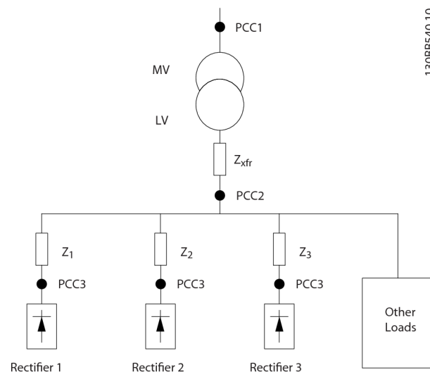
Afbeelding 3.4 Klein distributiesysteem
