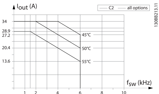
Afbeelding 5.21 Reductie van de uitgangsstroom wegens schakelfrequentie en omgevingstemperatuur voor behuizingsgrootte C2, 60° AVM
