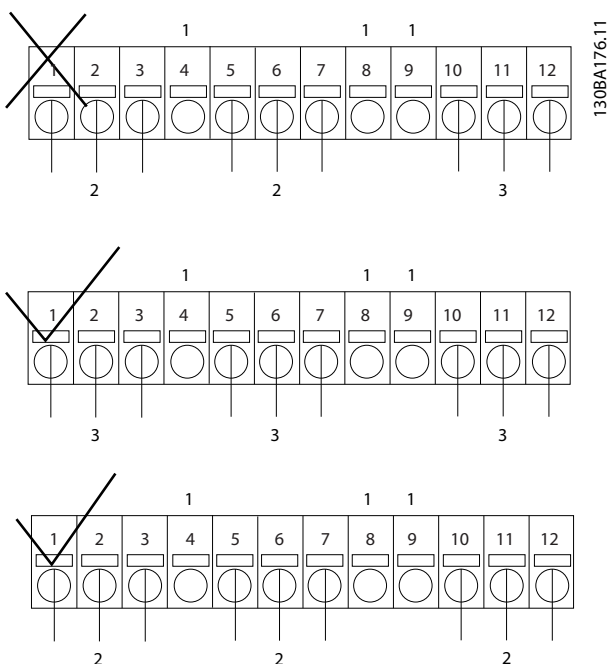
Afbeelding 7.9 MCB 112 installeren
