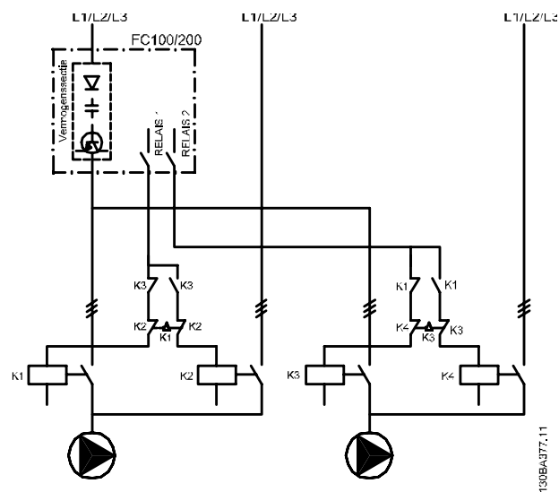
Afbeelding 4.13 Bedradingsschema voor hoofdpompwisseling
