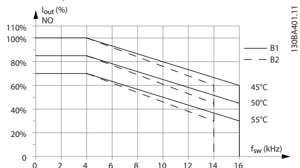
Afbeelding 5.7 Reductie van I_{out} voor diverse T_{AMB, MAX} voor behuizingsgrootte B1 en B2, bij gebruik van 60° AVM en een normale overbelastingsmodus (overbelastingskoppel van 110%)
