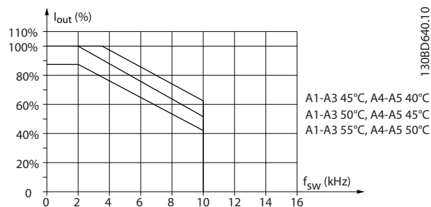
Afbeelding 5.6 Reductie van I_{out} voor diverse T_{AMB, MAX} voor behuizingsgrootte A, bij gebruik van SFAVM en een motorkabel van maximaal 10 m
