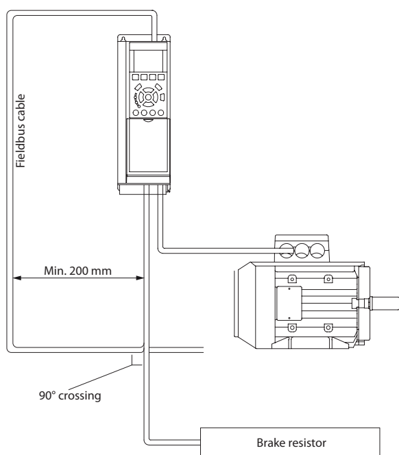
Afbeelding 3.43 Bekabeling
