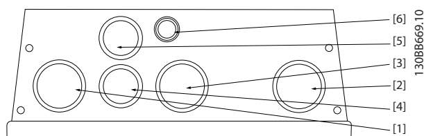
Afbeelding 8.28 Behuizingsgrootte B1, IP 55
