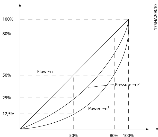
Afbeelding 2.2 Affiniteitswetten voor centrifugaalpomp
