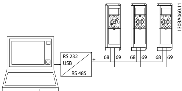
Afbeelding 3.41 Parallelle aansluitingen
