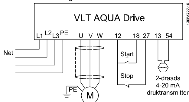
Afbeelding 4.7 Bedrading voor toepassing met pomp
