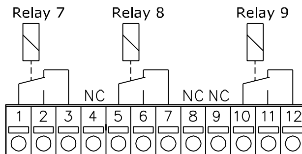
Afbeelding 7.6 Relais
