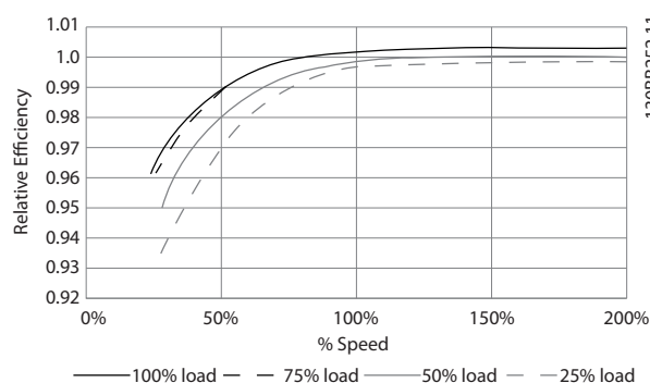
Afbeelding 3.19 Typische rendementscurves
