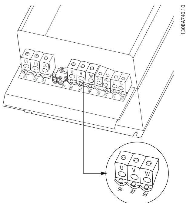
Afbeelding 8.17 Motoraansluiting voor behuizing C3 en C4
