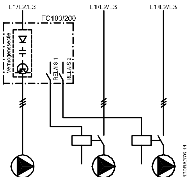
Afbeelding 4.12 Bedradingsschema voor pomp met variabel toerental
