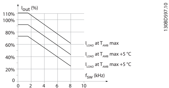
Afbeelding 5.23 Reductie van de uitgangsstroom wegens schakelfrequentie en omgevingstemperatuur voor behuizingsgrootte C3
