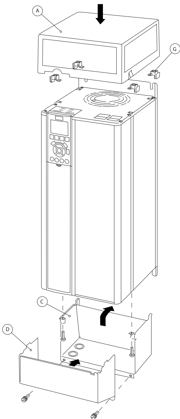
Afbeelding 3.34 Behuizingsgrootte B4, C3 en C4
