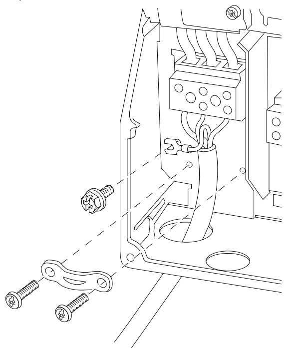
Afbeelding 8.4 Netvoeding voor behuizing B1 en B2
