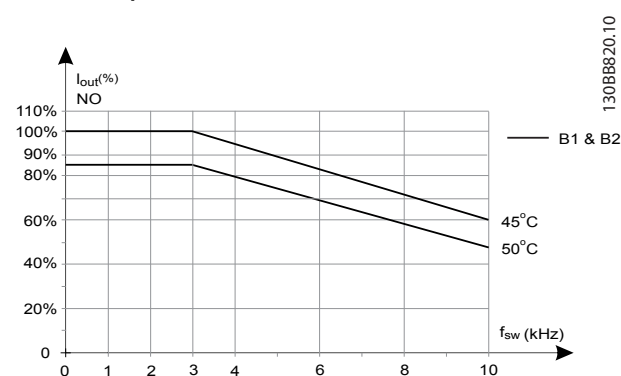
Afbeelding 5.11 Reductie van de uitgangsstroom wegens schakelfrequentie en omgevingstemperatuur voor 600 V-frequentieomvormers, behuizingsgrootte B, 60° AVM, NO
