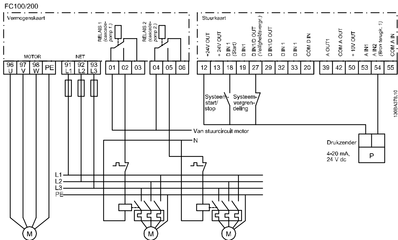
Afbeelding 4.11 Bedradingsschema cascaderelelaar
