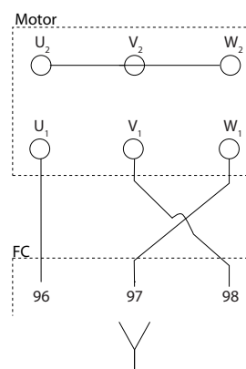
Afbeelding 3.10 Klemaansluiting voor rechtsom en linksom draaien
