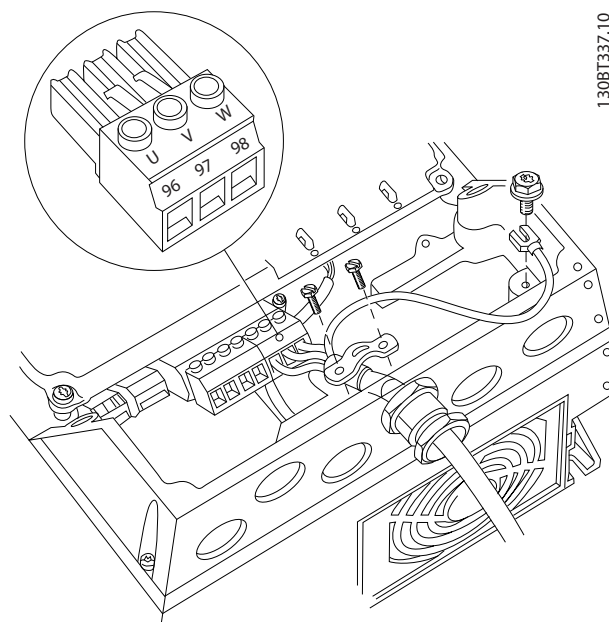
Afbeelding 8.12 Motoraansluiting voor behuizing A4/A5
