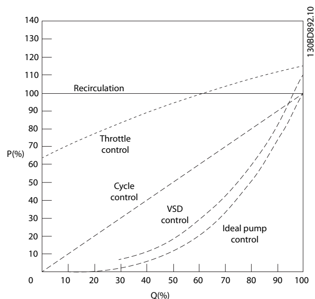
Afbeelding 2.5 Vergelijkende debietregelingscurves
