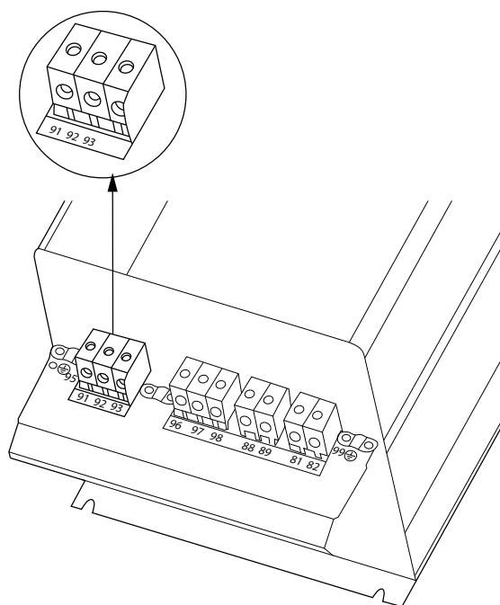
Afbeelding 8.8 Netvoeding voor behuizing C3 (IP 20)
