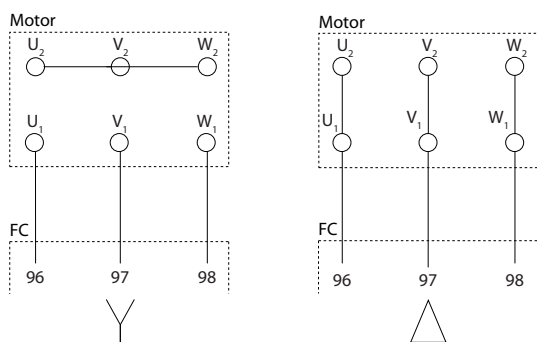
Afbeelding 8.10 Ster- en driehoekschakelingen
