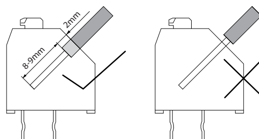
Afbeelding 7.7 Juiste kabeldoorvoer
