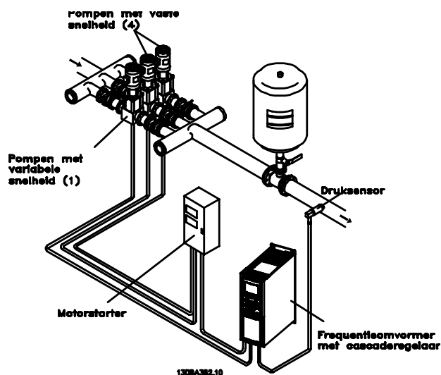
Afbeelding 4.9 BASIC cascaderelgelaar
