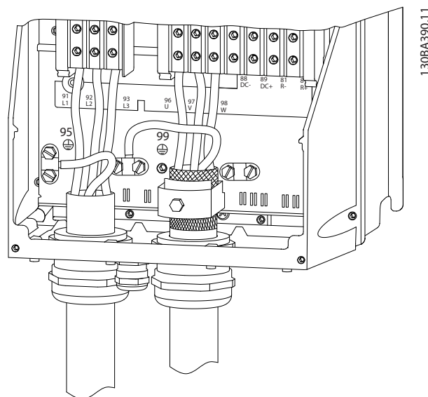
Afbeelding 8.16 Motoraansluiting voor behuizing C1 en C2 (IP 21/NEMA type 1 en IP 55/66/NEMA type 12)
