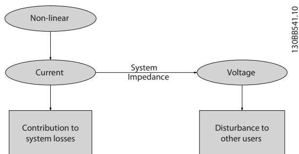
Afbeelding 3.5 Negatieve effecten van harmonischen
