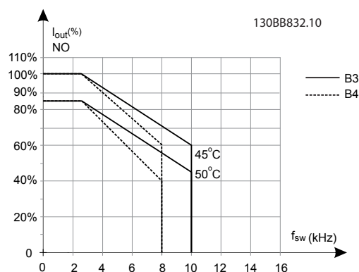
Afbeelding 5.10 Reductie van I_{out} voor diverse T_{AMB, MAX} voor behuizingsgrootte B3 en B4, bij gebruik van SFAVM en een normale overbelastingsmodus (overbelastingskoppel van 110%)
