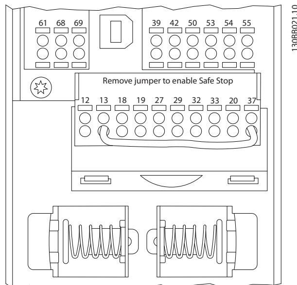
Afbeelding 3.42 Stuurkaartklemmen
