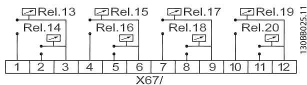
Afbeelding 7.19 Klemaansluitingen Advanced Cascade Controller MCO 102, 8 relais
