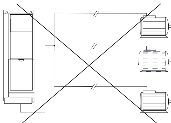
Afbeelding 3.12 Gemeenschappelijk koppelpunt voor lange kabellengtes
