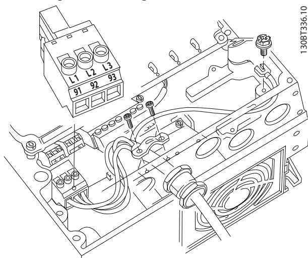
Afbeelding 8.2 Netvoeding en aarding zonder netschakelaar
