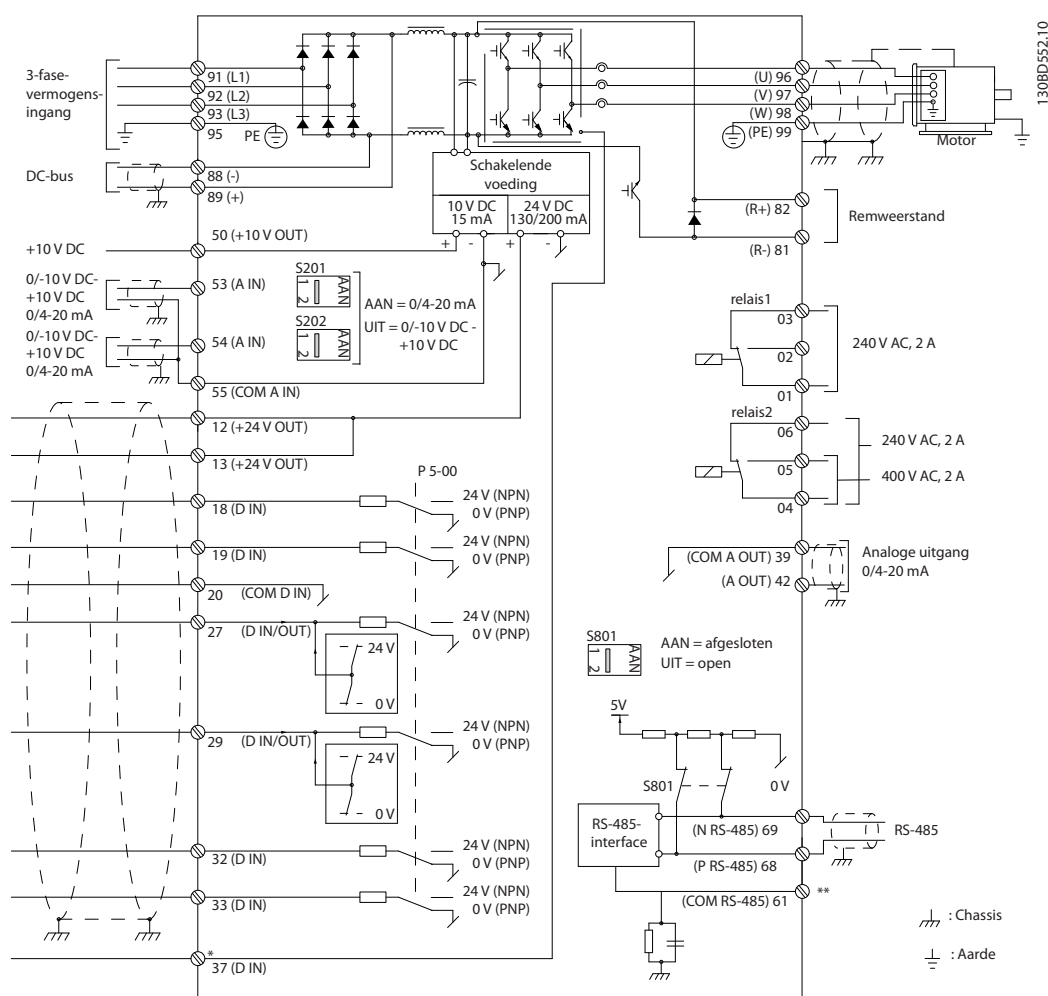
Afbeelding 3.20 Eenvoudig bedradingsschema
